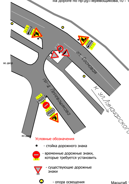
Схема размещения средств регулирования на северном пересечении пр-да Перовщикова и ул.Сосновой при производстве работ на дороге по пр-ду Перовщикова, 10 - 1 этап
