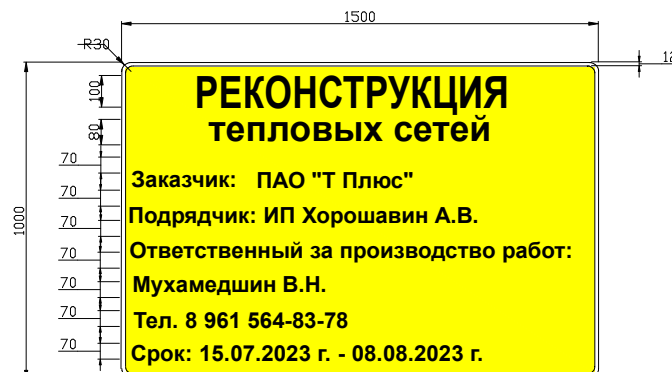
ЭСКИЗНЫЙ ПРОЕКТ ИНФОРМАЦИОННОГО ЩИТА
