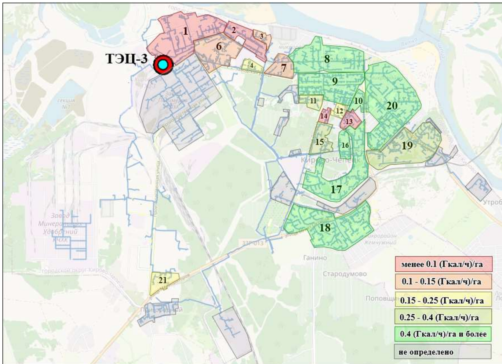
Рисунок 1 – Плотность нагрузок в существующей зоне действия ТЭЦ-3
