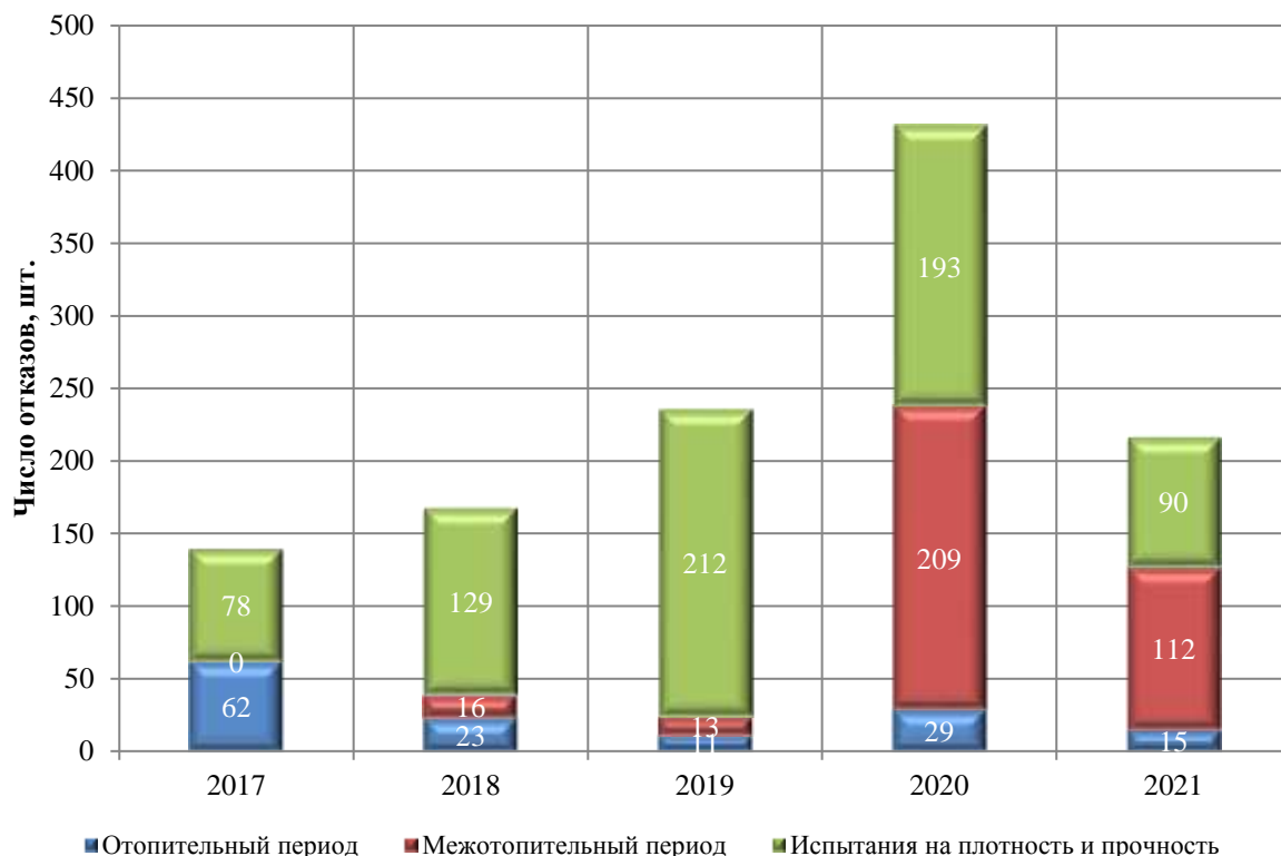
Рисунок 1 – Соотношение числа отказов
