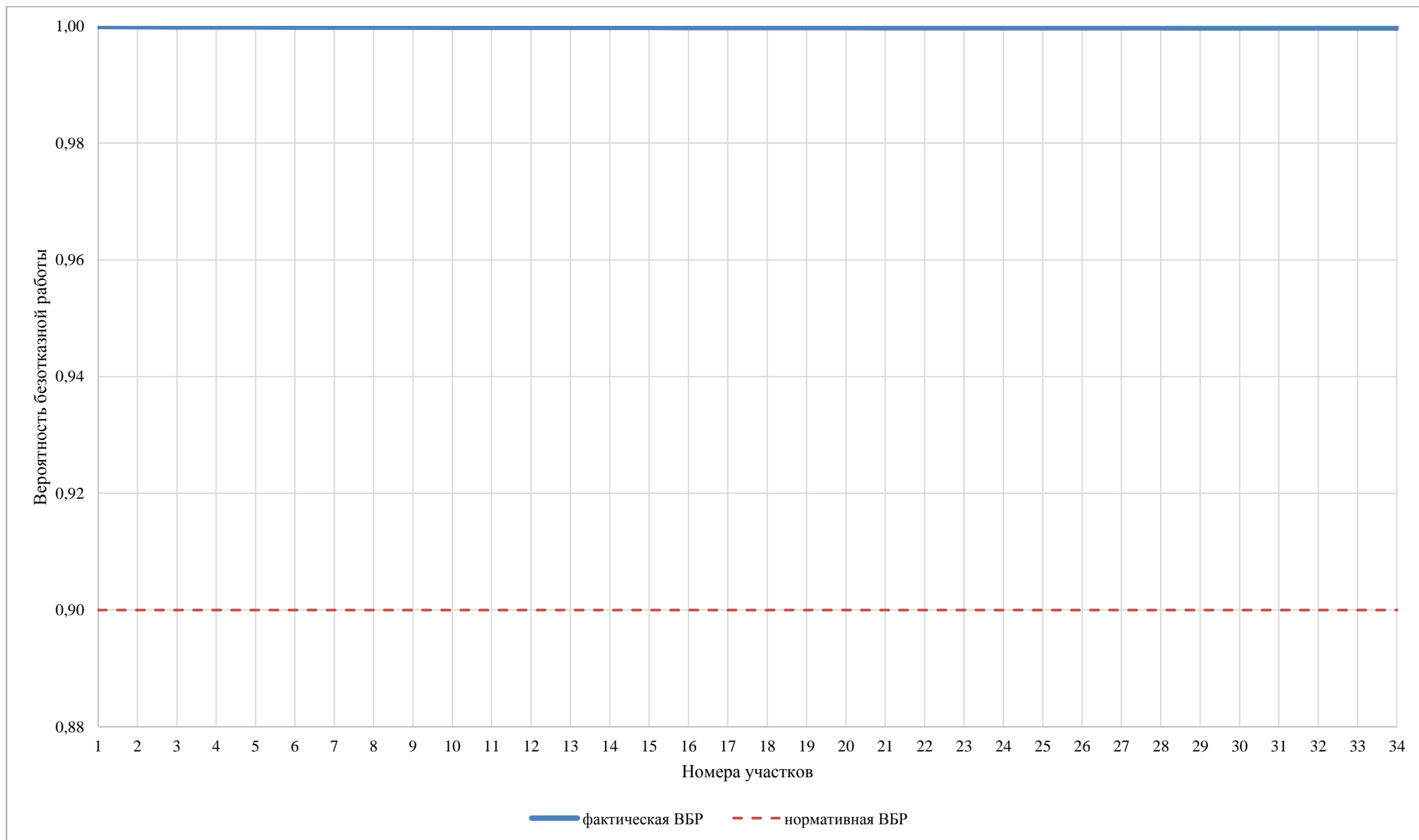
Рисунок 16 – Сравнительный анализ нормативной и фактической ВБР по пути движения теплоносителя, в зоне действия котельной Каринторф (рисунок П46.2 МУ)
