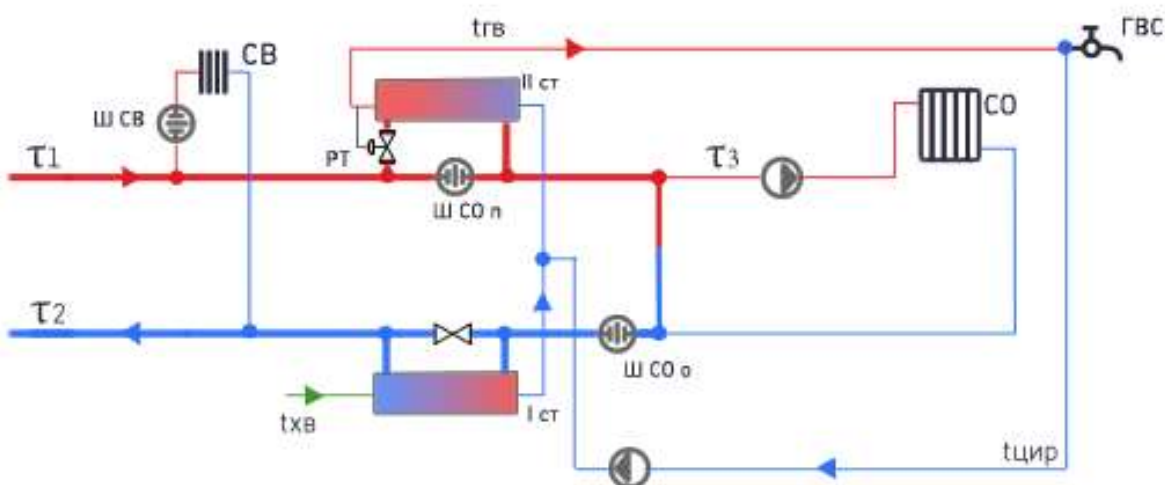
Рисунок 25 – Схема с двухступенчатым последовательным подключением подогревателей ГВС и насосным присоединением СО (насос на подающем трубопроводе)
