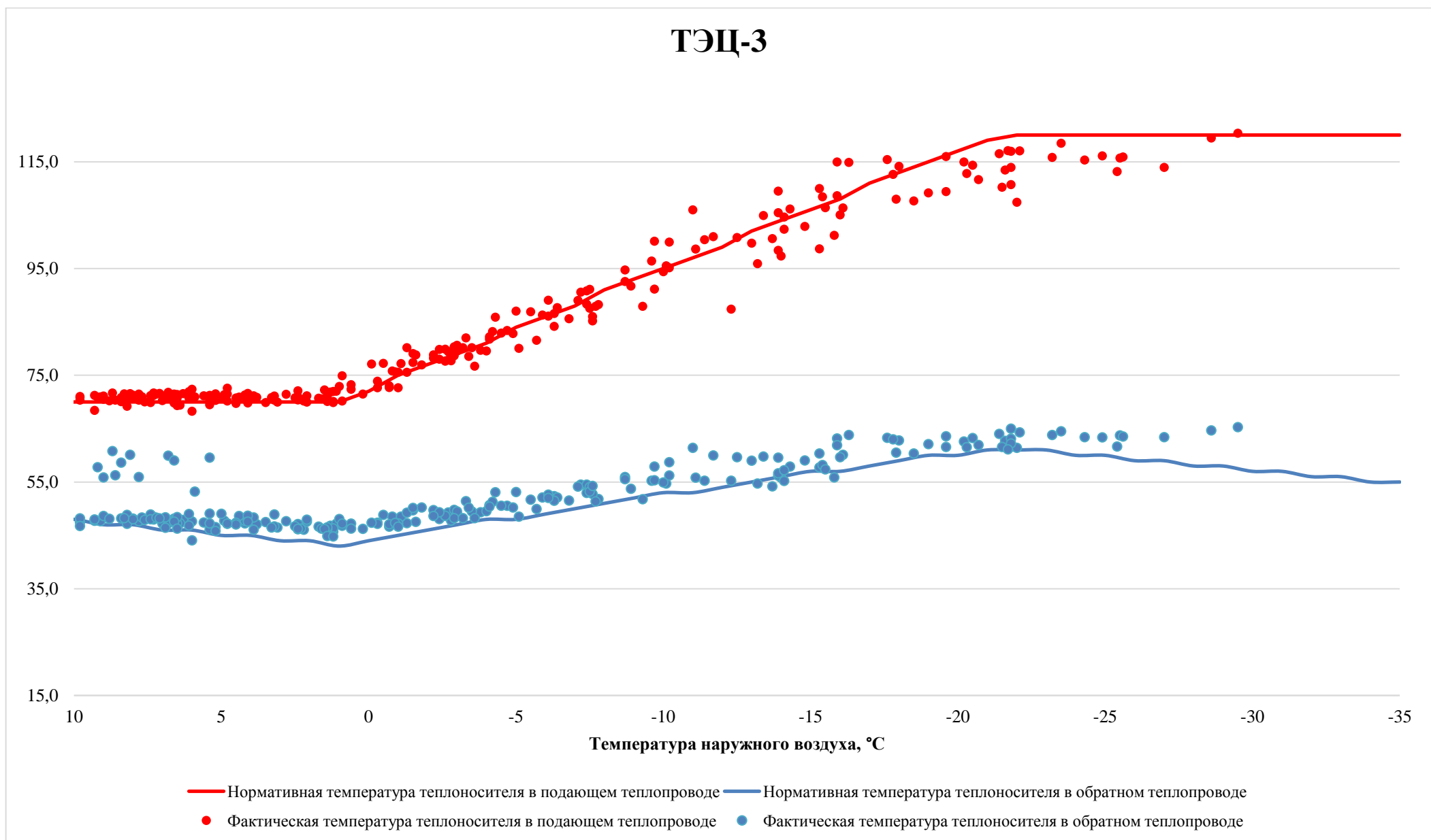
Рисунок 9 – Сравнение фактического графика изменения температуры теплоносителя от ТЭЦ-3 за 2021 г. и расчетного температурного графика
