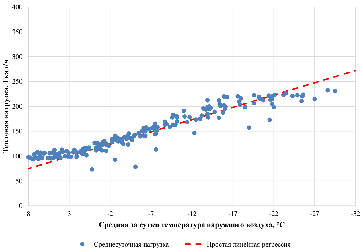
Рисунок 33 – Определение расчетной тепловой нагрузки на коллекторах, в зоне действия ТЭЦ-3
