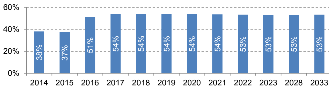
Рис. 2.1.5. Коэффициент использования установленной тепловой мощности Кировской ТЭЦ-3
