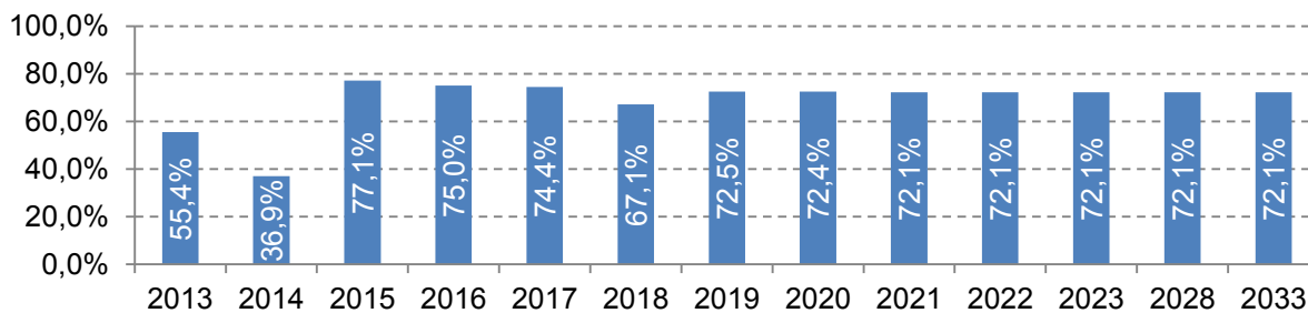
Рис. 2.1.6. Коэффициент использования установленной электрической мощности Кировской ТЭЦ-3
