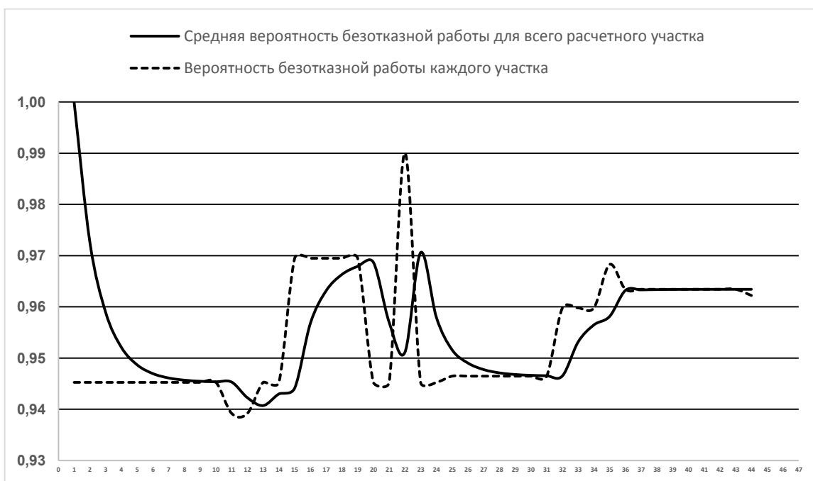
Рис. 9.1.3. Вероятность безаварийной работы тепловой магистрали от Кировской ТЭЦ-3 до ТК 10-16 в 2018 г. основная.
