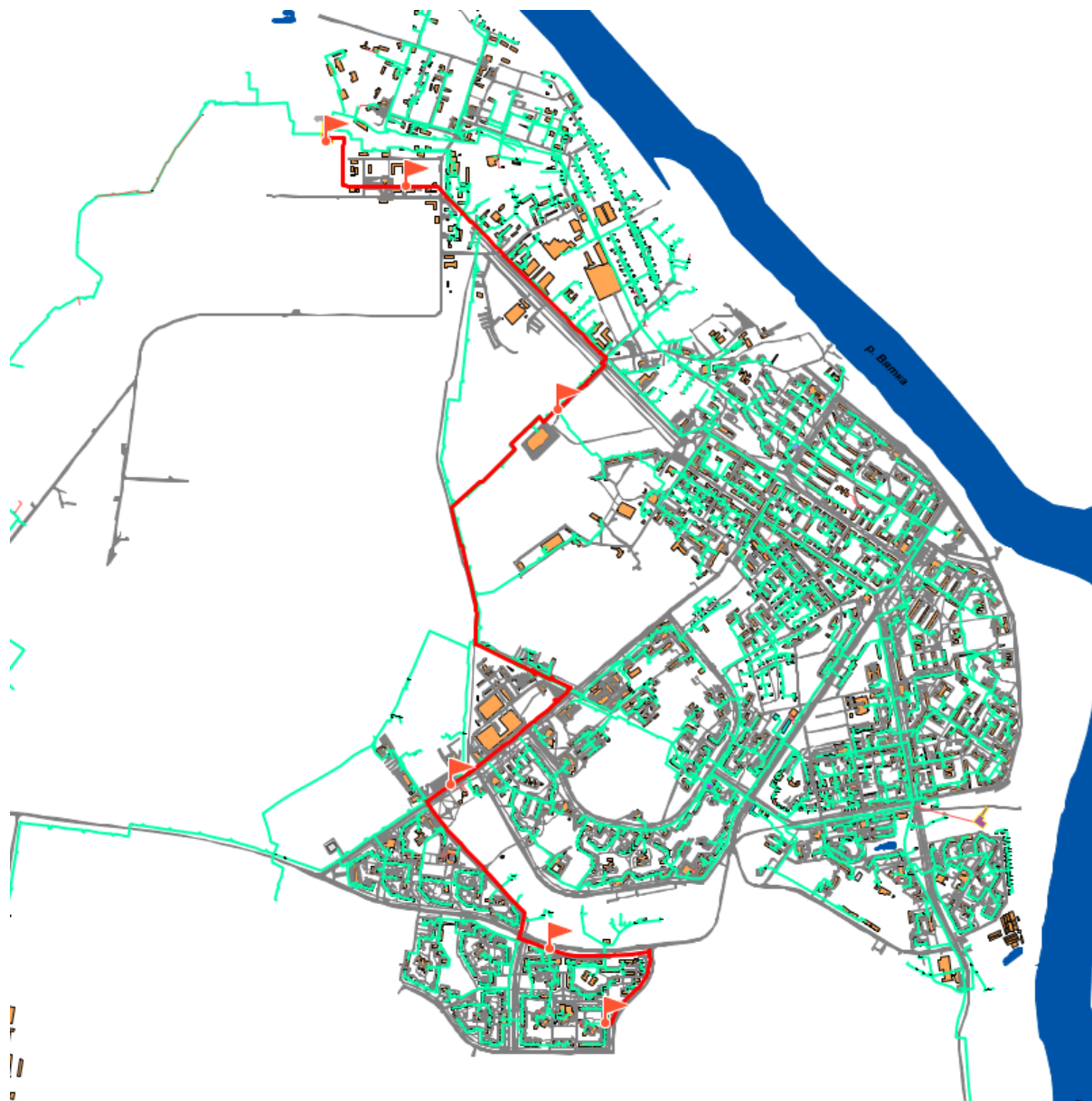
Рис. 9.1.2. Резервный участок тепловой сети от Кировской ТЭЦ-3 до ТК 10-16
