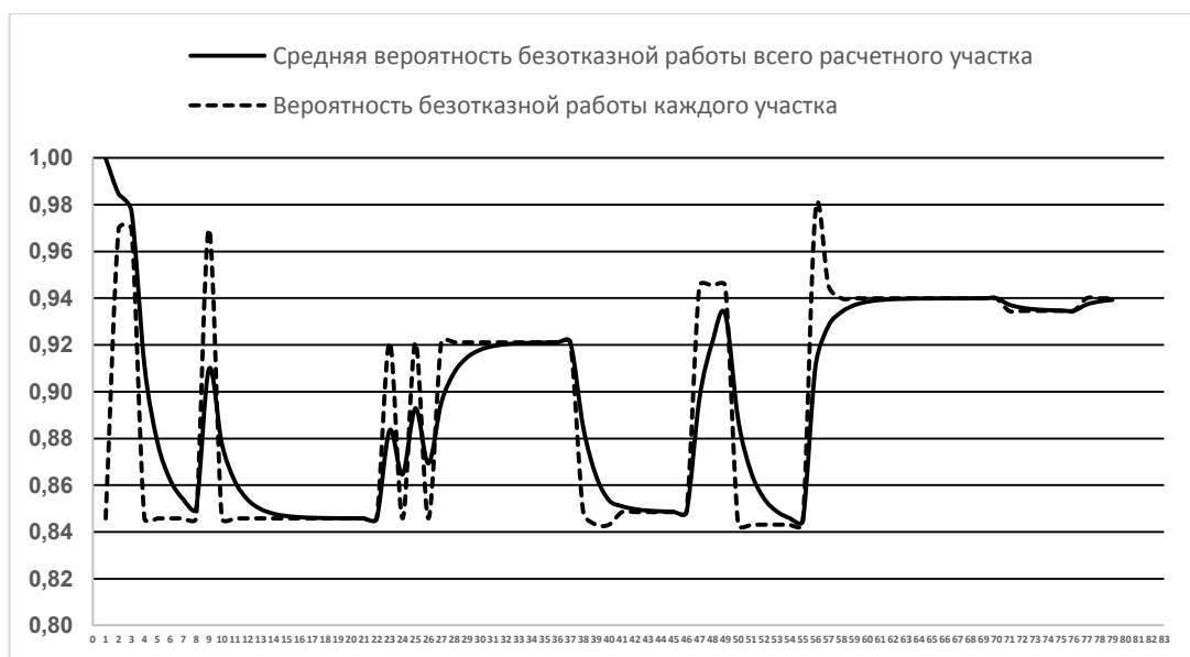
Рис. 9.1.13 Вероятность безаварийной работы тепломатриале от ТЭЦ-3 до 5-12 основная
