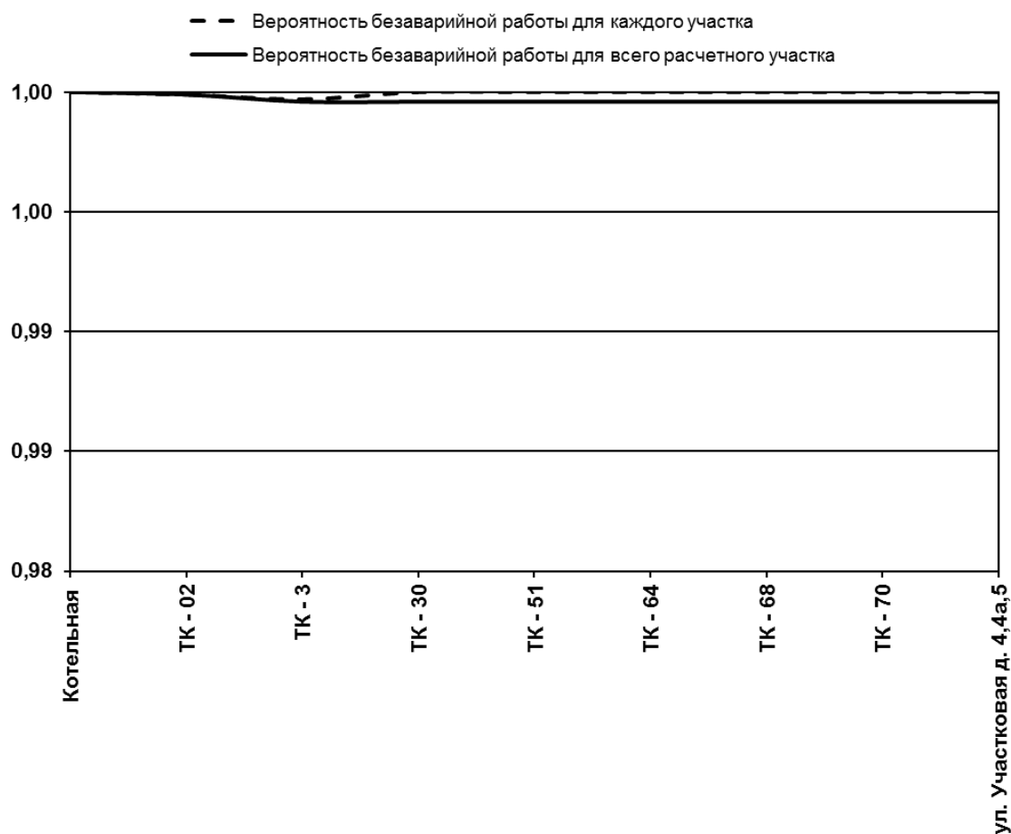
Рис. 9.2.2. Вероятность безаварийной работы тепловой магистрали от котельной Каринторф до ул. Участковая д.4, 4а, 5
