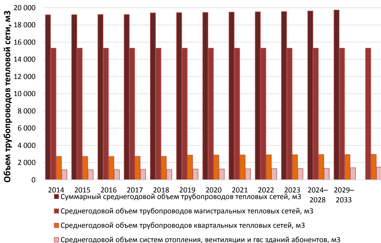
Рис. 7.2.1. Фактические и перспективные объемы тепловых сетей г. Кирово-Чепецка на период 2014 – 2033 гг.
