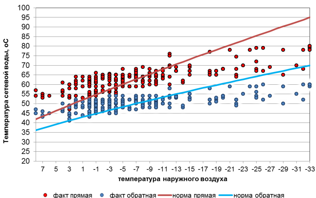
Рис. 3.2.3. Сравнение фактической температуры сетевой воды в подающих и обратных трубопроводах с температурным графиком отпуска тепловой энергии в тепловые сети от котельной микрорайона Каринторф
