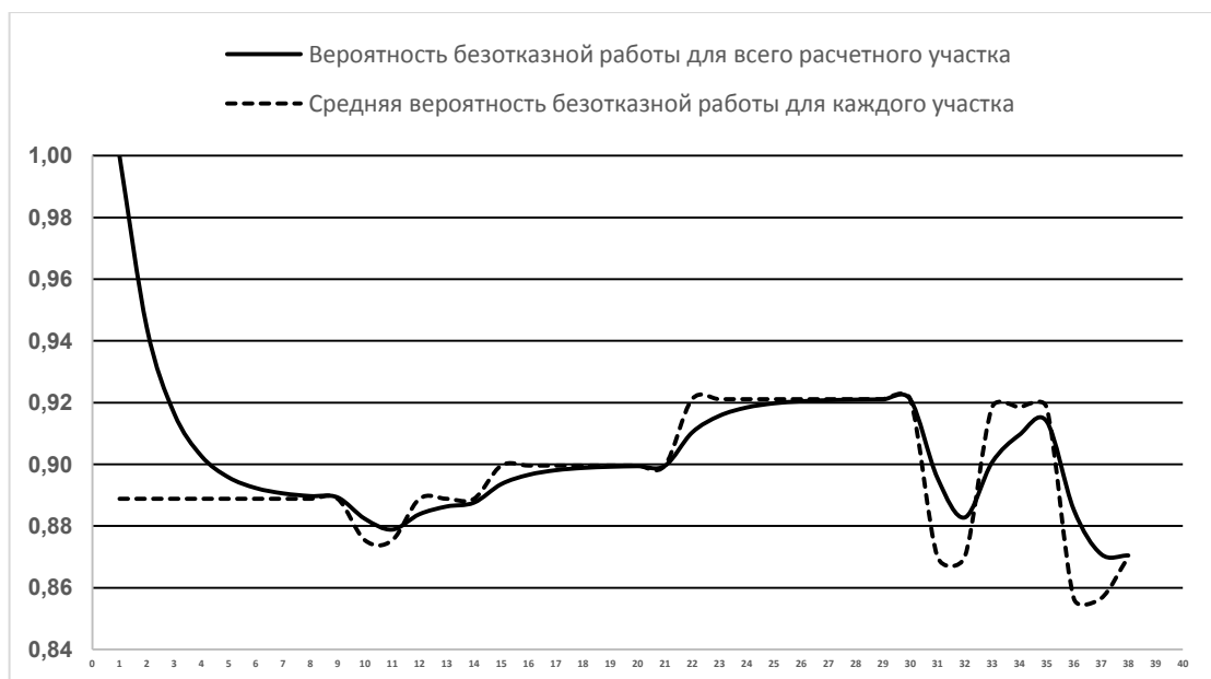
Рис. 9.1.8. Вероятность безаварийной работы тепловой магистрали от ТЭЦ-3 до Уз 3-47 резерв
