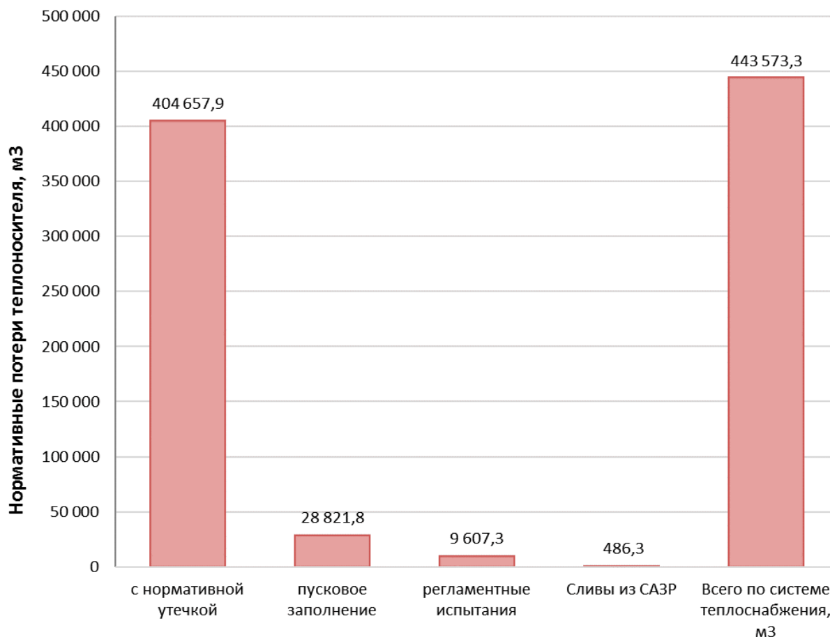
Рис. 7.1.1. Расчетные значения потерь теплоносителя с нормативной утечкой, на пусковое заполнение, на регламентные испытания для магистральных, квартальных тепловых сетей, потребителей и суммарно по системе теплоснабжения
