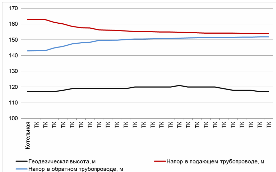
Рис. 6.2.2. Пьезометрический график работы тепловой сети от котельной мкр. Каринторф в 2018 г.
