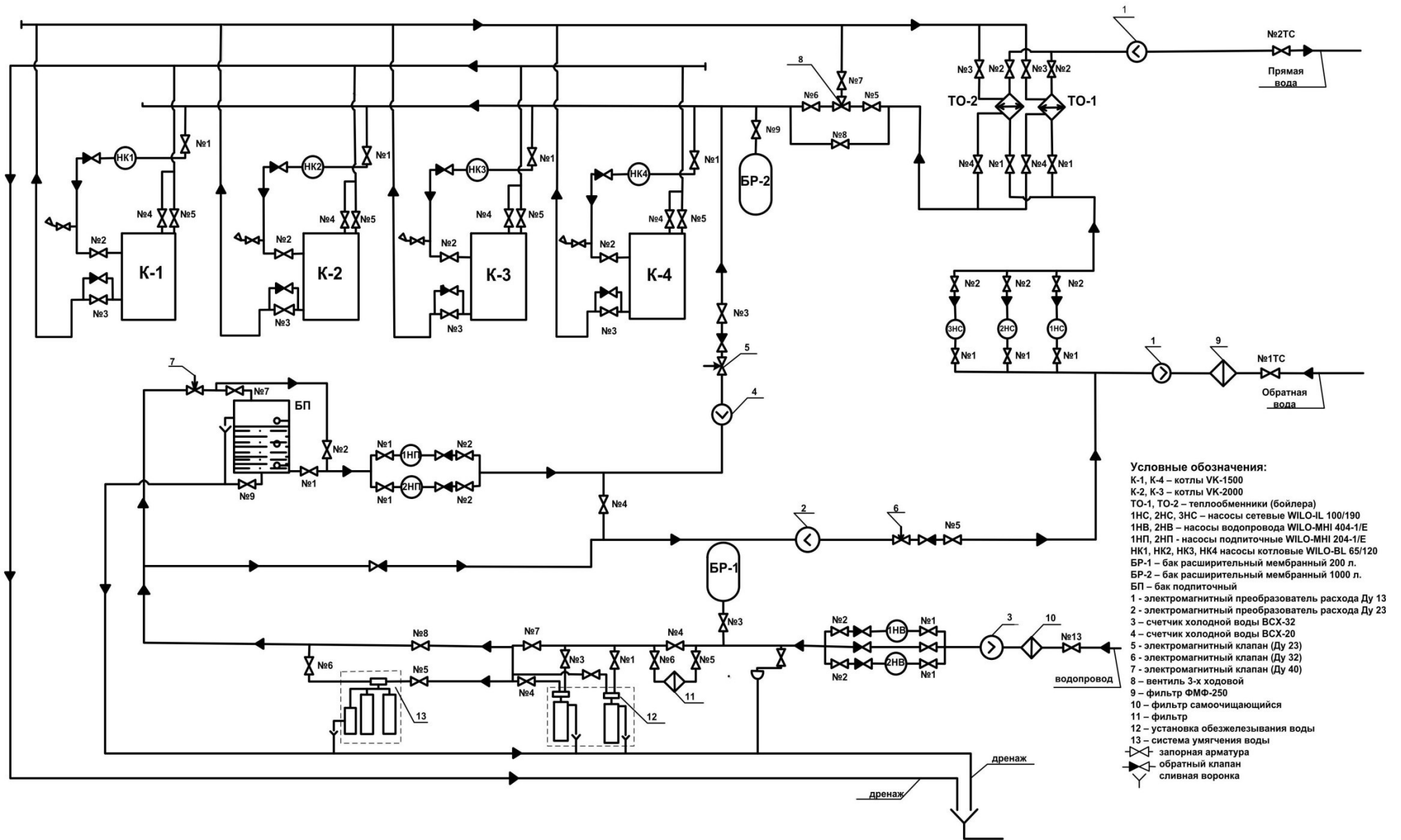
Рис. 2.2.1. Тепловая схема котельной Каринторфф
