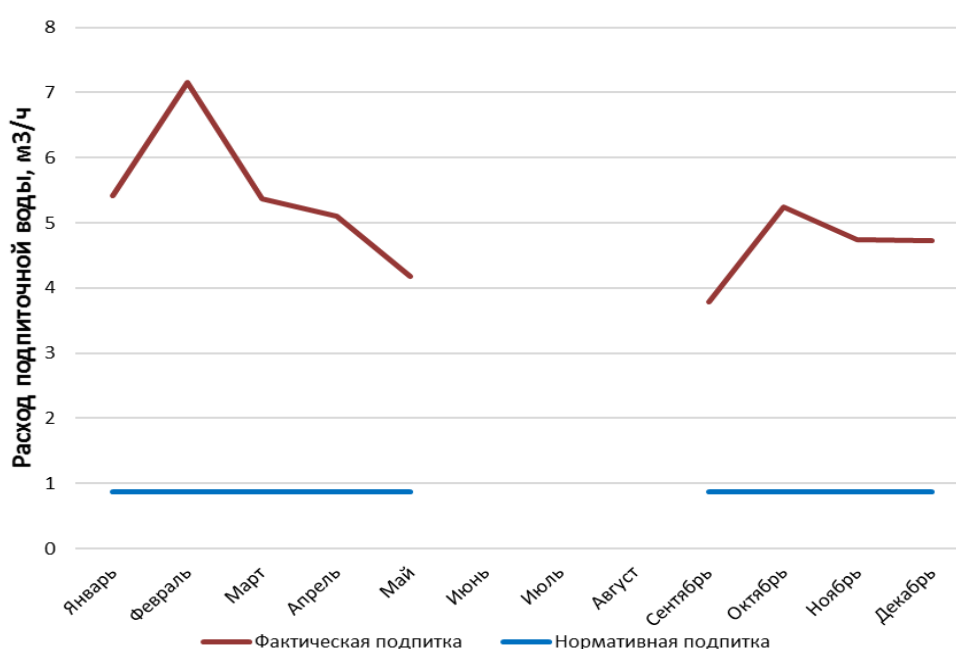
Рис. 7.4.1. Нормативные и фактические ПСВ в тепловых сетях котельной мкр. Каринторфф
