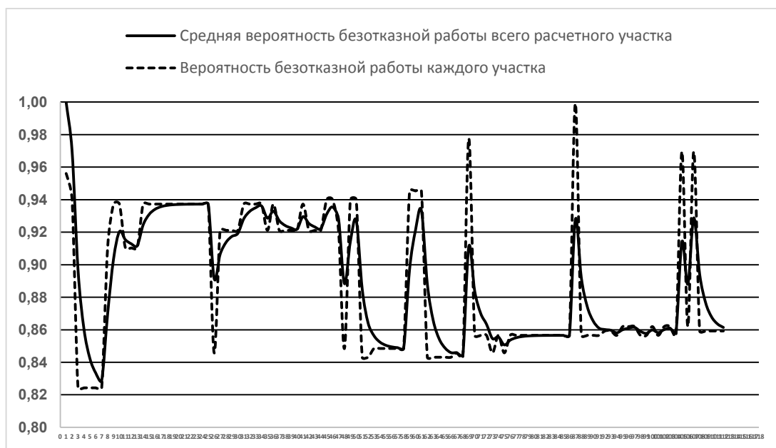
Рис. 9.1.17. Вероятность безаварийной работы тепловой магистрали от ТЭЦ-3 до ТК-4-32 основная
