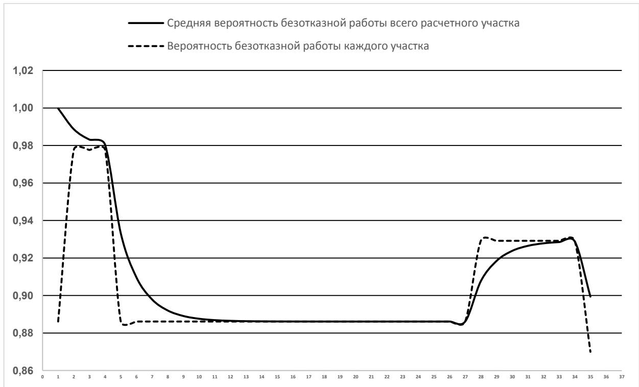
Рис. 9.1.10. Вероятность безаварийной работы тепловой магистрали от Кировской ТЭЦ-3 до ПМК-6
