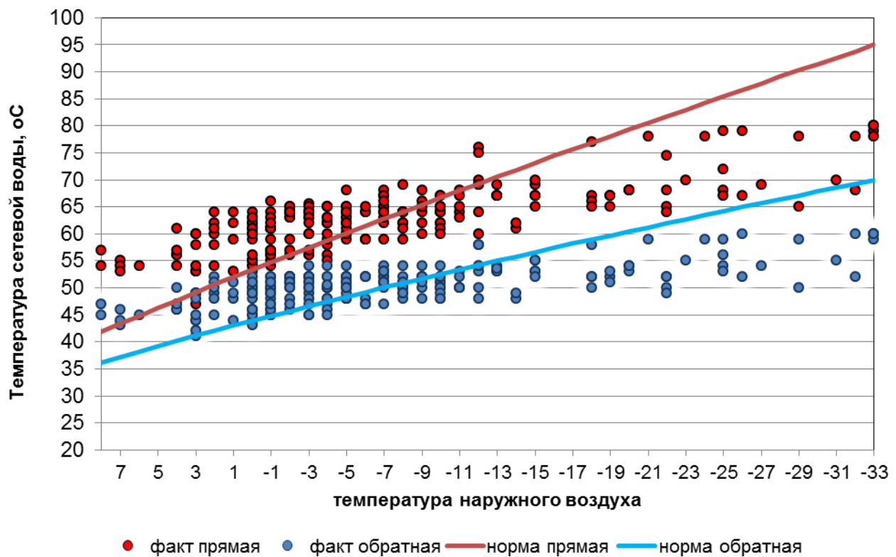
Рис. 3.2.3. Сравнение фактической температуры сетевой воды в подающих и обратных трубопроводах с температурным графиком отпуска тепловой энергии в тепловые сети от котельной микрорайона Каринторф
