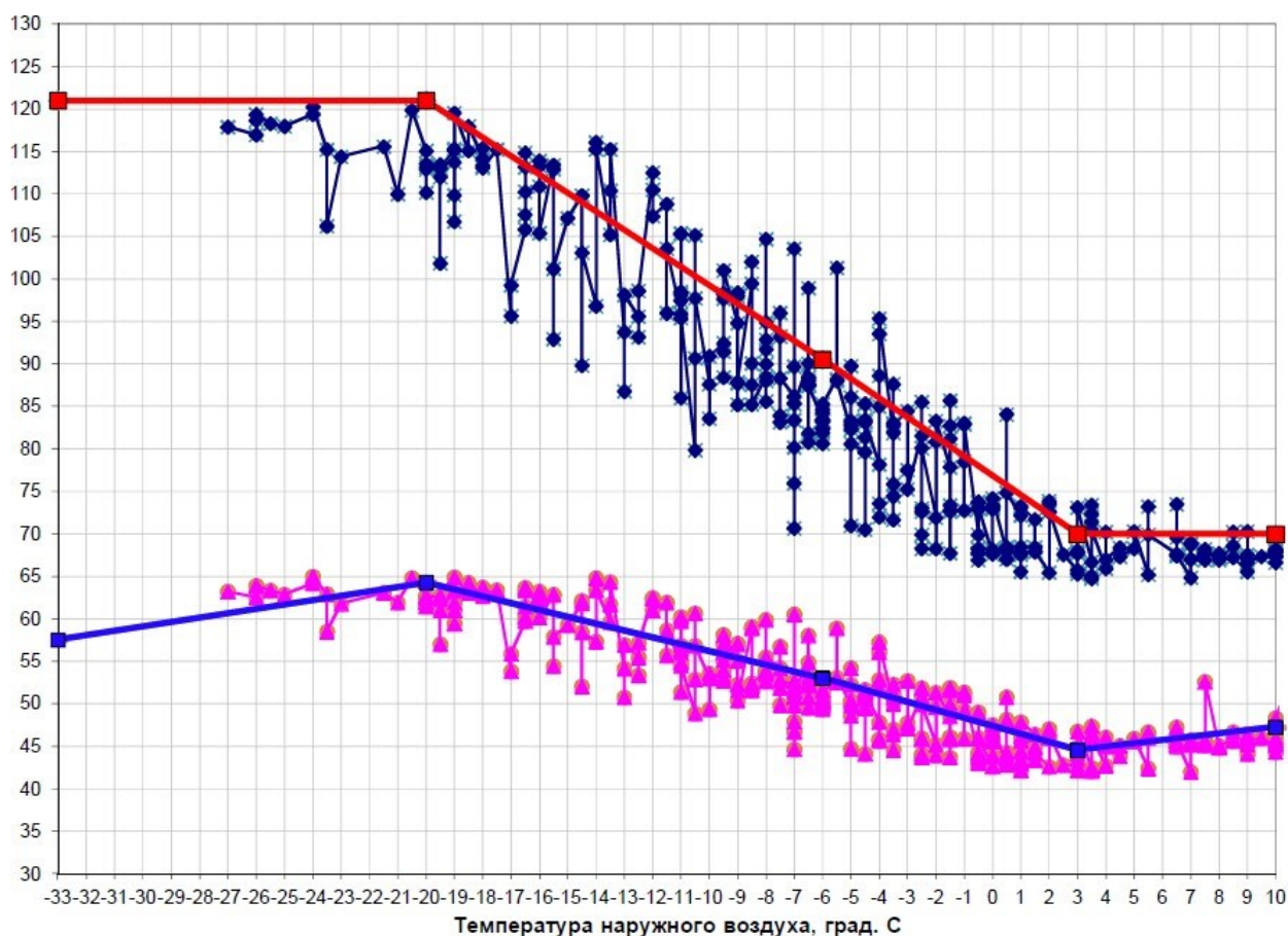
Рис. 3.1.3. Сопоставление фактической температуры сетевой воды в подающих и обратных трубопроводах тепловых сетей АО "КТК" от ТЭЦ-3 г. Кирово-Чепецка с нормируемыми значениями
