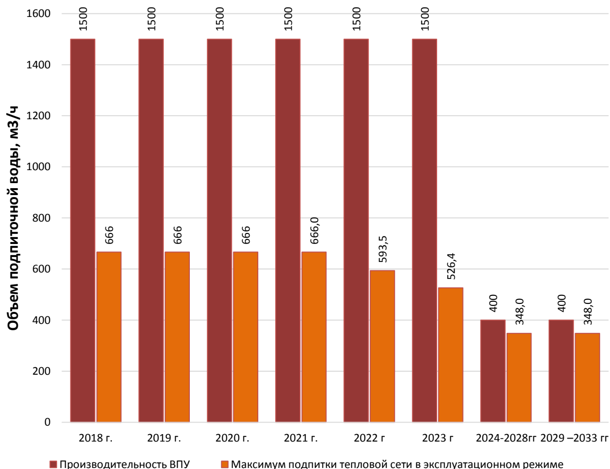
Рис. 7.5.3. Перспективная подпитка тепловой сети и расчетная производительность ВПУ Кировской ТЭЦ-3 для подпитки тепловой сети на период 2018 – 2033 гг.
