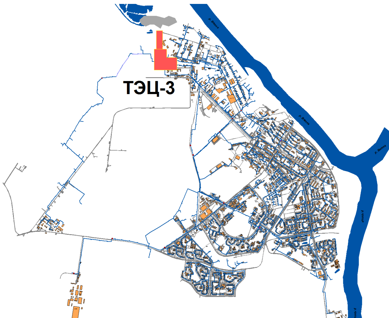
Рис. 3.1.1. Общий вид тепловых сетей в зоне теплоснабжения Кировской ТЭЦ-3
