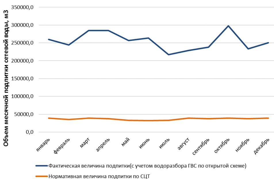
Рис. 7.3.1 Сопоставление нормативной и фактической подпитки тепловой сети с учетом открытого ГВС
