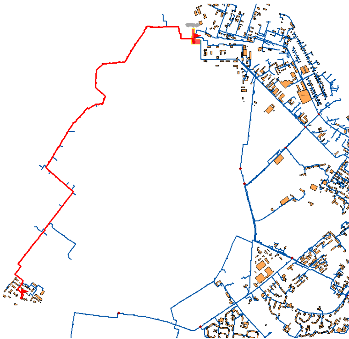
Рис. 9.1.9. Расчетный участок теплосети Кировской ТЭЦ-3 до ПМК-6
