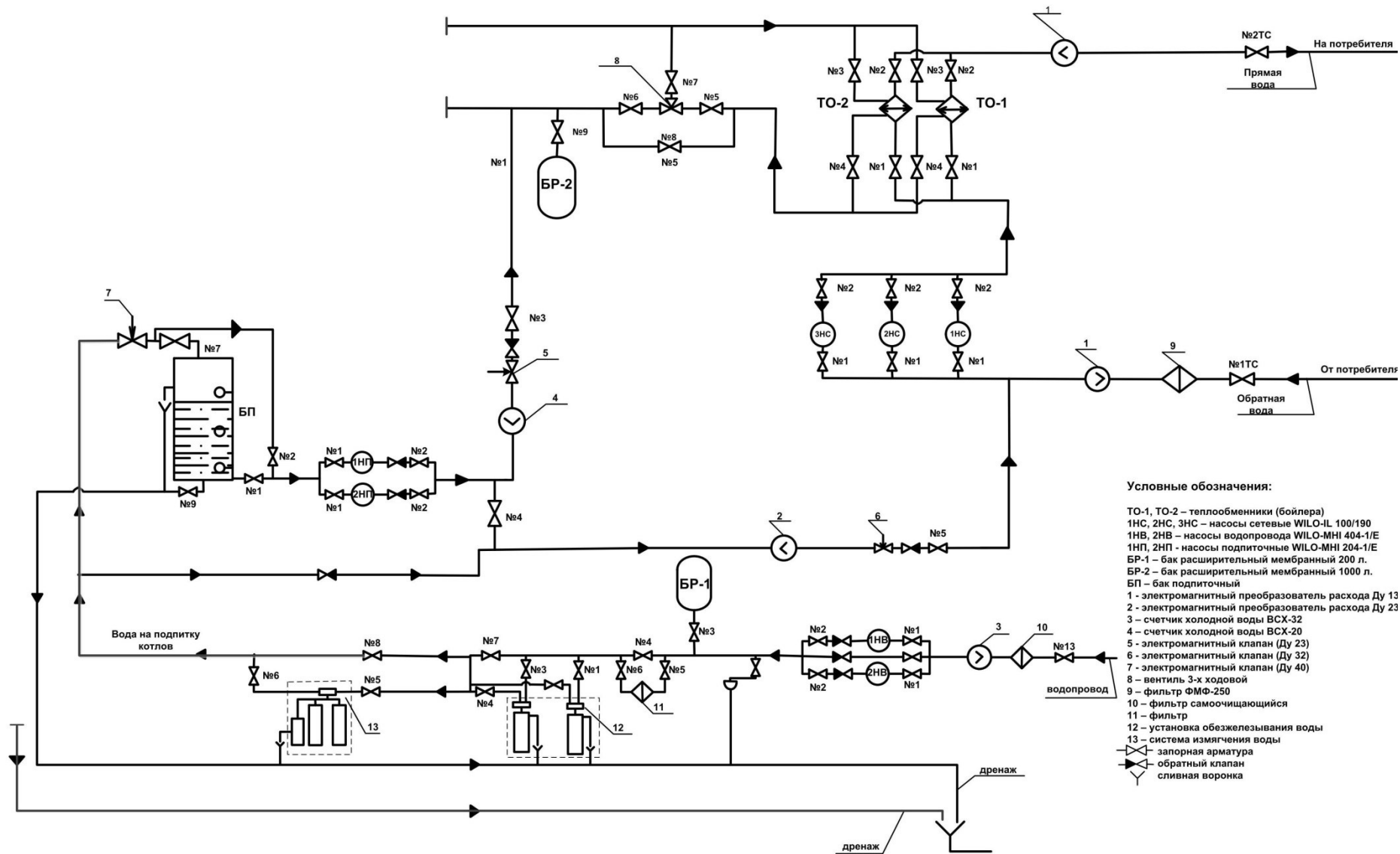
Рис. 2.2.2 Схема выдачи тепловой мощности на котельной микрорайона Каринторф
