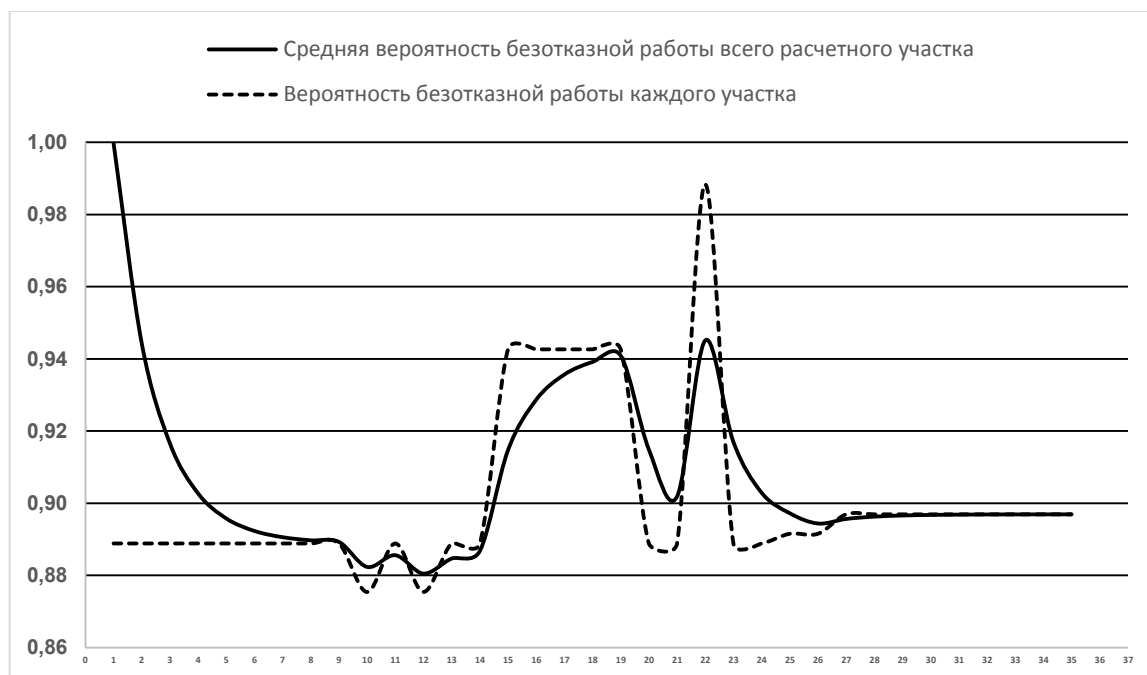
Рис. 9.1.20. Вероятность безаварийной работы тепловой магистрали от Кировской ТЭЦ-3 до 7НО-57 г.
