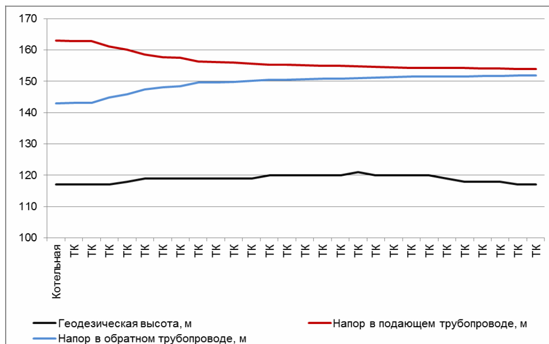
Рис. 3.2.5. Пьезометрический график работы тепловой сети от котельной мкр. Каринторф в 2018 г.
