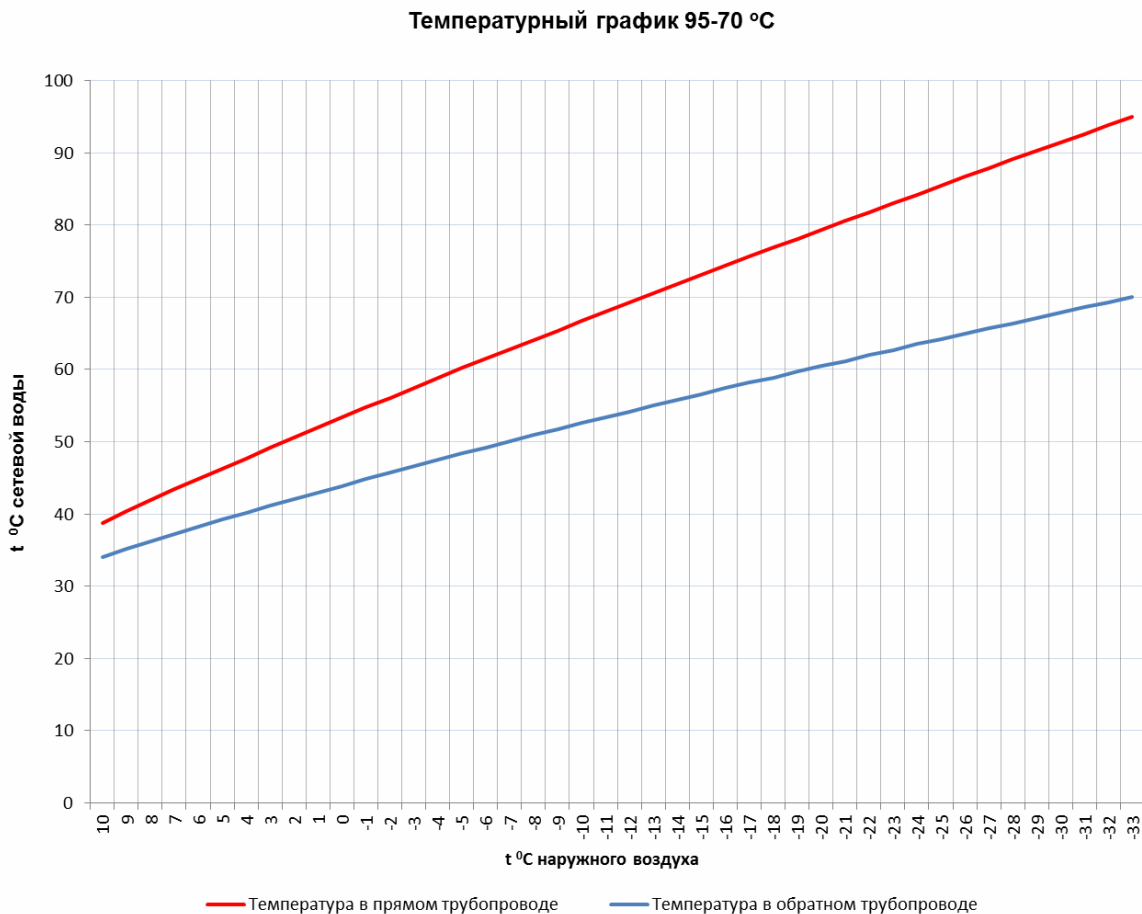
Рис. 3.2.2. Температурный график отпуска тепловой энергии от котельной микрорайона Каринторф
