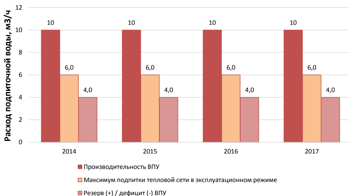
Рис. 7.6.1. Балансы производительности водоподготовительной установки, общей подпитки тепловой сети, резерва/дефицита котельной БМК-8.0 на период 2014-2017 гг.
