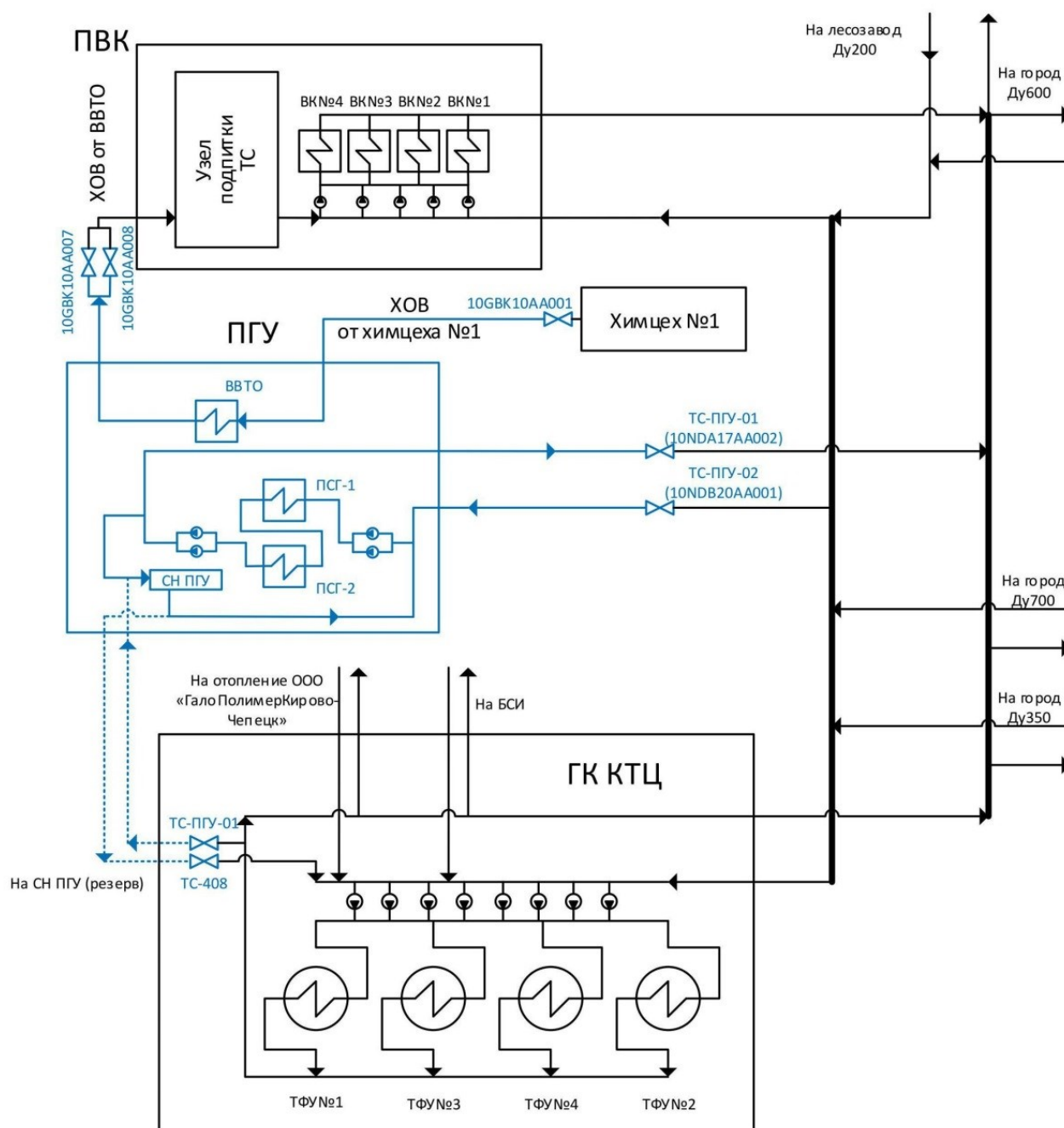
Рис. 2.1.3. Схема выдачи тепловой мощности Кировской ТЭС-3
