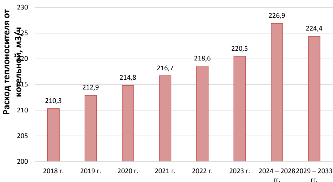
Рис. 7.6.3. Перспективный расход теплоносителя для обеспечения нагрузки на отопление, вентиляцию и ГВС котельной микрорайона Каринторф за период 2018 – 2033 гг.
