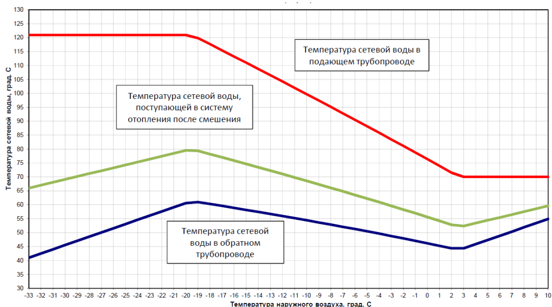
Рис. 3.1.2. Температурный график теплосети в зоне действия Кировской ТЭЦ-3.
