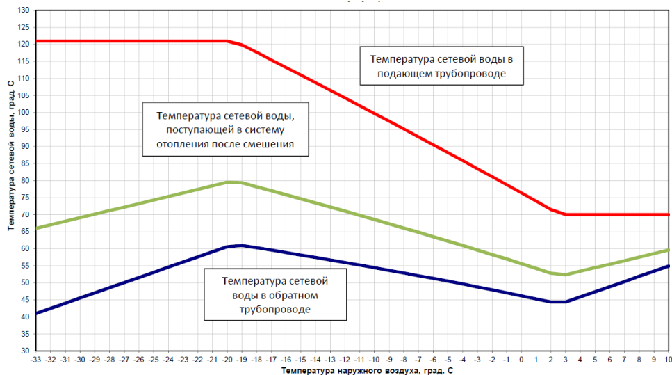
Рис. 2.1.4. Температурный график теплосети Кировской ТЭЦ-3, действовавший до 09.12.2013 года.
