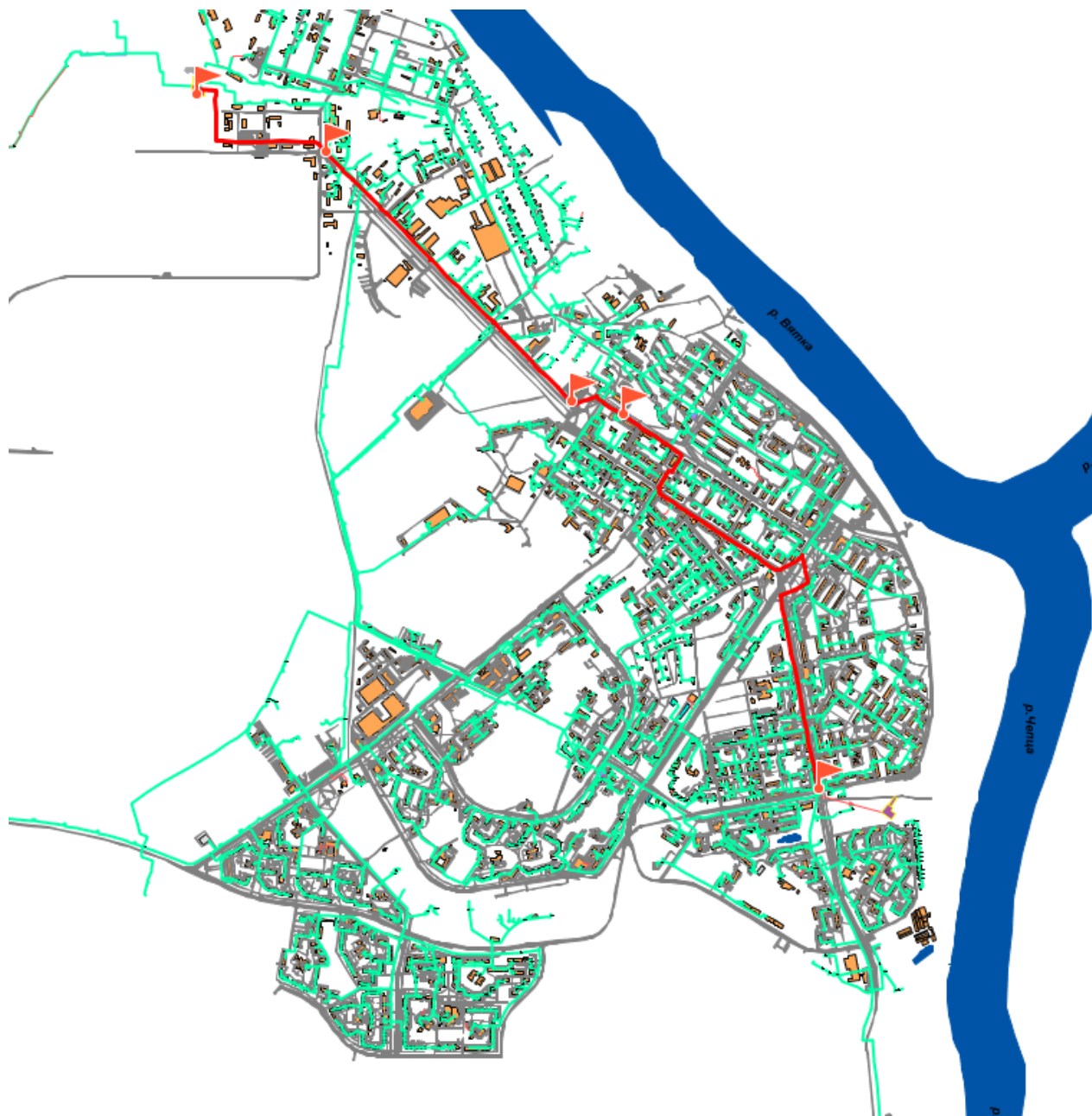
Рис. 9.1.16. Расчетный участок теплосети Кировской ТЭЦ-3 до ТК-4-32
