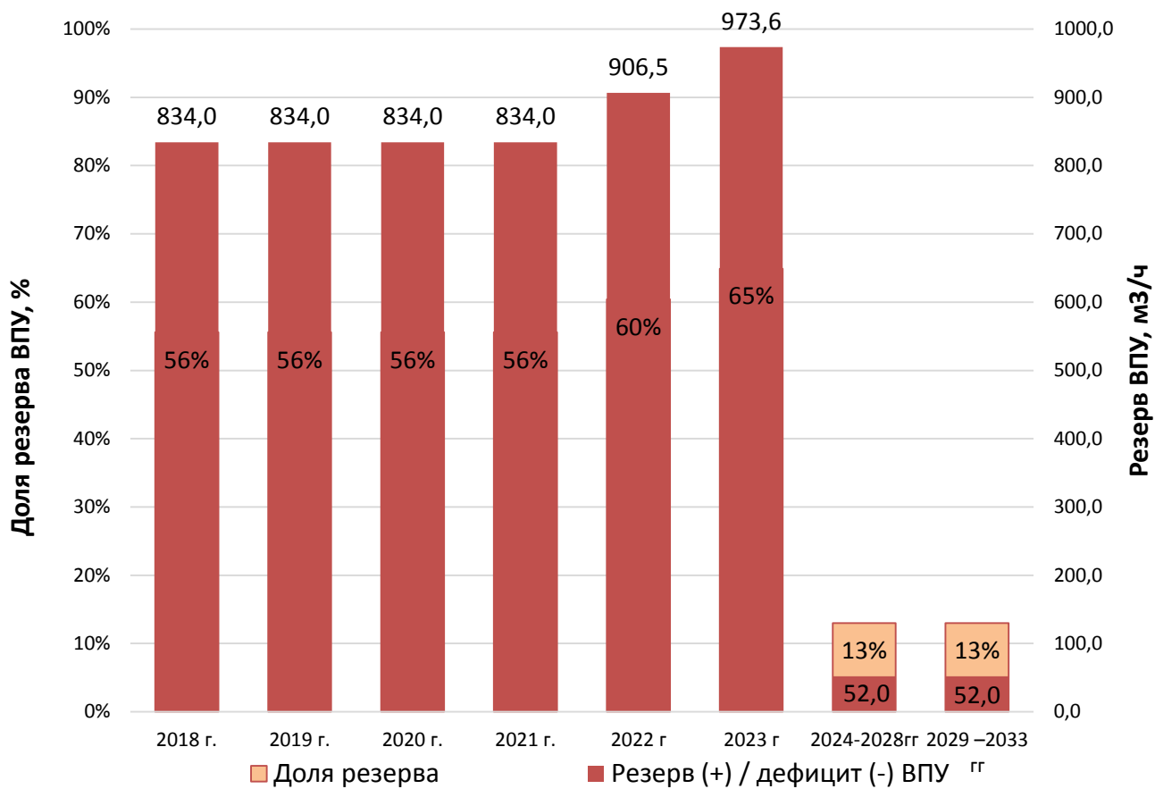
Рис. 7.5.5 Резервы производительности ВПУ Кировской ТЭЦ-3 на период 2018 – 2033 гг.
