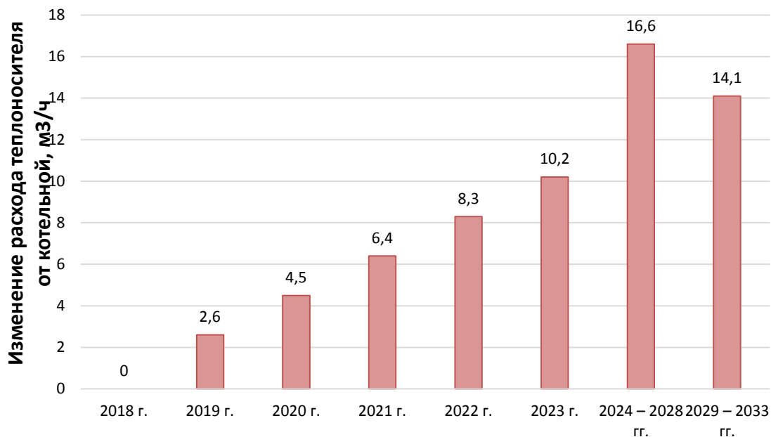
Рис. 7.6.2. Перспективный прирост расхода теплоносителя котельной мкр Каринторф за период 2018-2033 гг.
