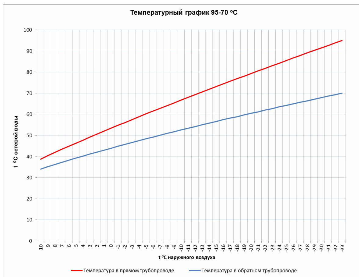
Рис. 2.2.3. Температурный график отпуска тепловой энергии от котельной микрорайона Каринторф
