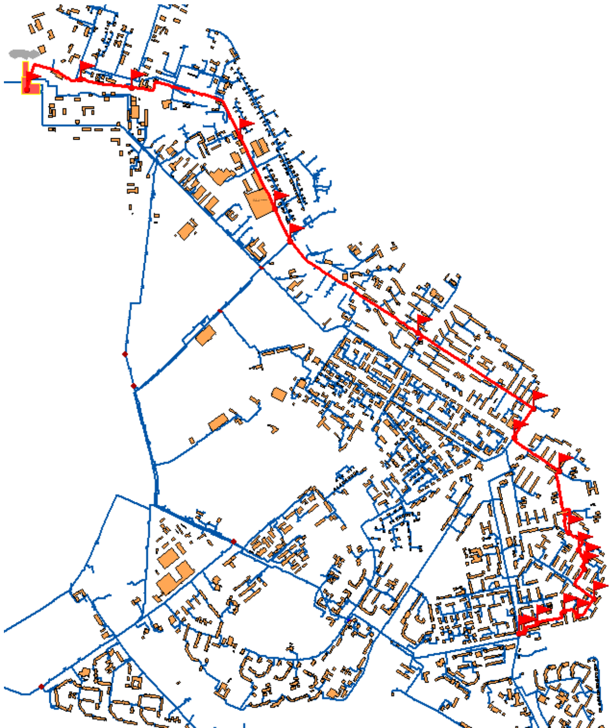
Рис. 9.1.15. Расчетный участок теплосети Кировской ТЭЦ-3 до ТК-4-32
