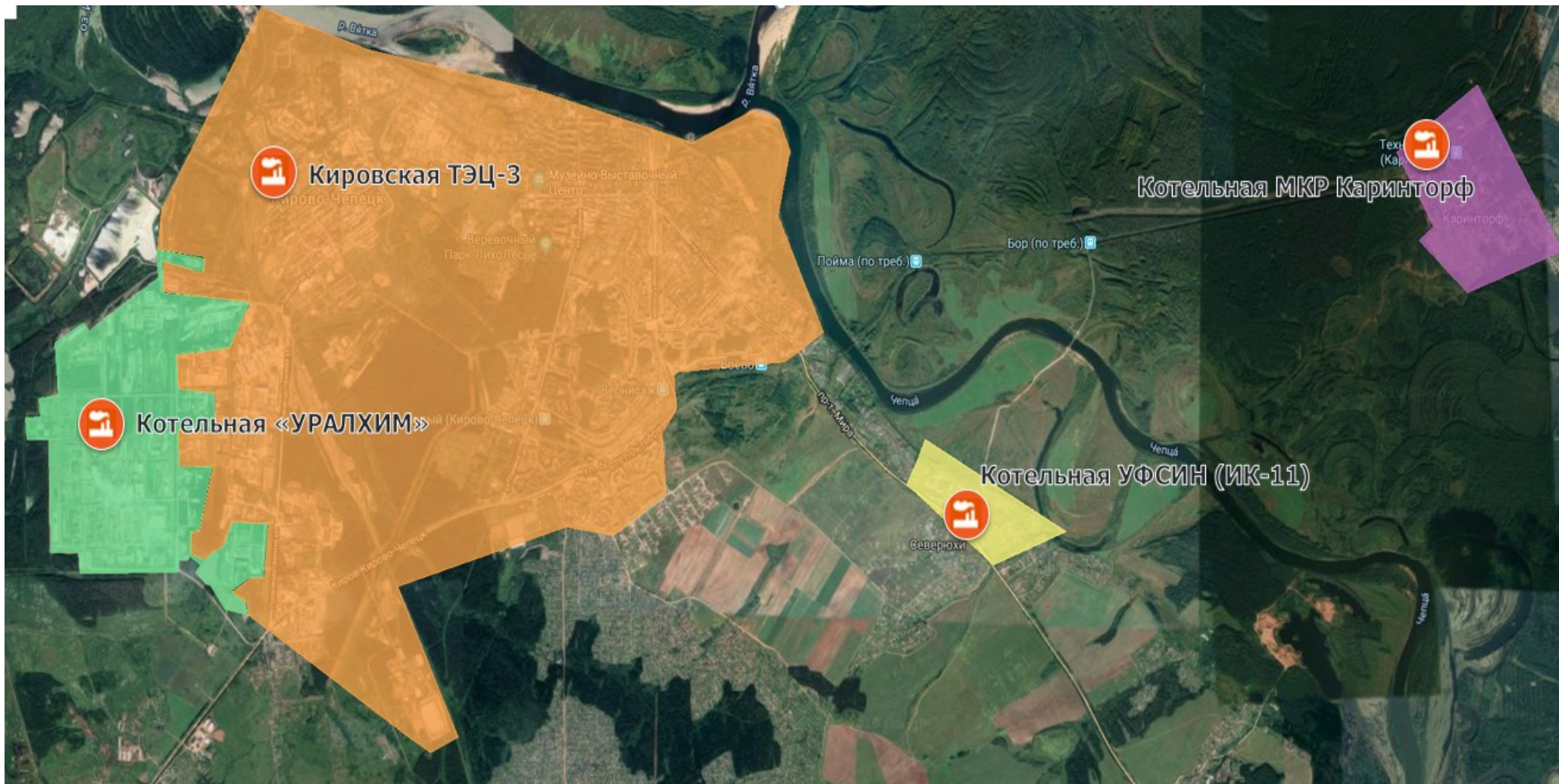
Рис. 2.1.1. Схема расположения источников теплоснабжения в г. Кирово-Чепецк
