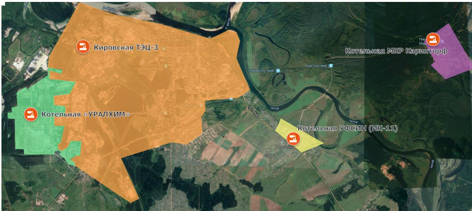
Рис. 2.1.1. Схема расположения источников теплоснабжения в г. Кирово-Чепецк
