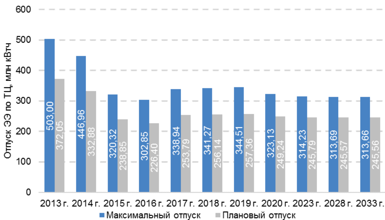
Рис. 3.4. Сопоставление максимального и планового отпуска электроэнергии, выработанной по теплофикационному циклу Кировской ТЭС-3 на 2013 - 2033 гг.
