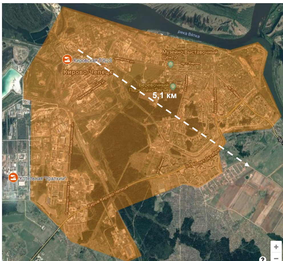
Рис. 2.10.2. Зона действия Кировской ТЭЦ-3 (стрелкой обозначен радиус эффективного теплоснабжения)
