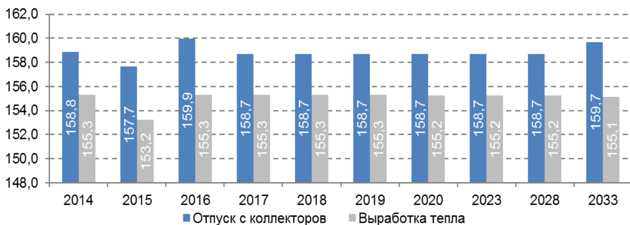
Рис. 5.2.2. Удельный расход условного топлива на выработку тепловой энергии котельной МКР Каринторф на 2013 - 2033 годы, квт/Гкал
