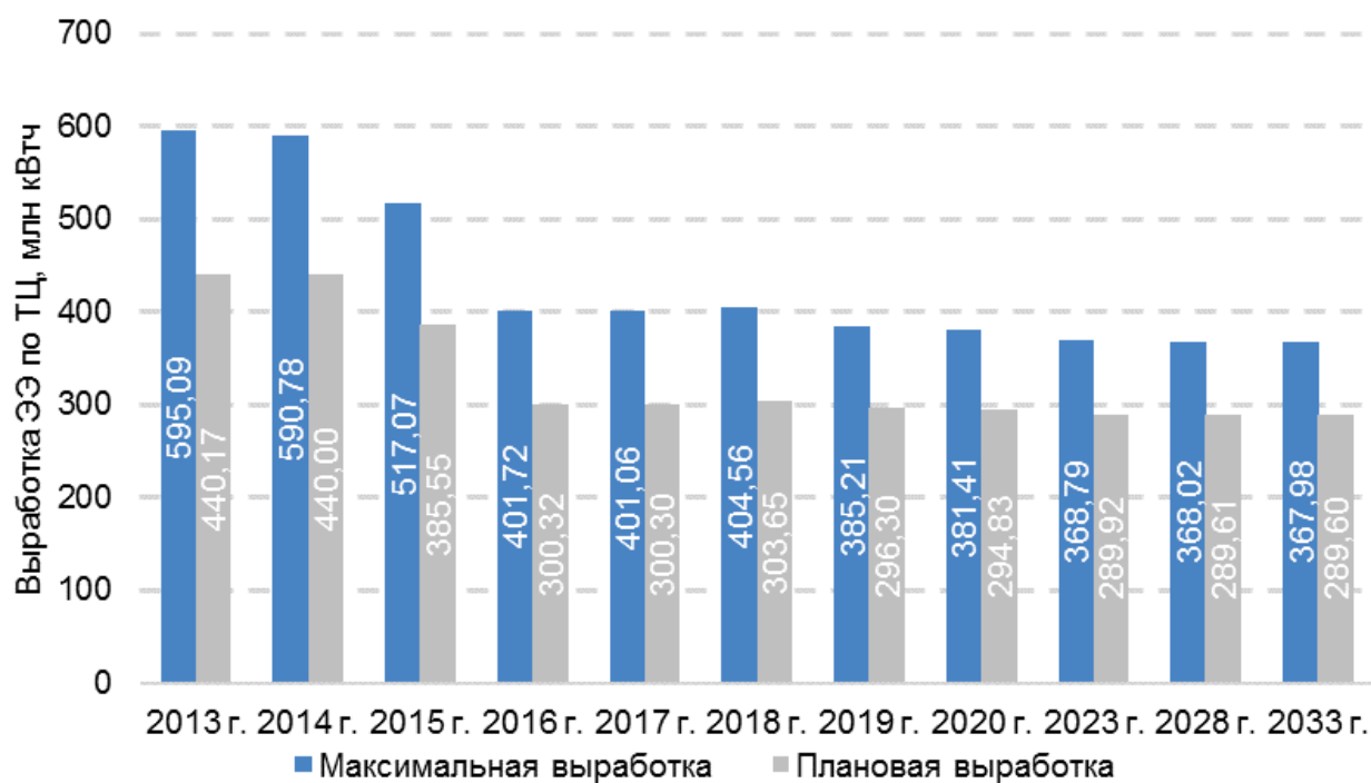
Рис. 3.3. Сопоставление максимальной и плановой выработки электроэнергии по теплофикационному циклу Кировской ТЭС-3 на 2013 - 2033 гг.
