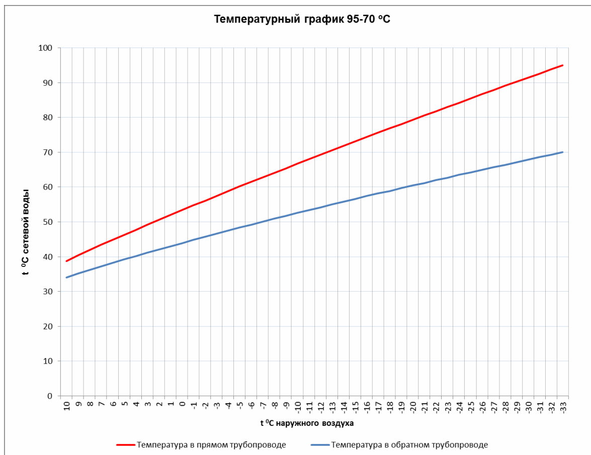
Рис. 5.7.2. Температурный график отпуска тепловой энергии от котельной микрорайона Каринторфф
