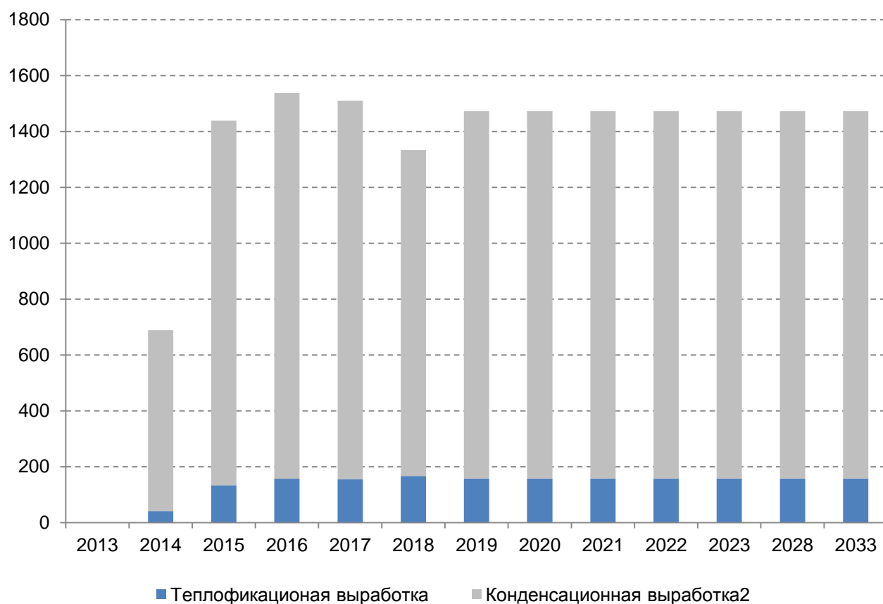
Рис.1.3.3. Выработка электроэнергии по теплофикационному и конденсационному циклам на 2013 - 2033 годы по ПГУ Кировской ТЭС-3, млн. кВтч
