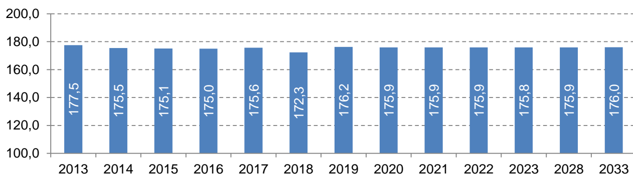
Рис. 1.3.10. Удельные расходы условного топлива на отпуск тепловой энергии в целом по Кировской ТЭЦ-3 на 2013 – 2033 годы, кг/Гкал
