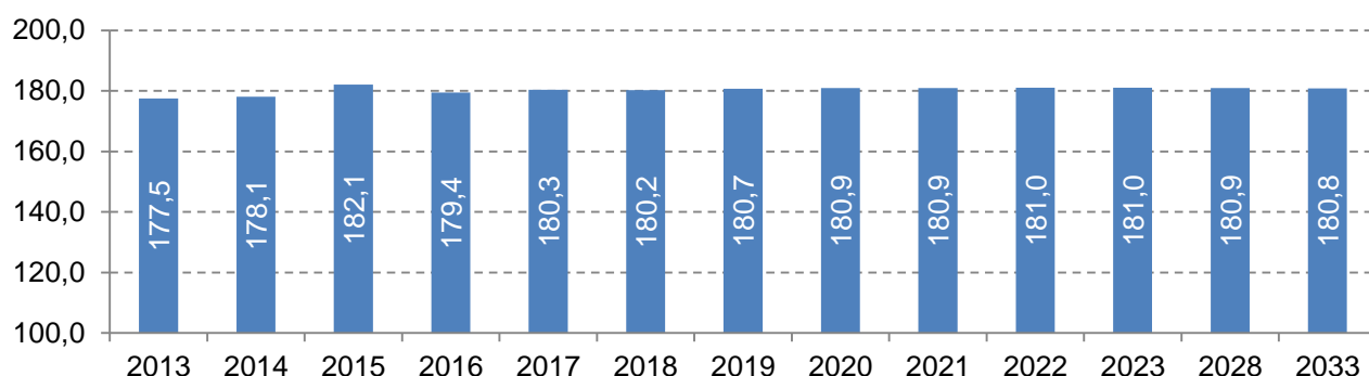
Рис. 1.3.11. Удельные расходы условного топлива на отпуск тепловой энергии по старой части Кировской ТЭЦ-3 на 2013 – 2033 годы, кг/Гкал
