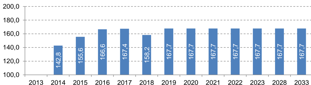
Рис. 1.3.12. Удельные расходы условного топлива на отпуск тепловой энергии по ПГУ Кировской ТЭЦ-3 на 2013 – 2033 годы, кг/Гкал
