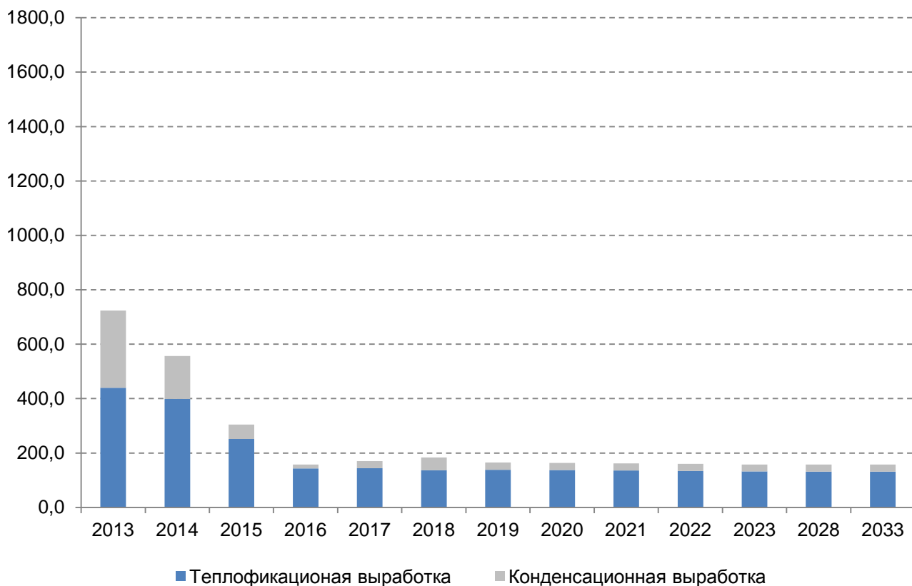
Рис.1.3.2. Выработка электроэнергии по теплофикационному и конденсационному циклам на 2013 - 2033 годы по старой части Кировской ТЭС-3, млн. кВтч
