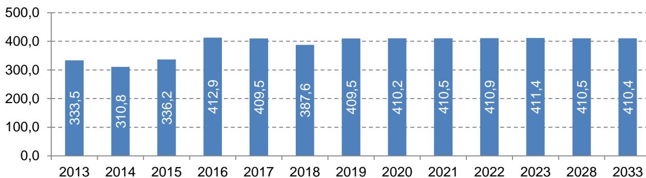
Рис.1.3.5. Удельные расхода условного топлива на отпуск электроэнергии по старой части Кировской ТЭС-3 на 2013 - 2033 годы
