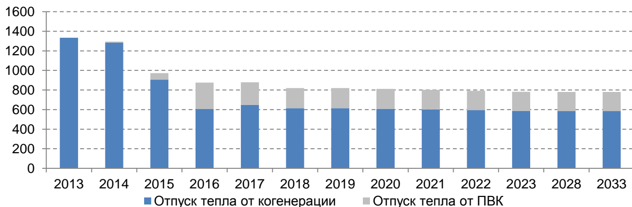
Рис. 1.3.8. Отпуск тепловой энергии внешним потребителям по старой части Кировской ТЭЦ-3 на 2013 - 2033 годы (включая отпуск с паром) , тыс. Гкал
