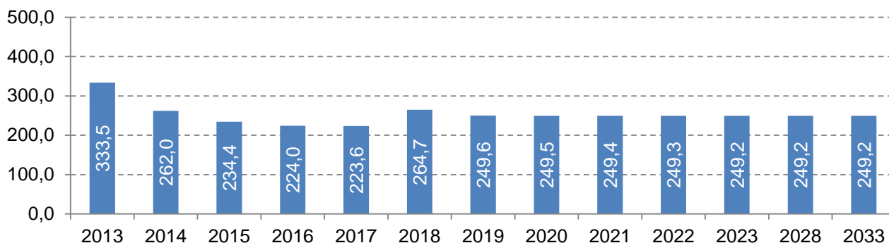
Рис.1.3.4. Удельные расхода условного топлива на отпуск электроэнергии в целом по Кировской ТЭС-3 на 2013 - 2033 годы, гут/кВтч
