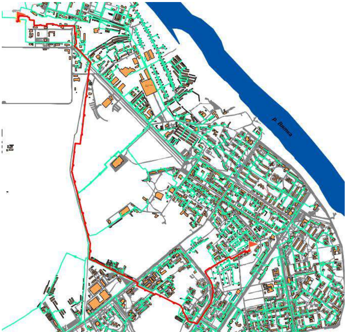
Рис. 2.2.3. Расчетная схема участка тепловой сети от ТЭЦ-3 до Уз. 14-10
