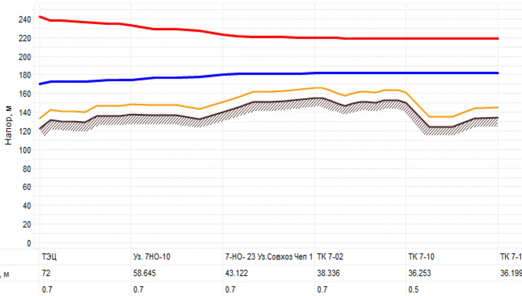
Рис. 2.3.10. Пьезометрический график работы тепловой сети от ТЭЦ-3 до ТК 7-11 в 2033 гг.
