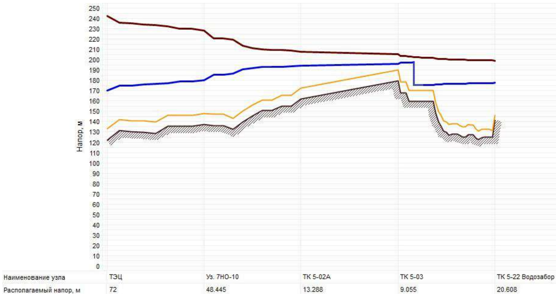
Рис. 2.2.14. Пьезометрический график работы тепловой сети от ТЭЦ-3 до ТК 5-22 2018 г.
