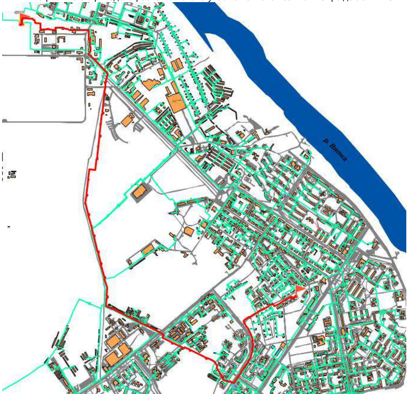
Рис. 2.3.3. Расчетная схема участка тепловой сети от ТЭЦ-3 до Уз. 14-10
