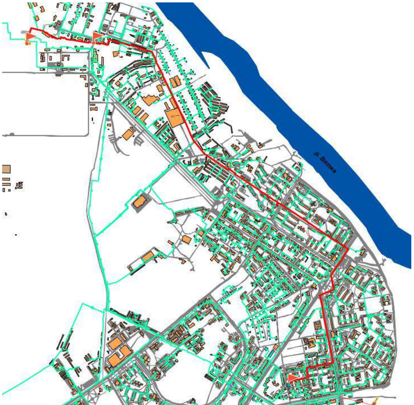
Рис. 2.3.7. Расчетная схема участка тепловой сети от ТЭЦ-3 до ТК 23-5-2
