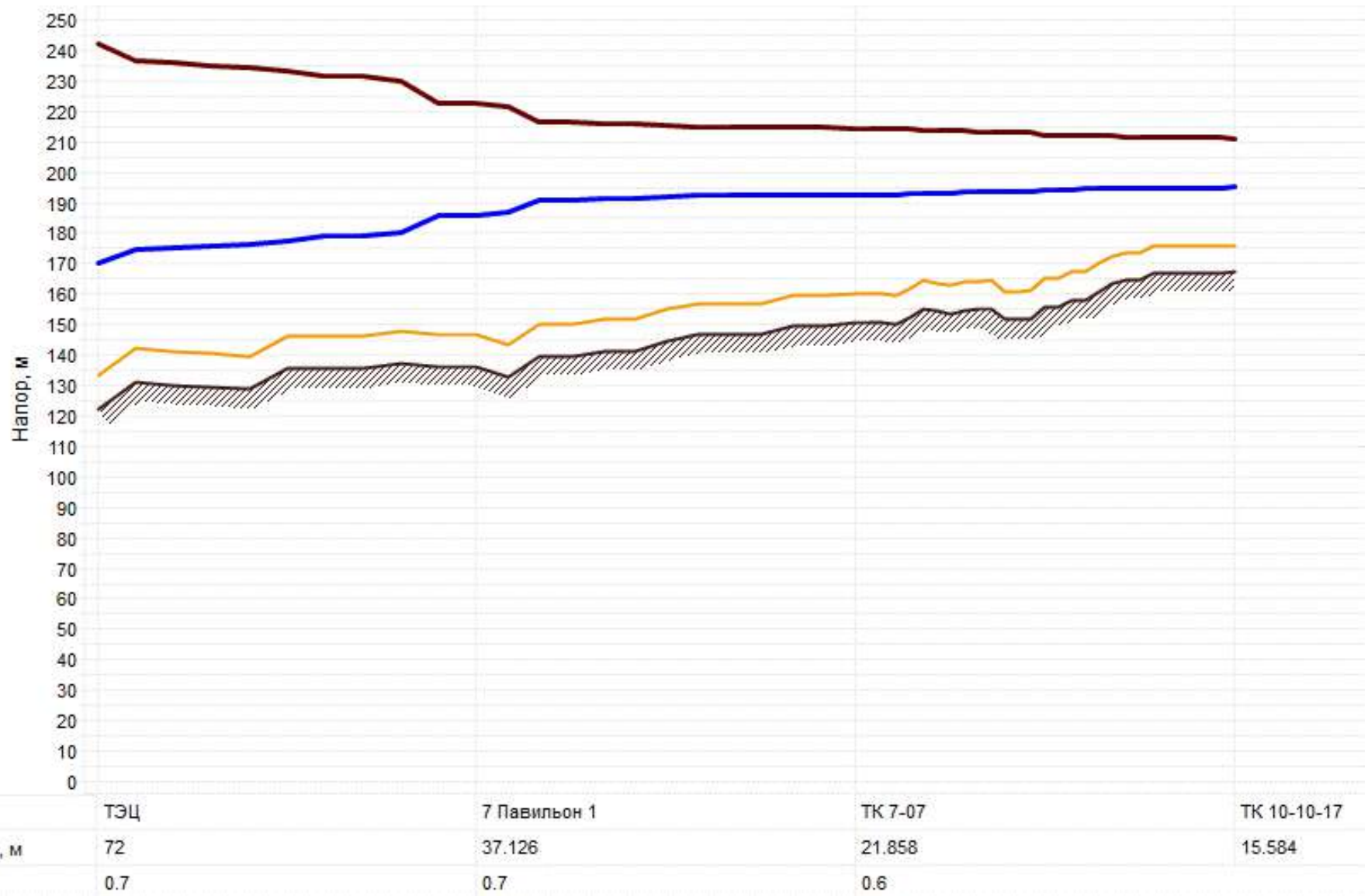
Рис. 2.2.22. Пьезометрический график работы тепловой сети от ТЭЦ-3 до ТК 10-10-17 при строительстве перемычки от тепломагистрали БСИ до тепломагистрали, идущей к базе «ОРСа»
