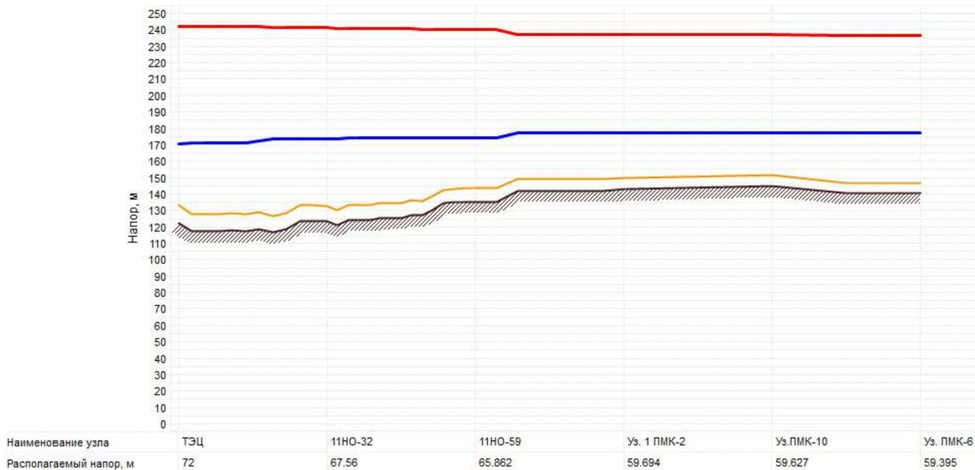
Рис. 2.2.2. Пьезометрический график работы тепловой сети от ТЭЦ-3 до Уз. ПМК-6 в 2018 г.
