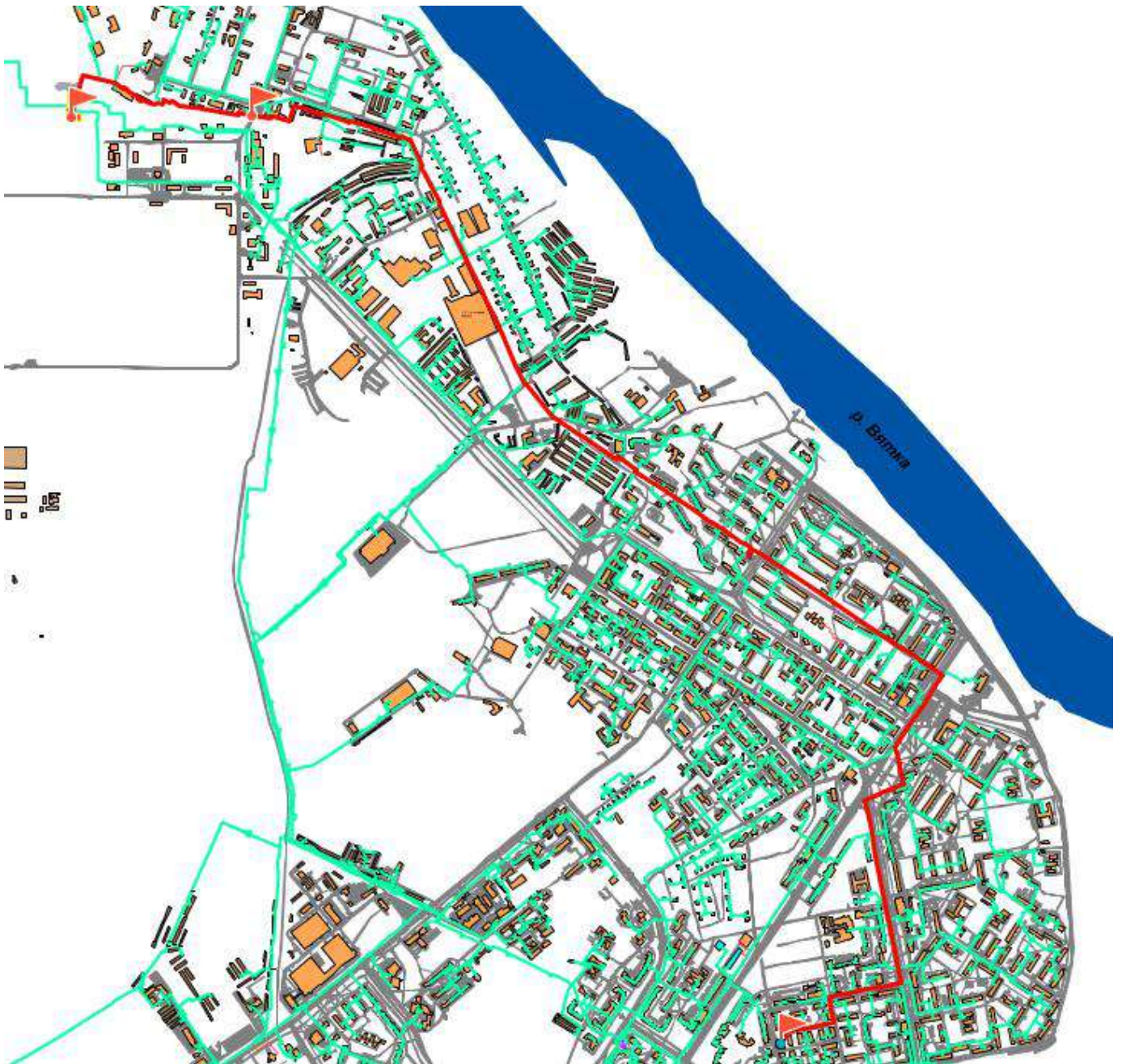
Рис. 2.2.7. Расчетная схема участка тепловой сети от ТЭЦ-3 до ТК 23-5-2
