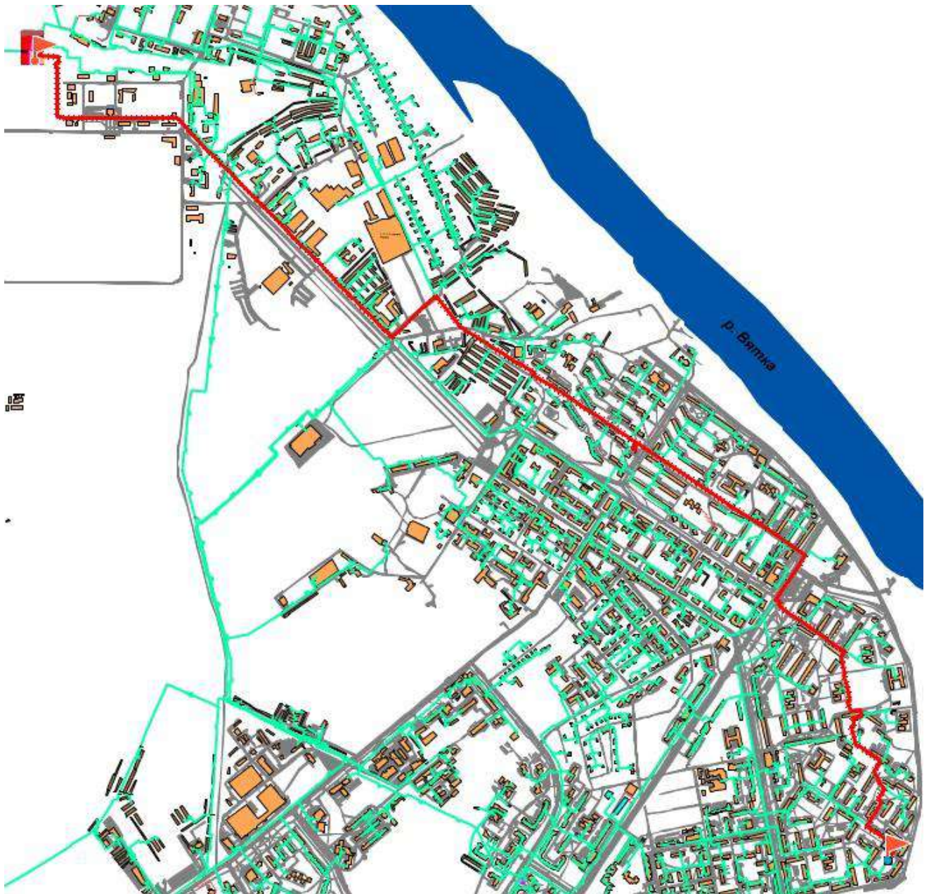
Рис. 2.3.5. Расчетная схема участка тепловой сети от ТЭЦ-3 до ТК 4-32 (через Черемушки)
