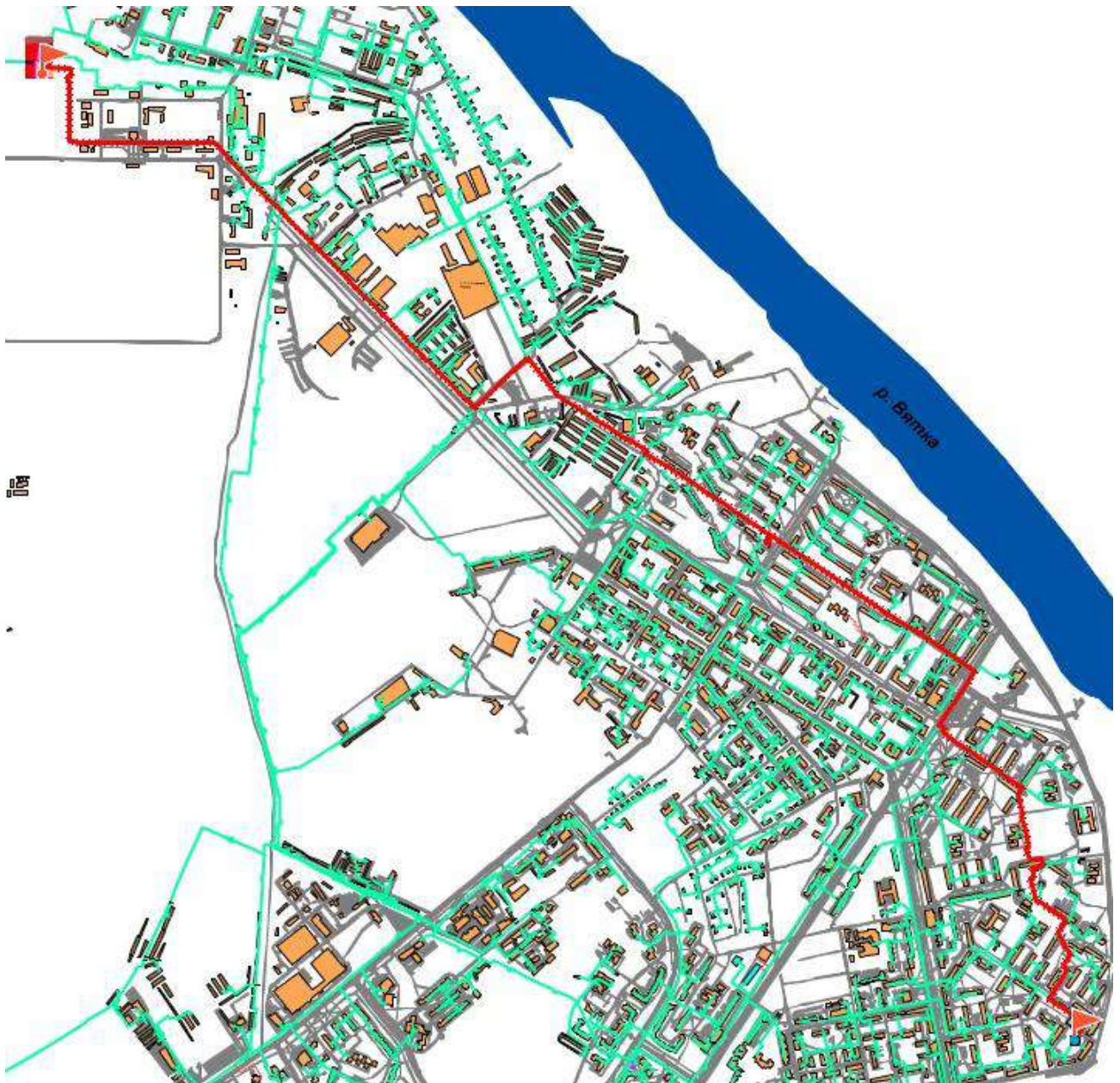
Рис. 2.1.5. Расчетная схема участка тепловой сети от ТЭЦ-3 до ТК 2-24 (через Черемушки)
