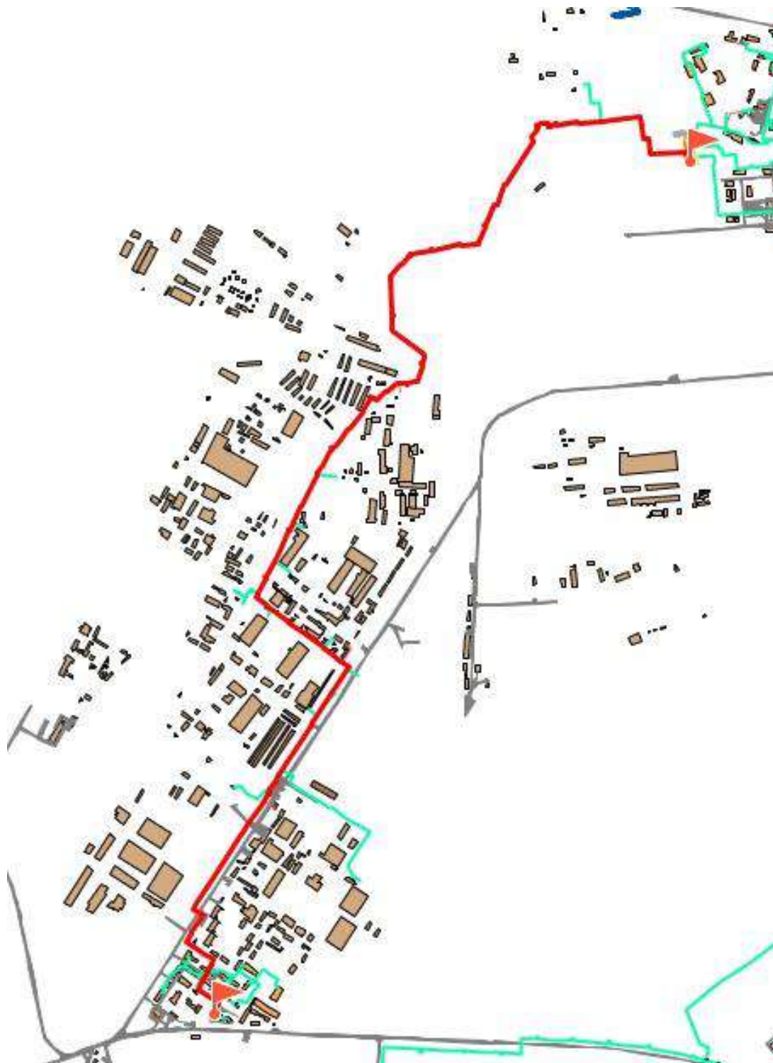
Рис. 2.2.1. Расчетная схема участка тепловой сети от ТЭЦ-3 до Уз. ПМК-6
