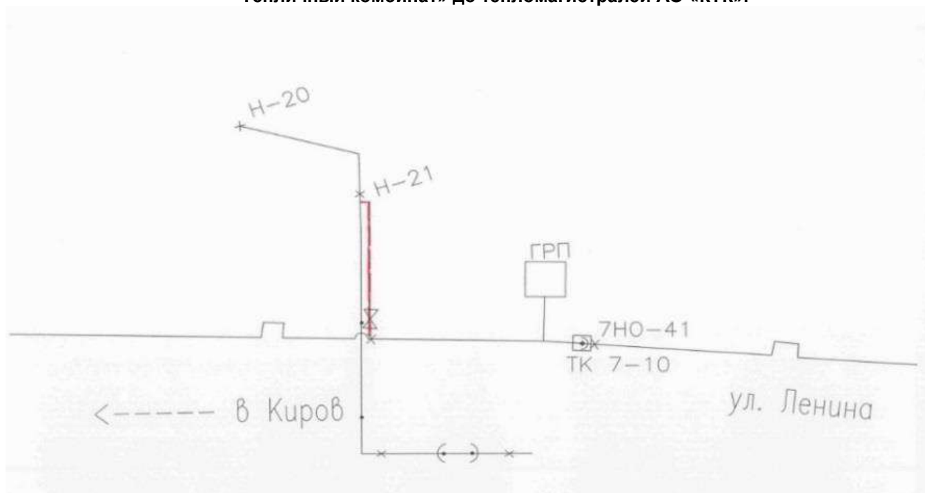
Рис. 2.2.19. Строительство перемычки схемы от тепломагистральной «Чепецкий Тепличный комбинат» до тепломагистралей АО «КТК».
