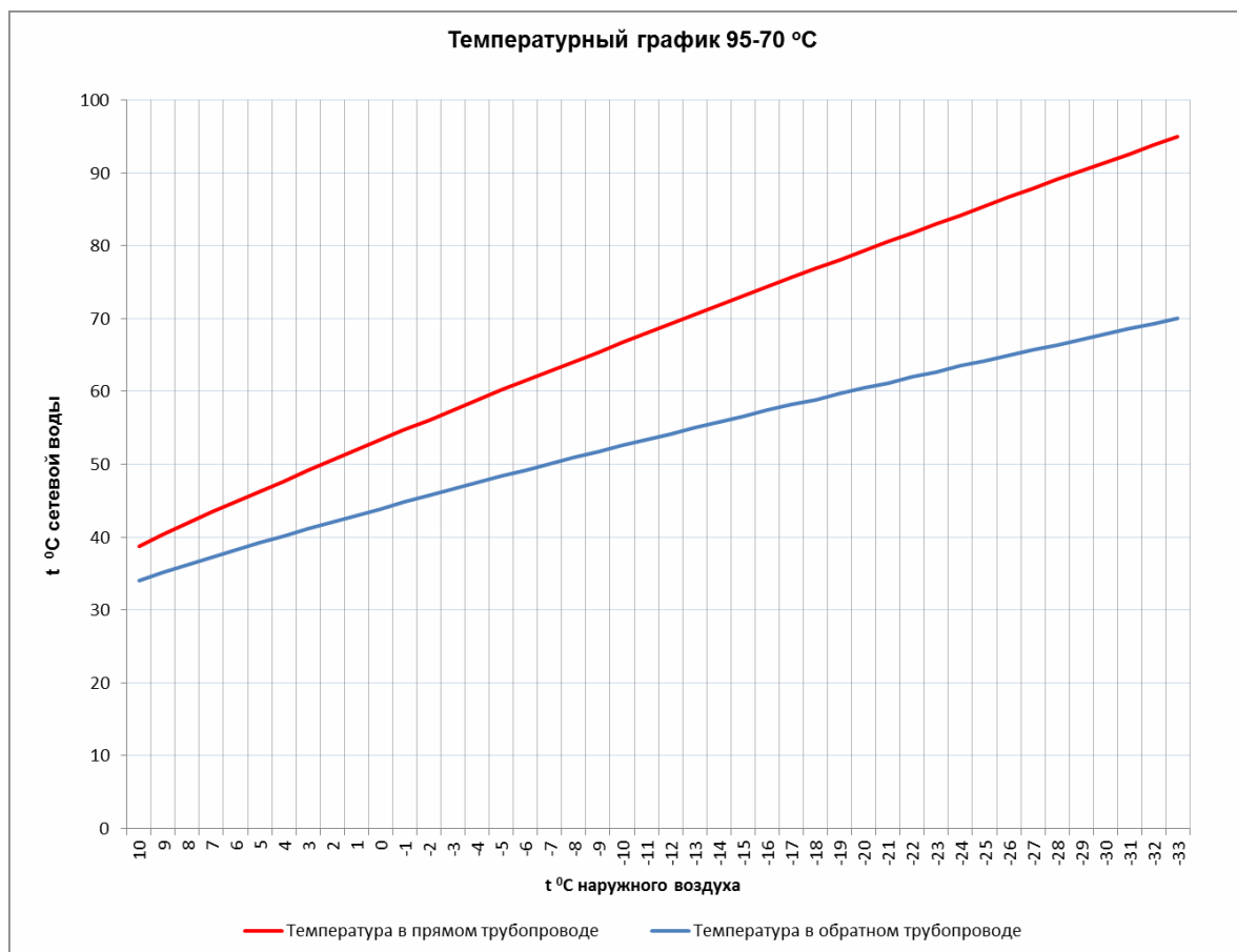
Рис. 5.7.2. Температурный график отпуска тепловой энергии от котельной микрорайона Каринторф
