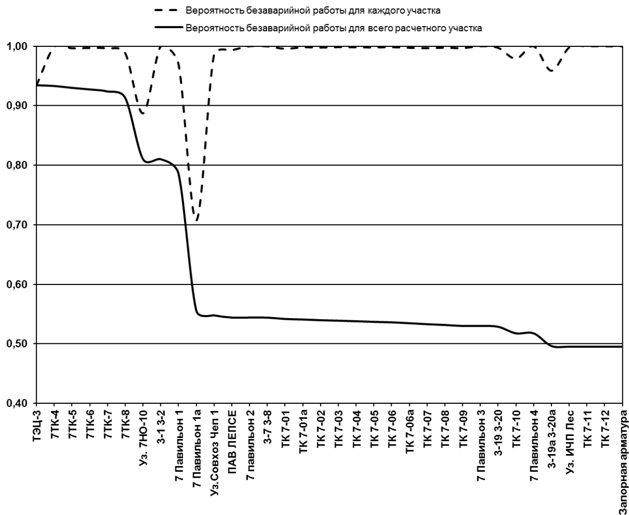
Рис. 2.1.24. Вероятность безаварийной работы тепловой магистрали от Кировской ТЭС-3 до 7НО-57 в 2014 г.
