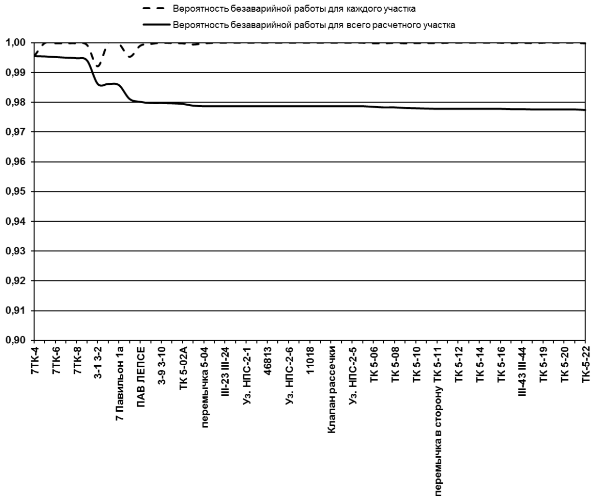
Рис. 2.1.25. Вероятность безаварийной работы тепловой магистрали от Кировской ТЭЦ-3 до ТК-5-22 в 2033 г.
