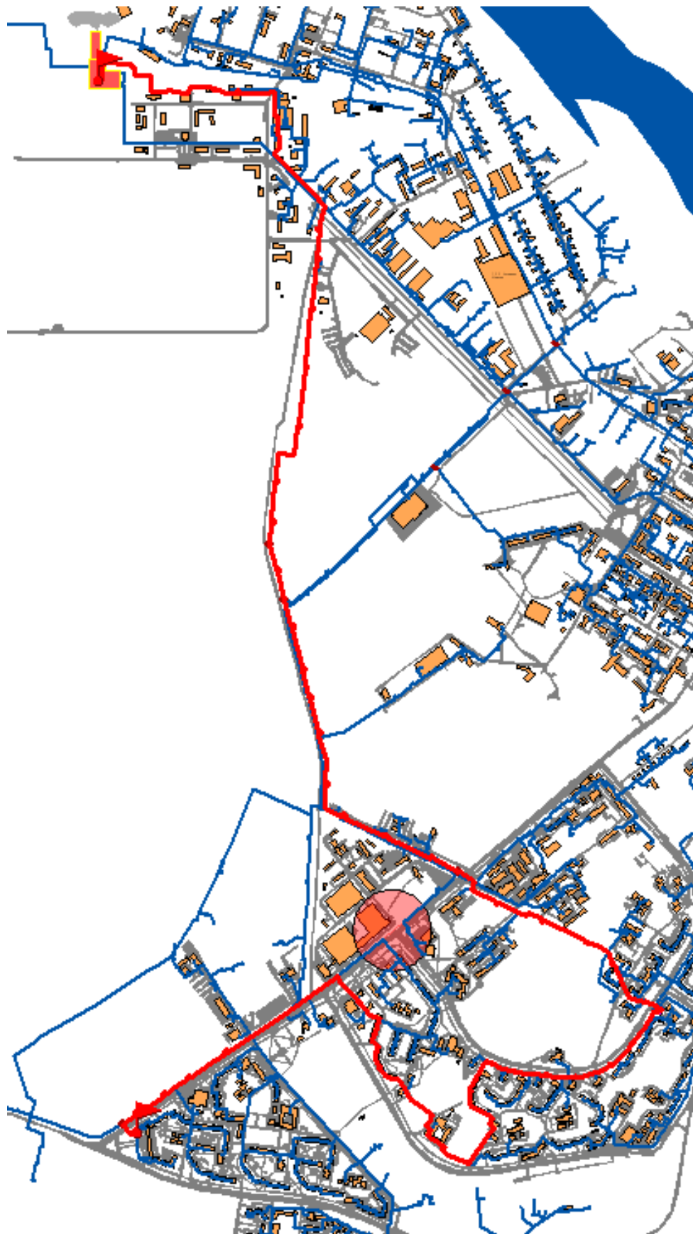
Рис. 3.2.2. Отключенный участок ТК 7-02 – ТК 7-03 тепловой сети Кировской ТЭЦ-3
