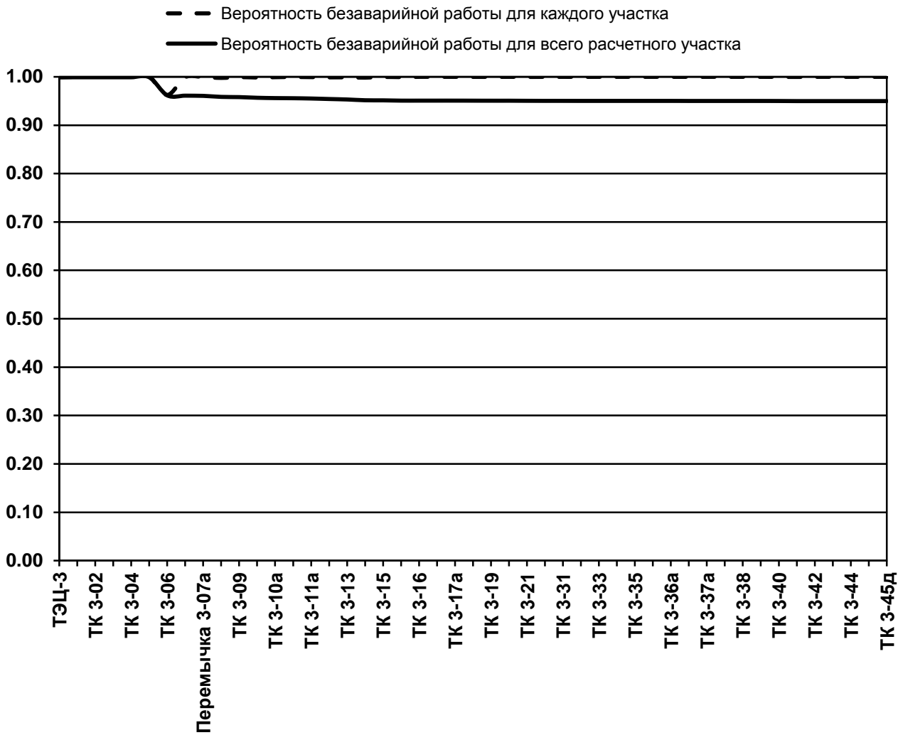
Рис. 2.1.7. Вероятность безаварийной работы тепловой магистрали от Кировской ТЭЦ-3 до Уз 3-47 в 2033 г.
