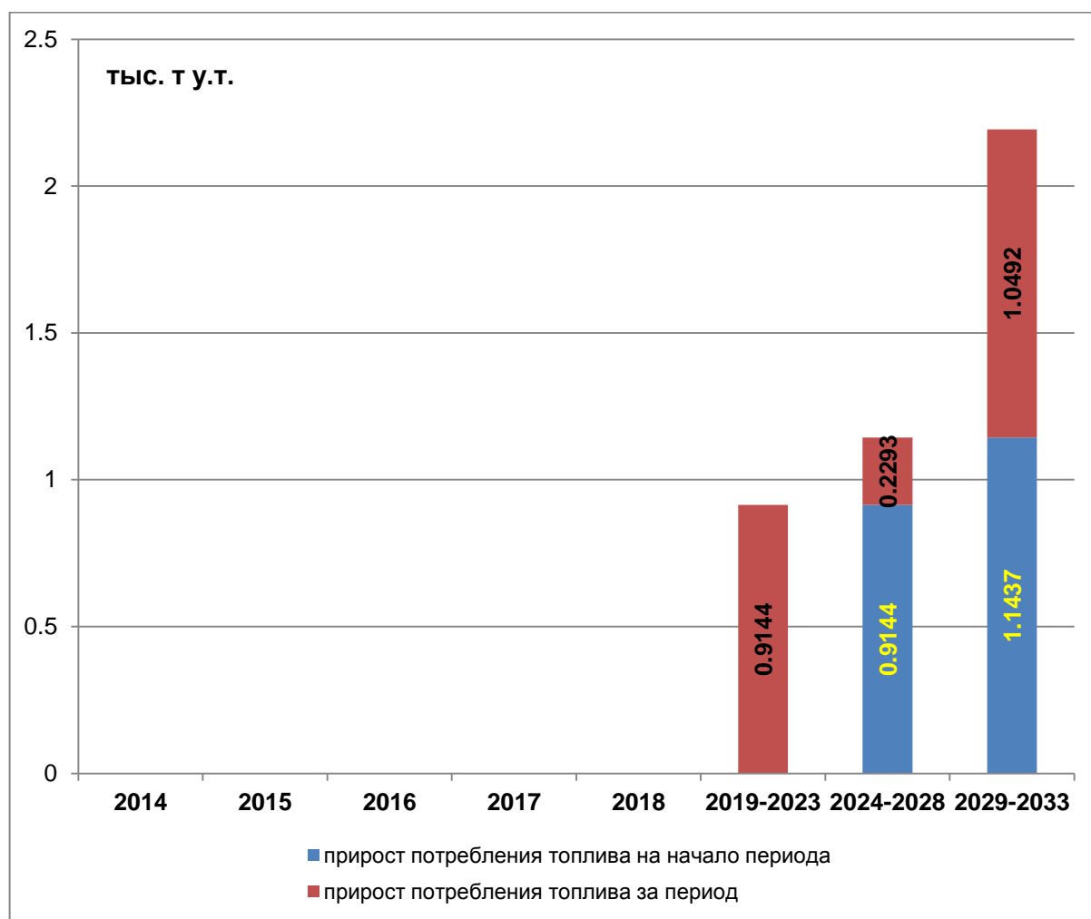
Рис. 2.7.1. Прогнозируемый прирост расхода природного газа на Кировской ТЭЦ-3 для обеспечения теплоснабжения потребителей в зоне нового строительства № 7 в период 2015 – 2033 гг.
