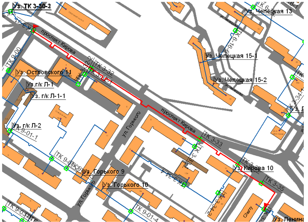
Рис. 4.6. Участок тепломагистрали от ТК3-31 до ТК3-36
