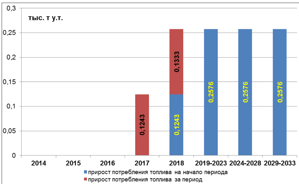
Рис. 2.3.3. Прогнозируемый прирост расхода природного газа для обеспечения теплоснабжения объектов ИЖС в зоне нового строительства № 3 в период 2015 – 2033 гг.
