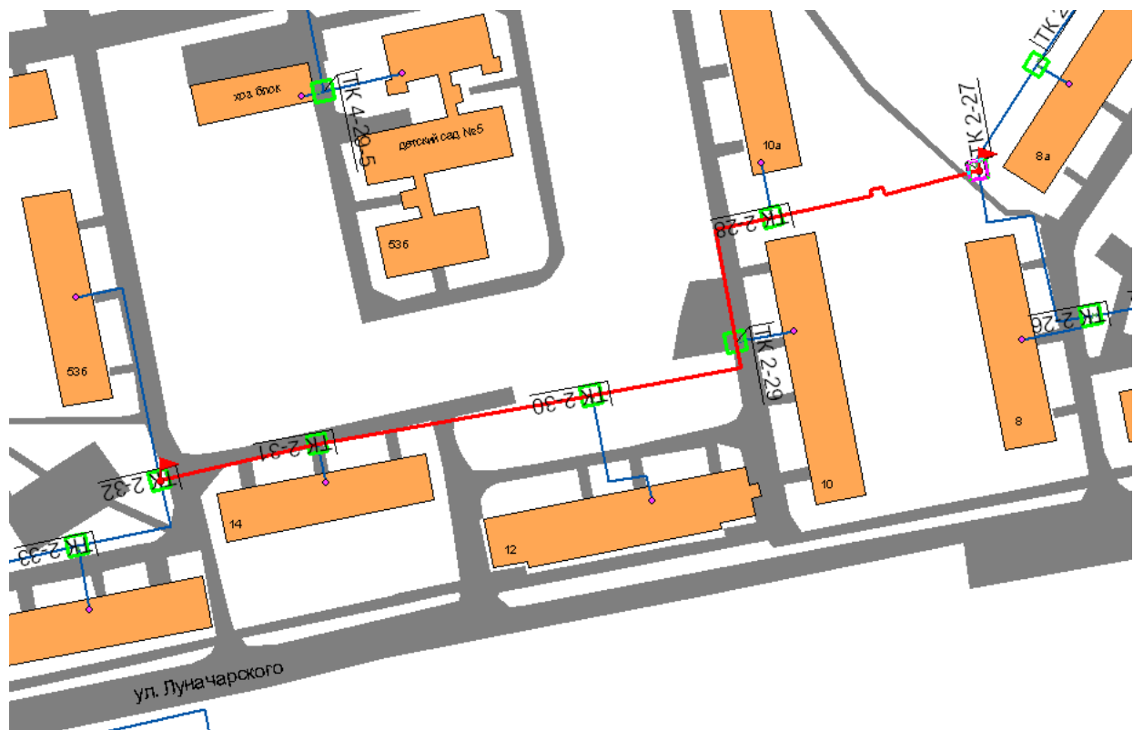
Рис. 4.12. Участок тепломагистрали отTK2-27 до ТК2-32
