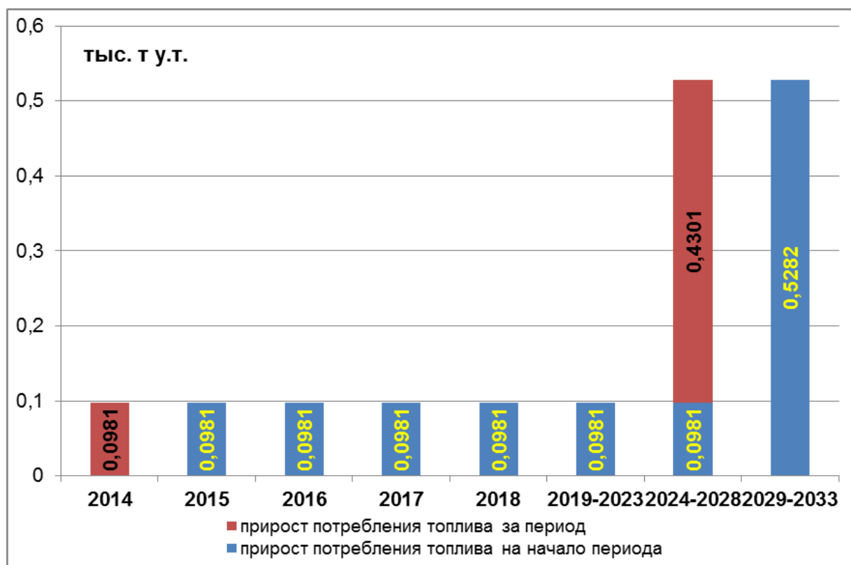
Рис. 2.5.2. Прогнозируемый прирост расхода природного газа на Кировской ТЭЦ-3 для обеспечения теплоснабжения потребителей в зоне нового строительства № 5 в период 2015 – 2033 гг.
