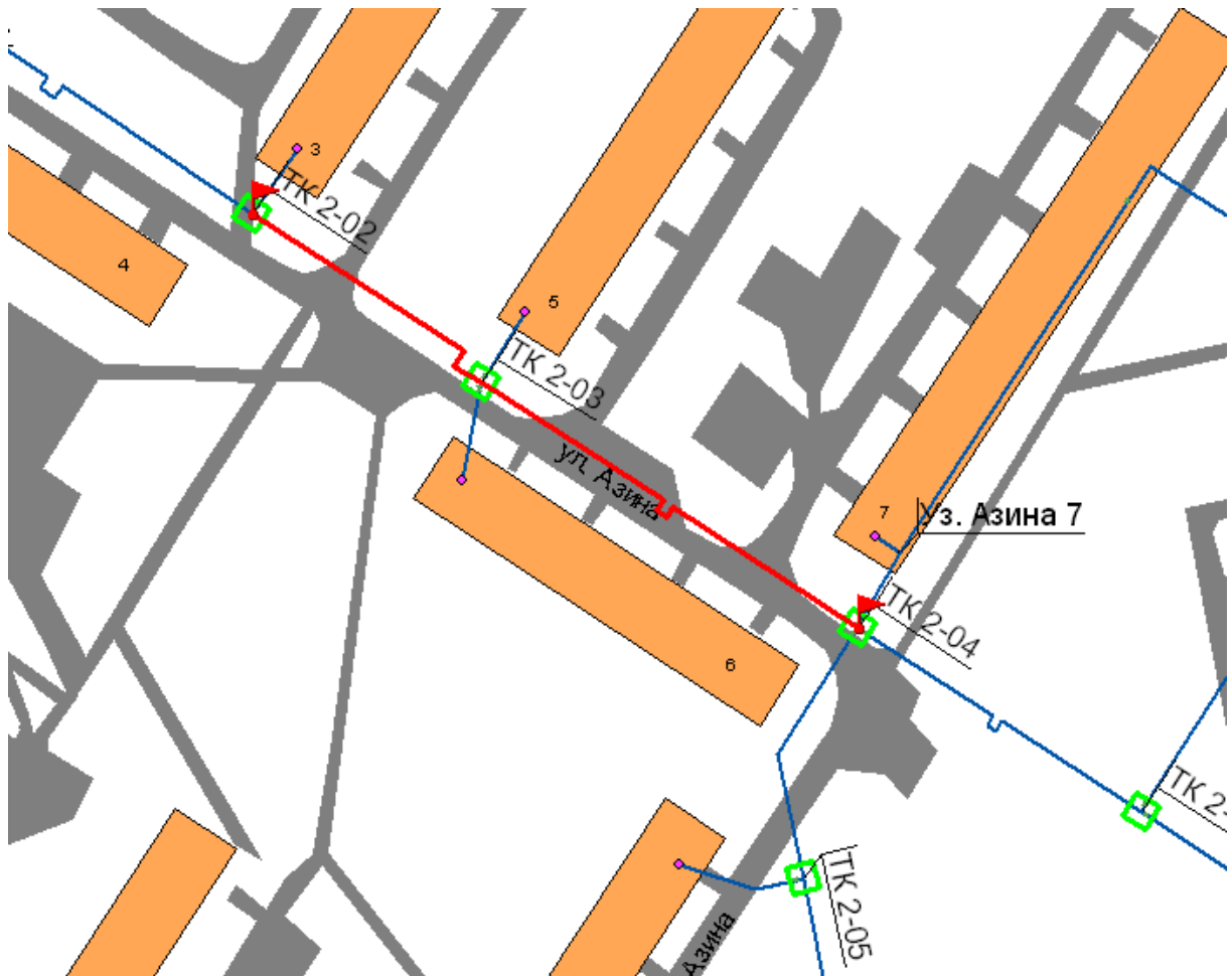
Рис. 4.11. Участок тепломагистрали отTK2-02 до ТК2-04
