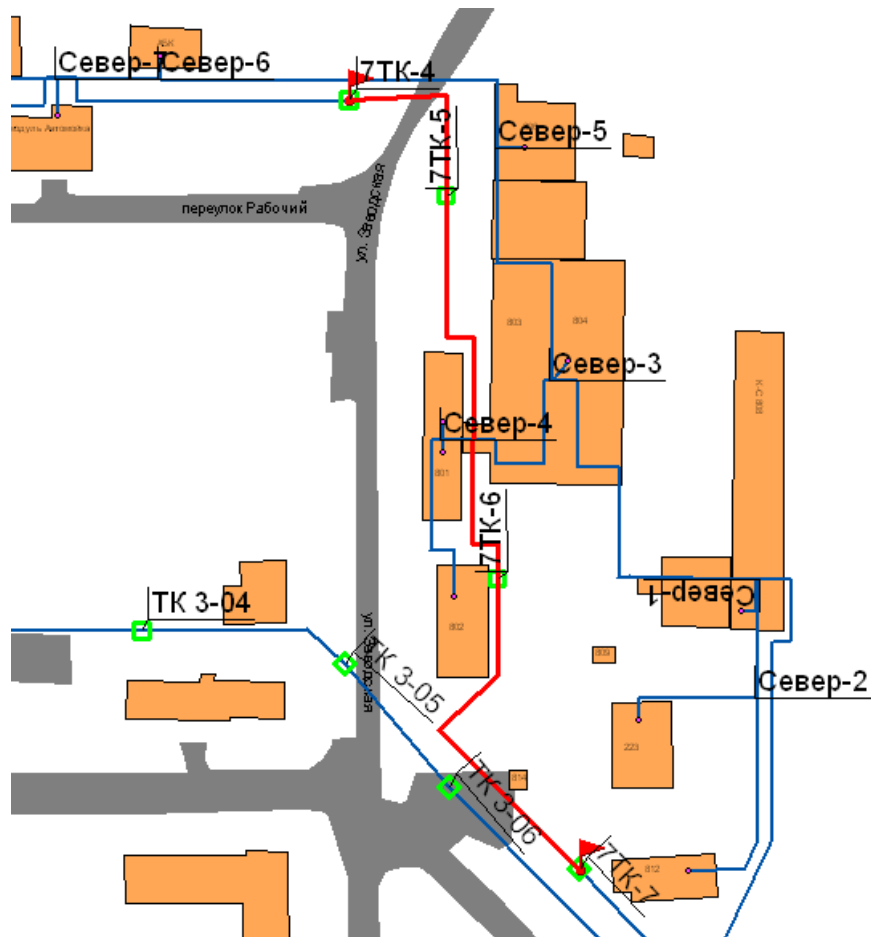
Рис. 4.1. Участок тепломагистрали \varnothing 700 подземный по территории предприятия «Север»
