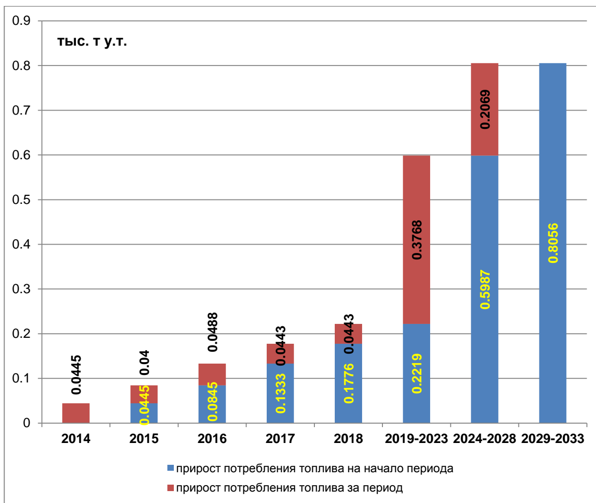
Рис. 2.8.2. Прогнозируемый прирост расхода природного газа для обеспечения теплоснабжения объектов ИЖС в зоне нового строительства № 8 в период 2015 – 2033 гг.
