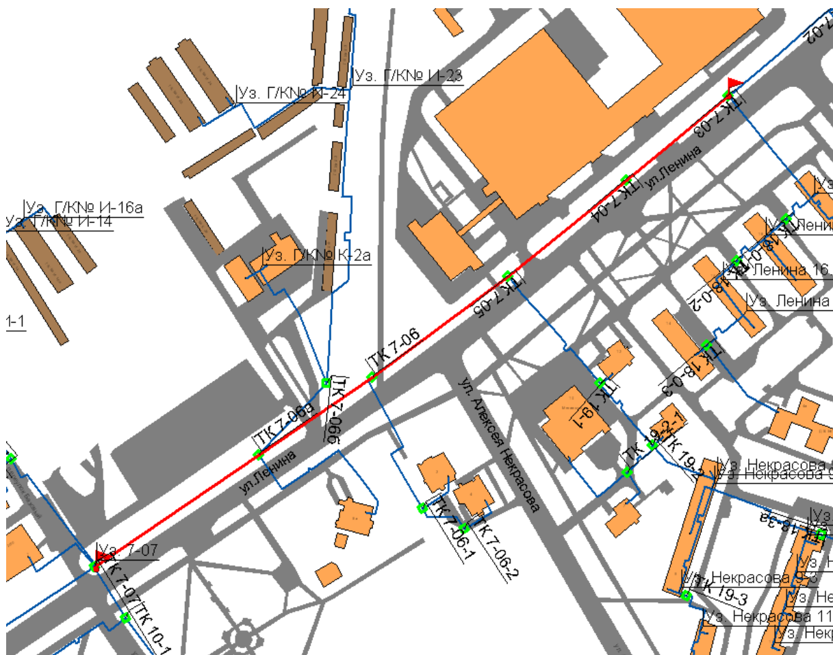
Рис. 4.2. Участок тепломагистрали \varnothing 700 от ТК7-03 до ТК7-07
