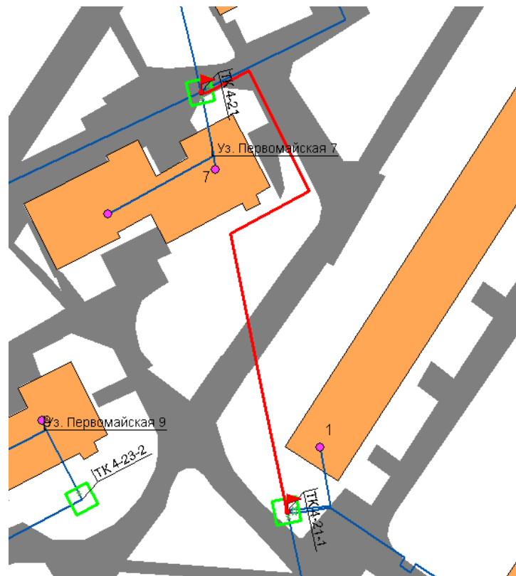
Рис. 4.27. Участок сети от TK4-21 до TK421-1
