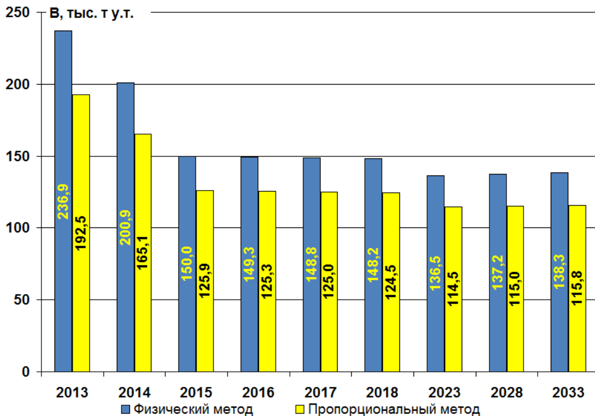
Рис.1.4.9. Перспективный суммарный расход условного топлива на отпуск тепловой энергии по Кировской ТЭС-3 (существующее оборудование)
