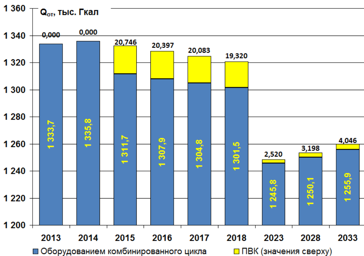
Рис. 1.3.18. Прогноз на 2014 - 2033 годы отпуски Кировской ТЭЦ-3 тепловой энергии в целом (включая отпуск с паром) внешним потребителям (ТЭЦ в целом)
