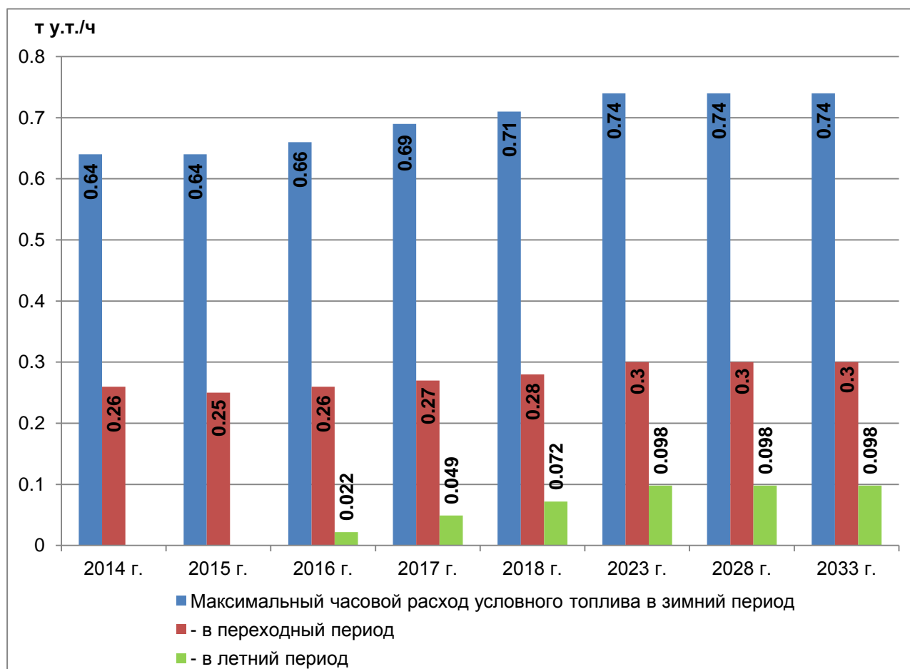
Рис. 3.2.1. Перспективные максимальные часовые расходы условного топлива на котельной микрорайона Каринторф на период 2014 – 2033 гг.
