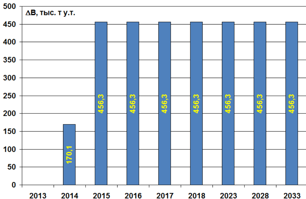
Рис.1.4.2. Прогноз на 2014 - 2033 годы изменения расхода условного топлива Кировской ТЭЦ-3 от состояния на 2013 год (вновь вводимая ПГУ-220Т)
