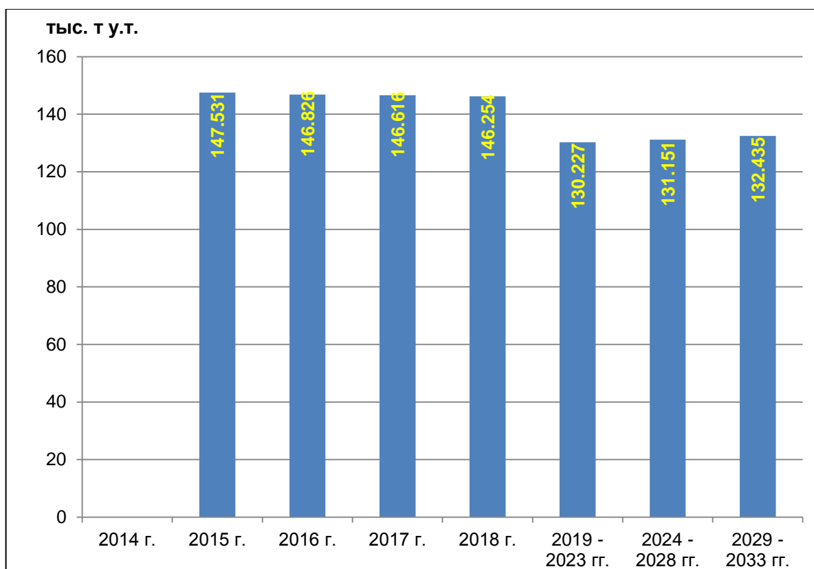
Рис. 1.7.2. Изменение расхода условного топлива по всем источникам тепловой мощности г. Кирова-Чепецка в период 2014 – 2033 гг.
