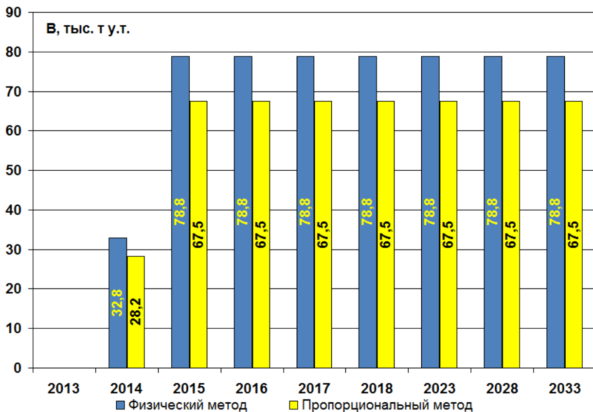
Рис.1.4.10. Перспективный суммарный расход условного топлива на отпуск тепловой энергии по Кировской ТЭС-3 (вновь вводимая ПГУ-220Т)
