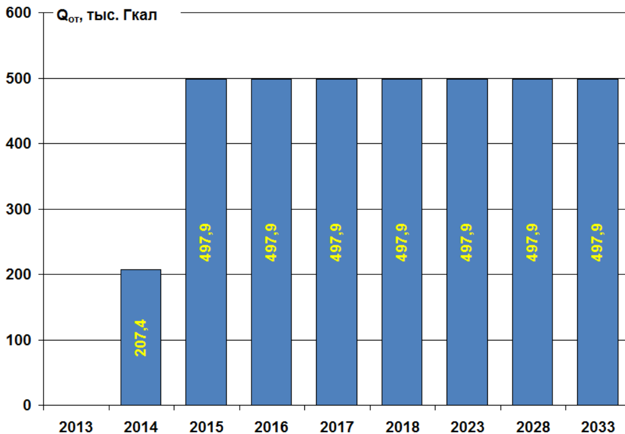
Рис. 1.3.17. Прогноз на 2014 - 2033 годы отпуски Кировской ТЭЦ-3 тепловой энергии в целом внешним потребителям (вновь вводимая ПГУ-220Т)
