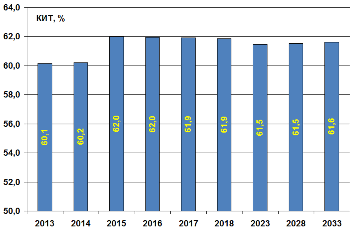
Рис.1.4.14. Прогноз на 2014 - 2033 годы изменения коэффициента использования топлива Кировской ТЭЦ-3 (ТЭЦ в целом)
