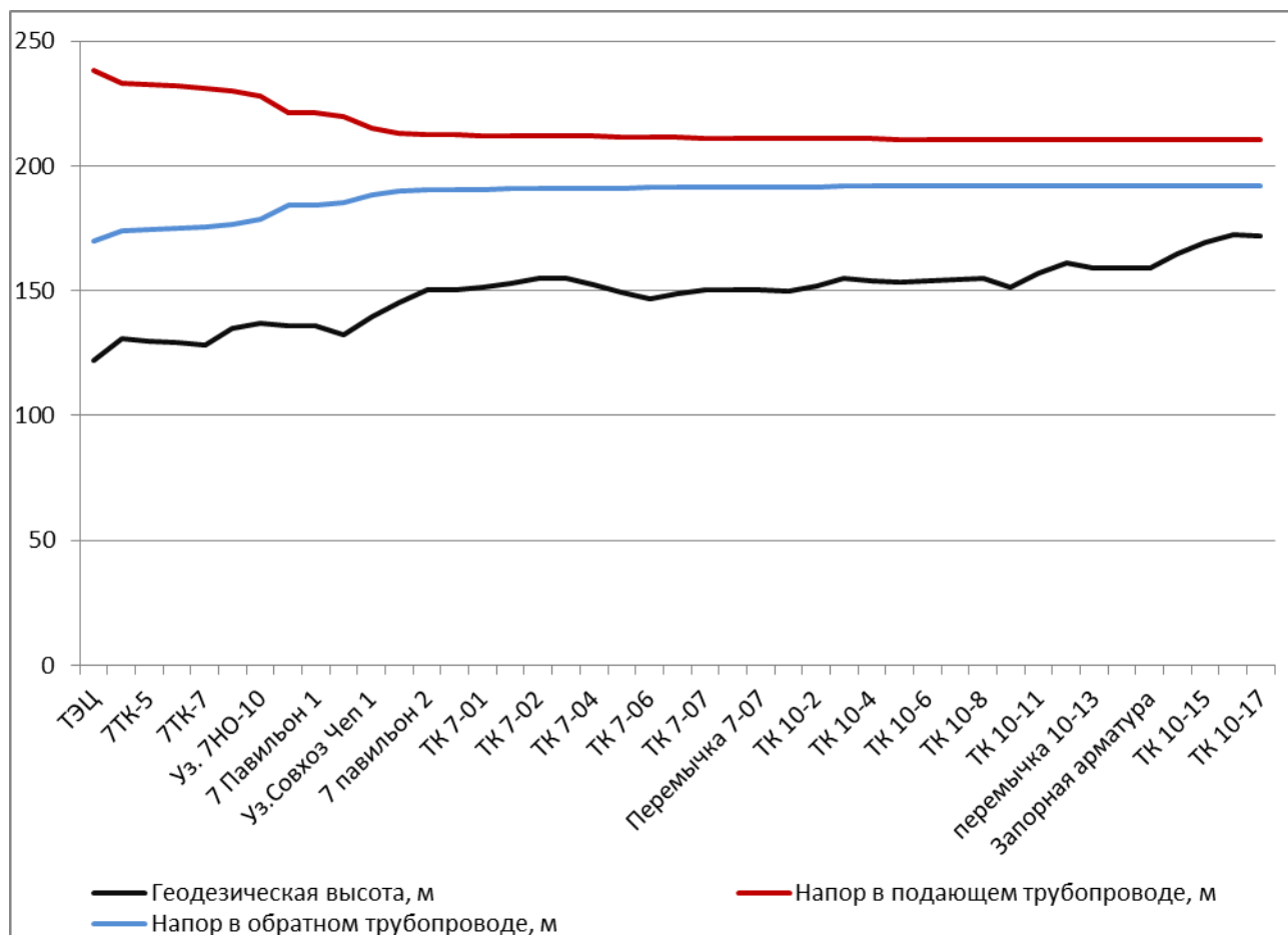
Рис. П 2.3.12. Пьезометрический график работы тепловой сети от ТЭЦ-3 до ул. Победы 11 2017 г.
