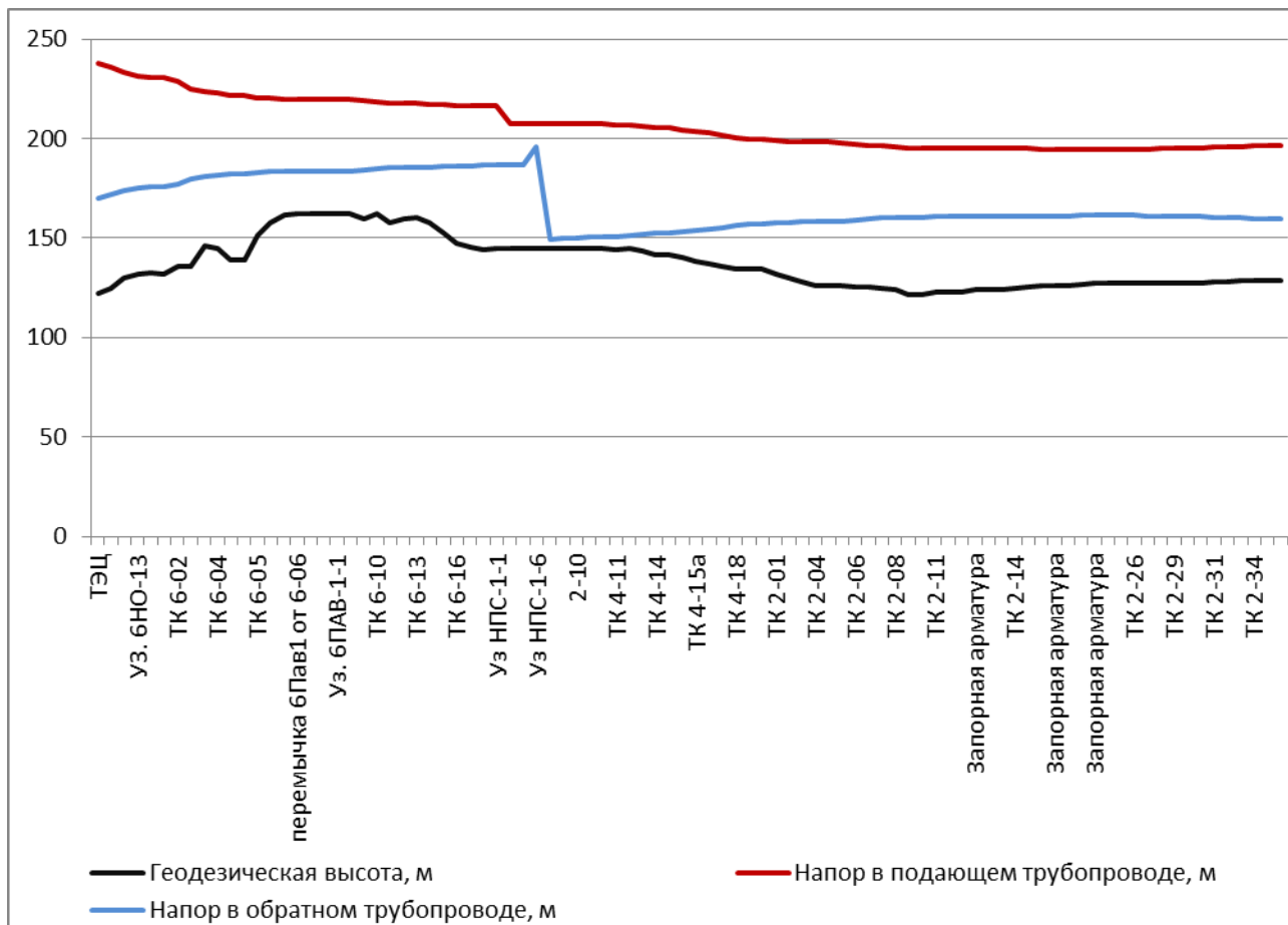
Рис. П 2.4.6. Пьезометрический график работы тепловой сети от ТЭЦ-3 до ТК 4-32 (через Черемушки) в 2018 г.
