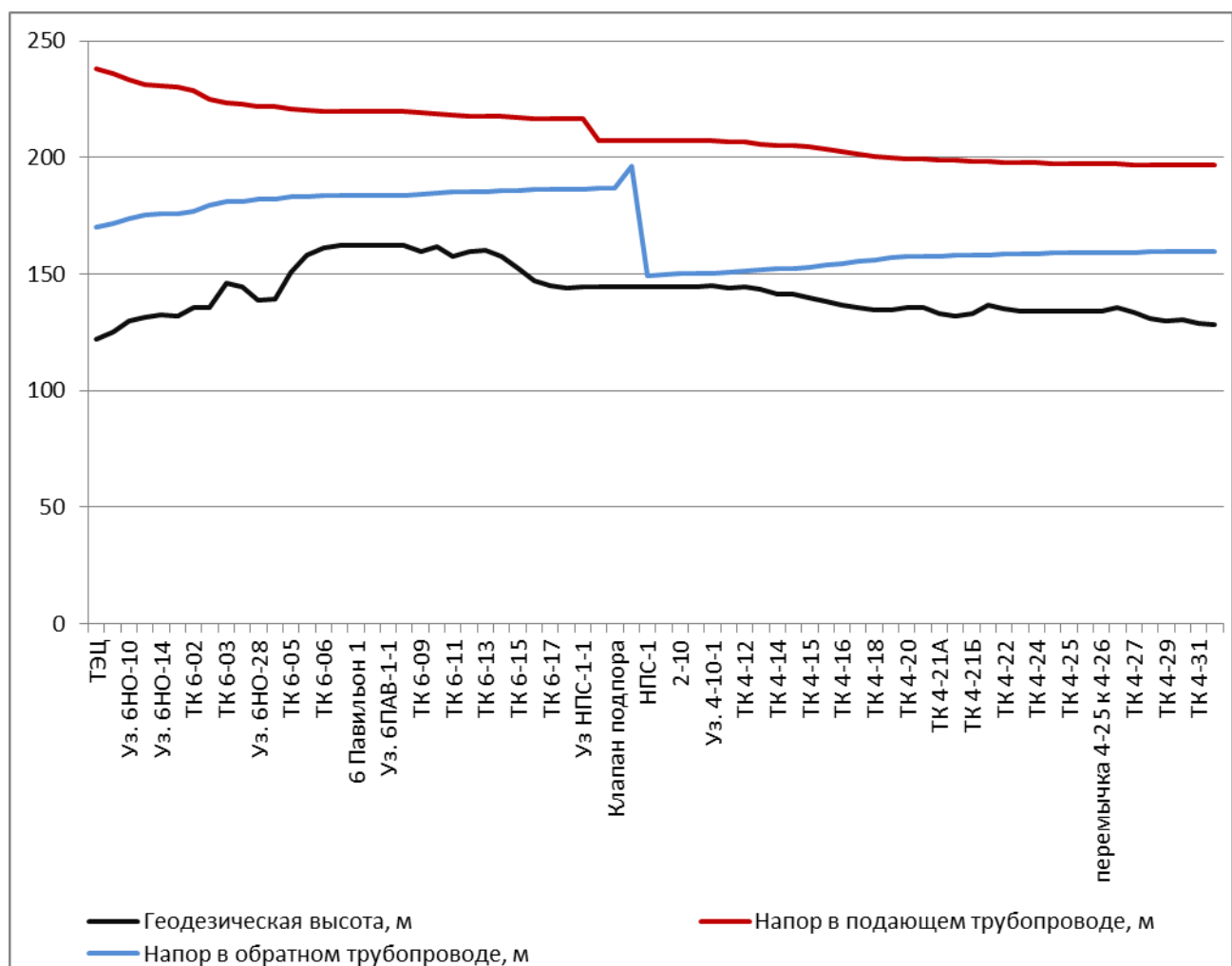
Рис. П 2.1.8. Пьезометрический график работы тепловой сети от ТЭЦ-3 до ТК 4-32 2015 г.
