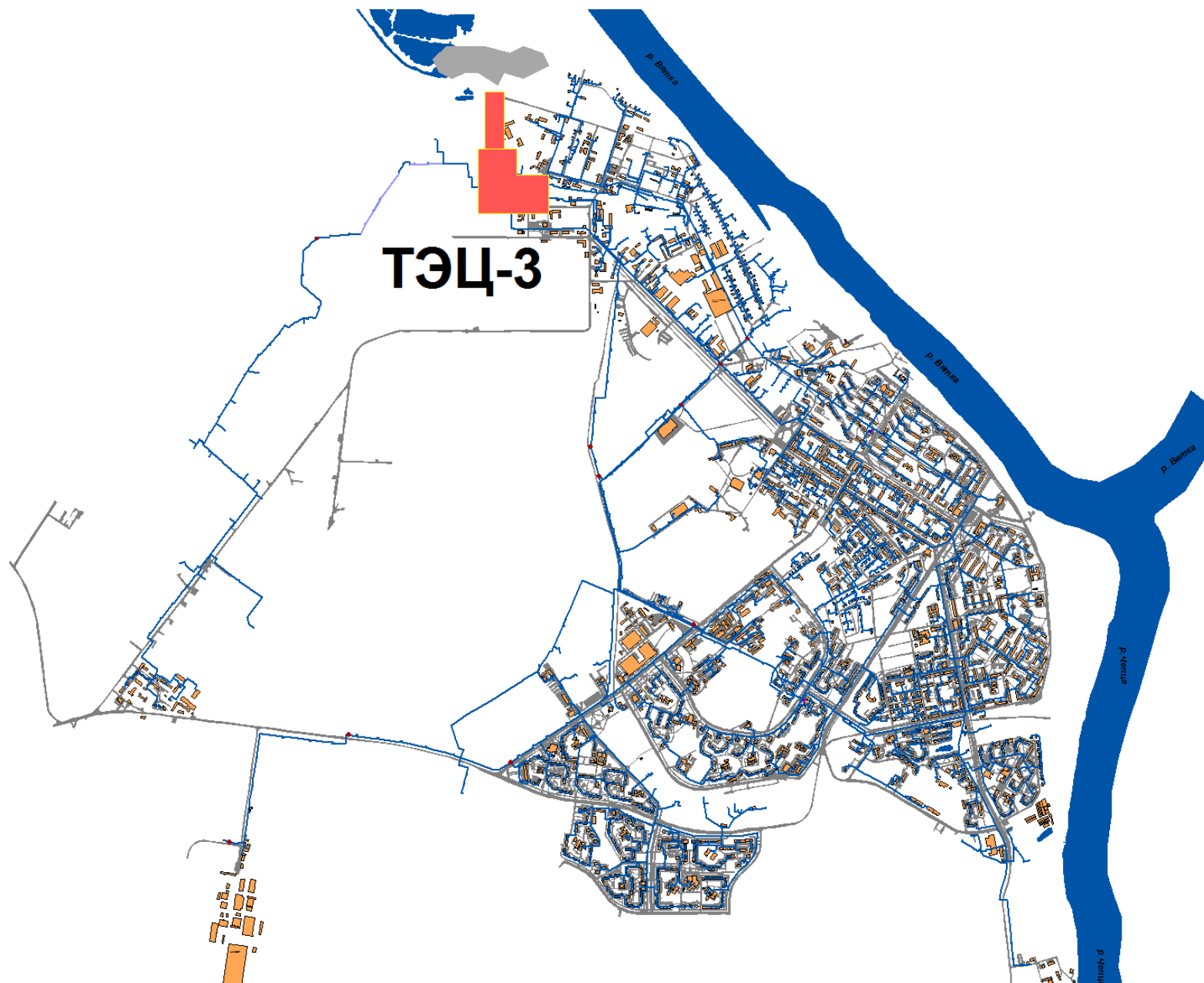
Рис. 1.1.1. Схема расположения источников теплоснабжения в г. КирОВО-Чепецк
