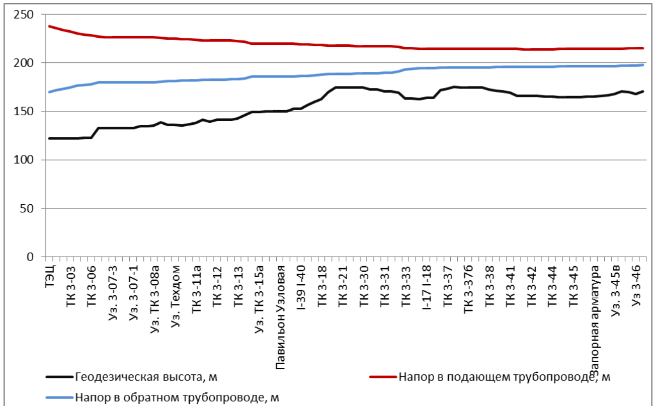
Рис. П 2.5.4. Пьезометрический график работы тепловой сети от ТЭЦ-3 до Уз. 3-47 в 2019-2023 гг.
