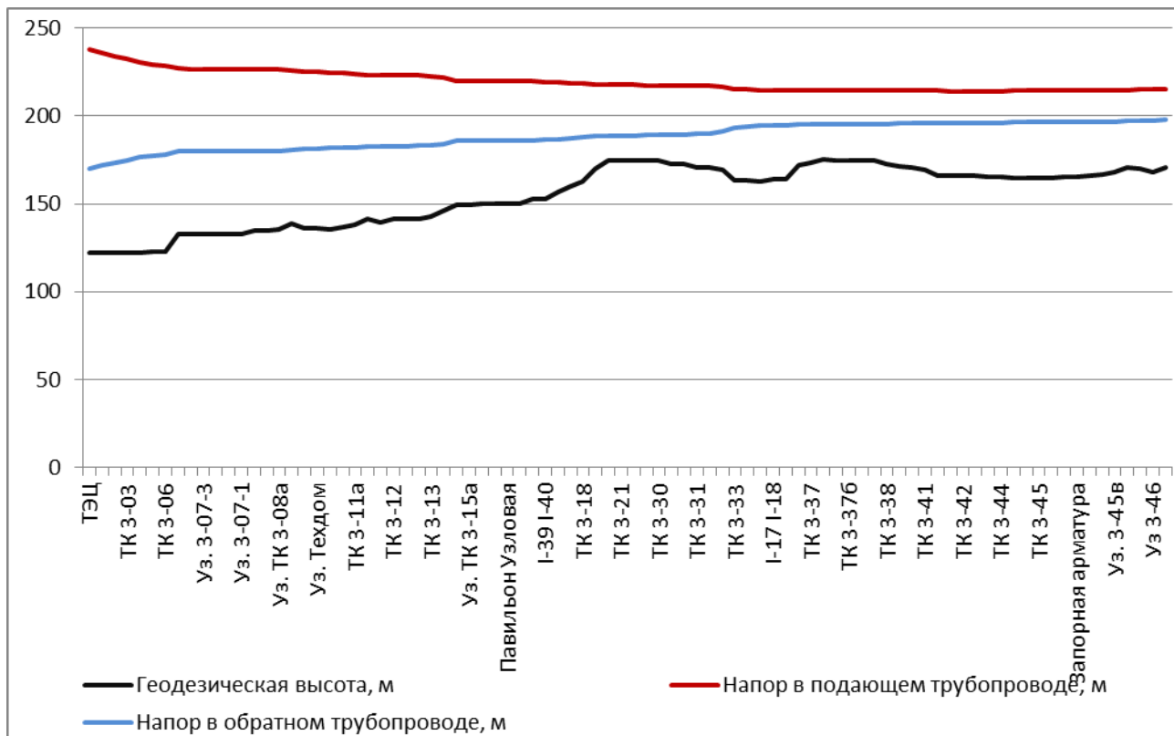
Рис. П 2.4.4. Пьезометрический график работы тепловой сети от ТЭС-3 до Уз. 3-47 в 2018 г.
