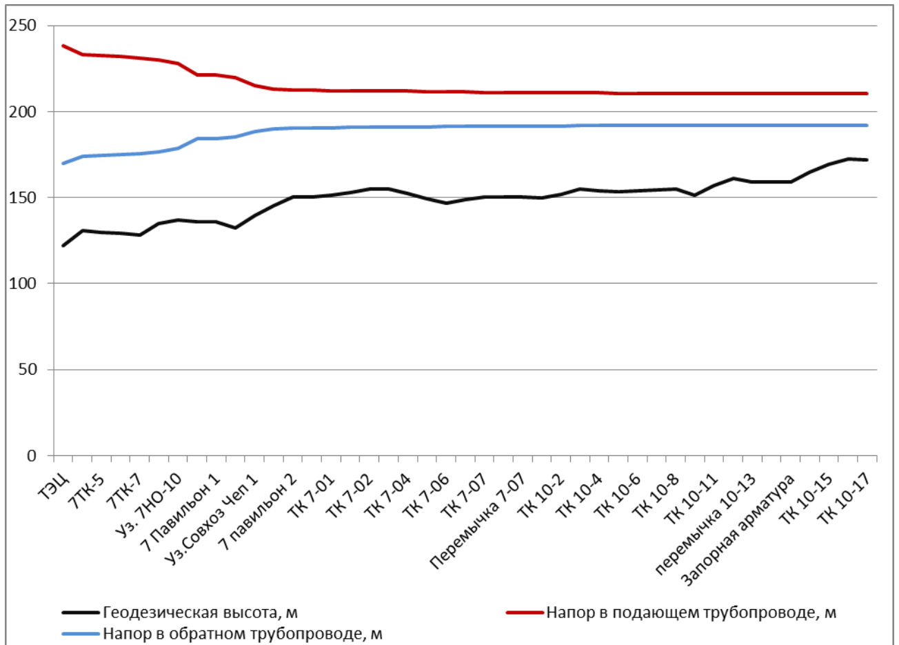
Рис. П 2.4.12. Пьезометрический график работы тепловой сети от ТЭЦ-3 до ул. Победы 11 2018 г.
