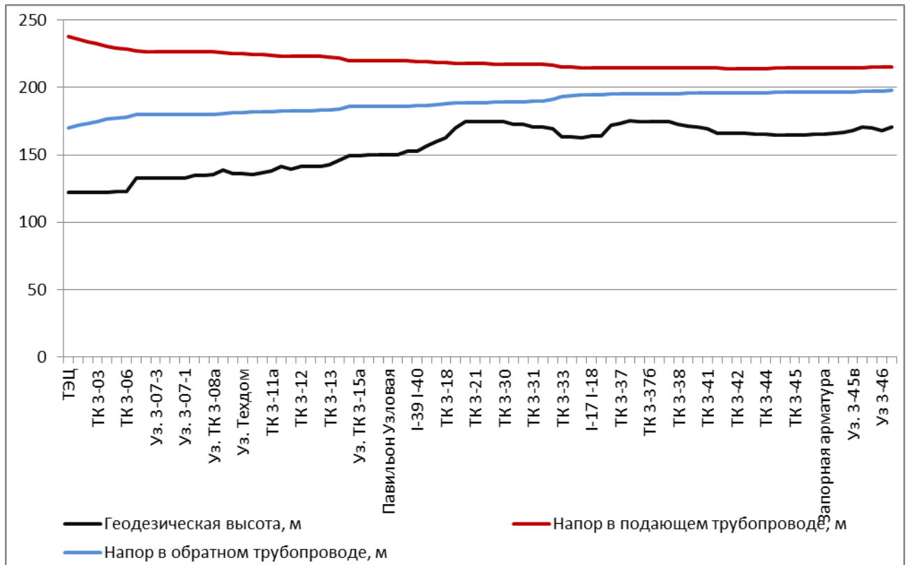
Рис. 2.3.4. Пьезометрический график работы тепловой сети от ТЭЦ-3 до Уз. 3-47 в 2033 гг.
