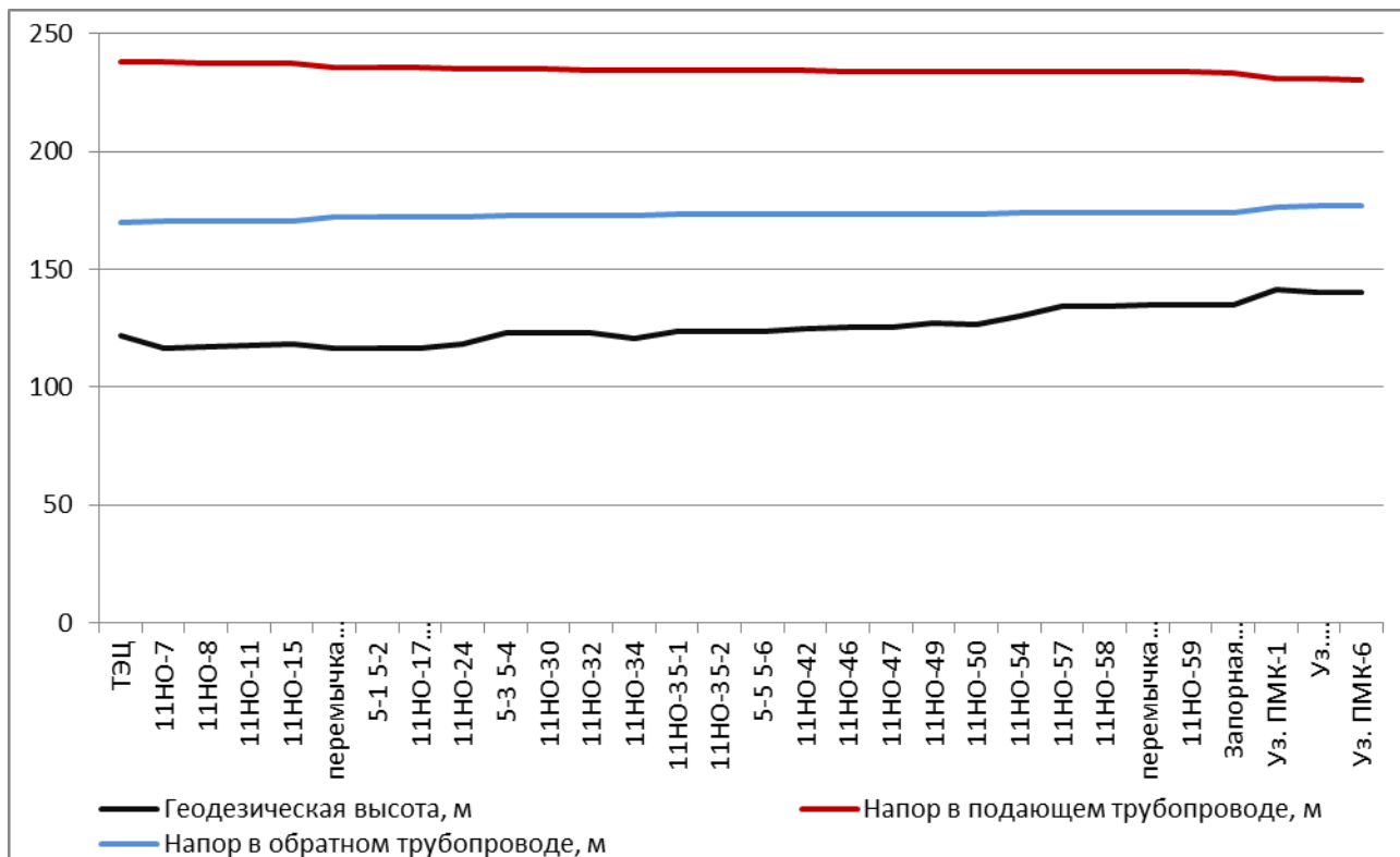
Рис. 2.3.2. Пьезометрический график работы тепловой сети от ТЭЦ-3 до Уз. ПМК-6 в 2033 гг.
