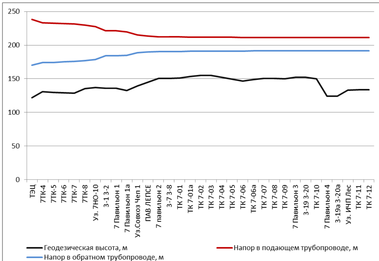
Рис. П 2.4.10. Пьезометрический график работы тепловой сети от ТЭС-3 до ТК 7-12 2018 г.
