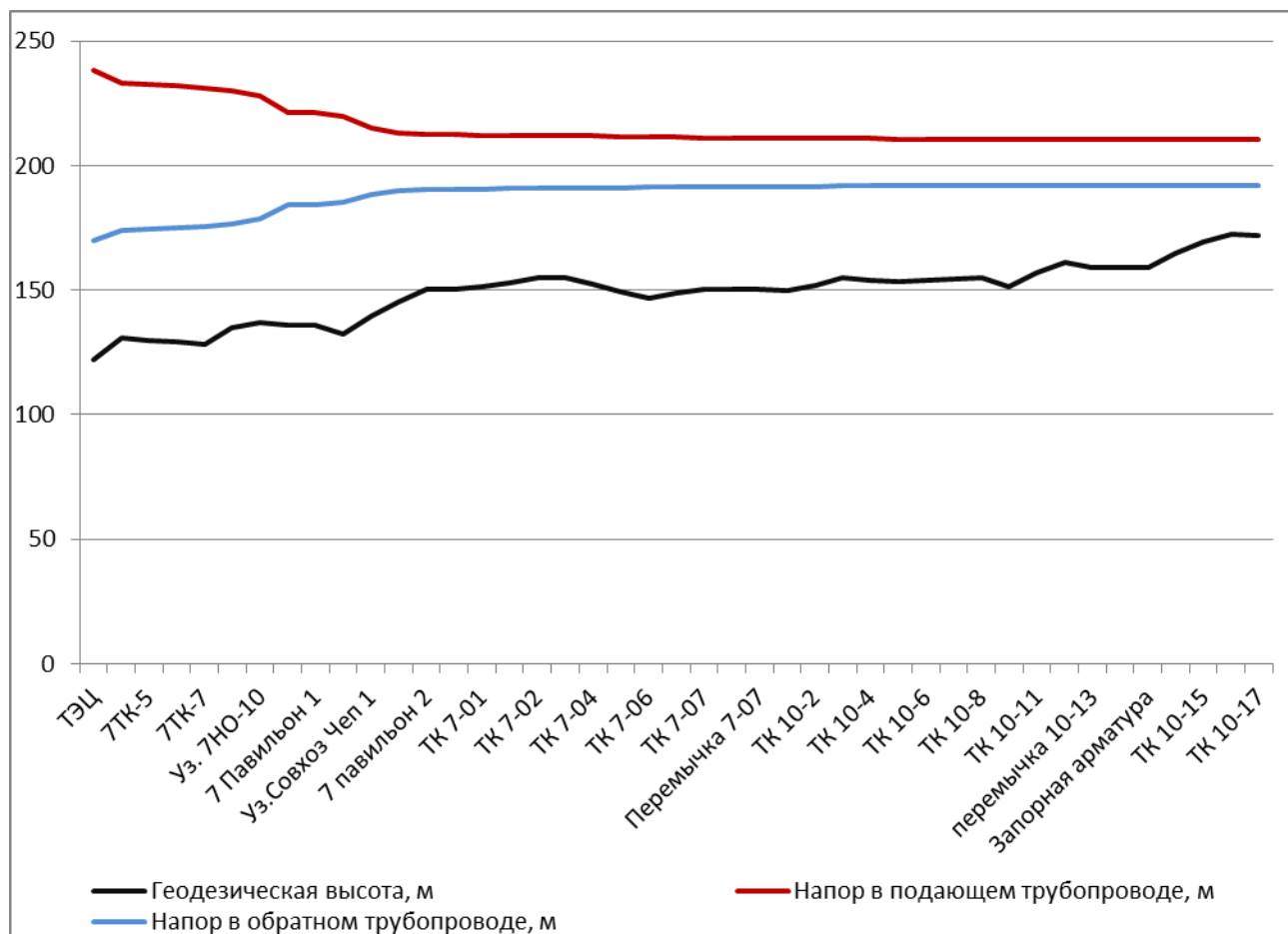
Рис. 2.3.12. Пьезометрический график работы тепловой сети от ТЭЦ-3 до ул. Победы 11 2033 г.
