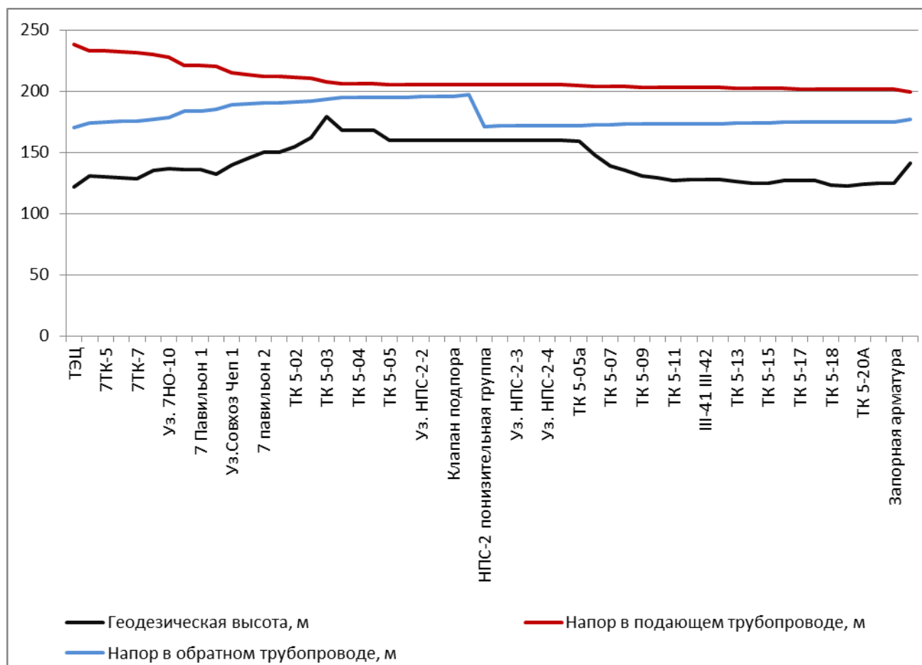
Рис. П 2.6.14. Пьезометрический график работы тепловой сети от ТЭЦ-3 до ТК 5-22 в 2024-2028 гг.
