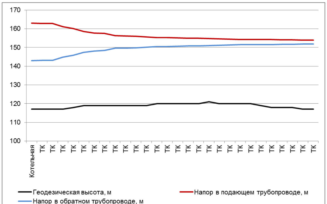
Рис. 2.2.16. Пьезометрический график работы тепловой сети от котельной мкр. Каринторф в 2013 г.
