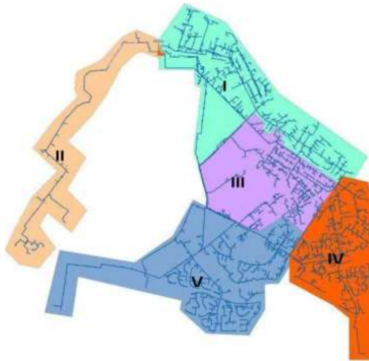
Рисунок 2.2 – Расчетная схема определения радиуса теплоснабжения Кировской ТЭЦ-3
