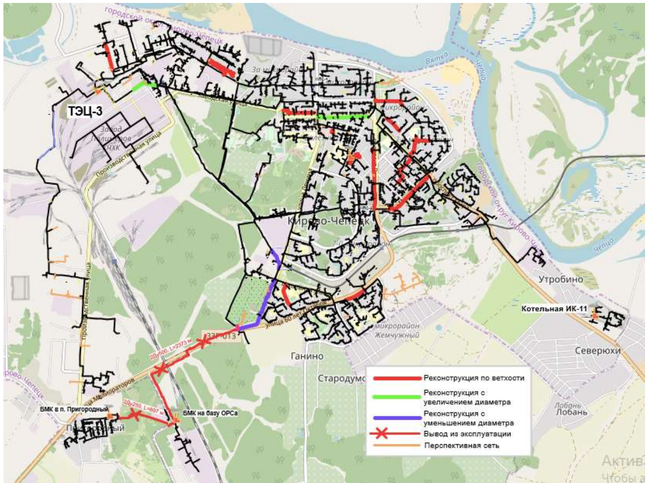
Рисунок 6.12 – Реконструкция по ветвисти тепловых сетей от ТЭЦ-3
