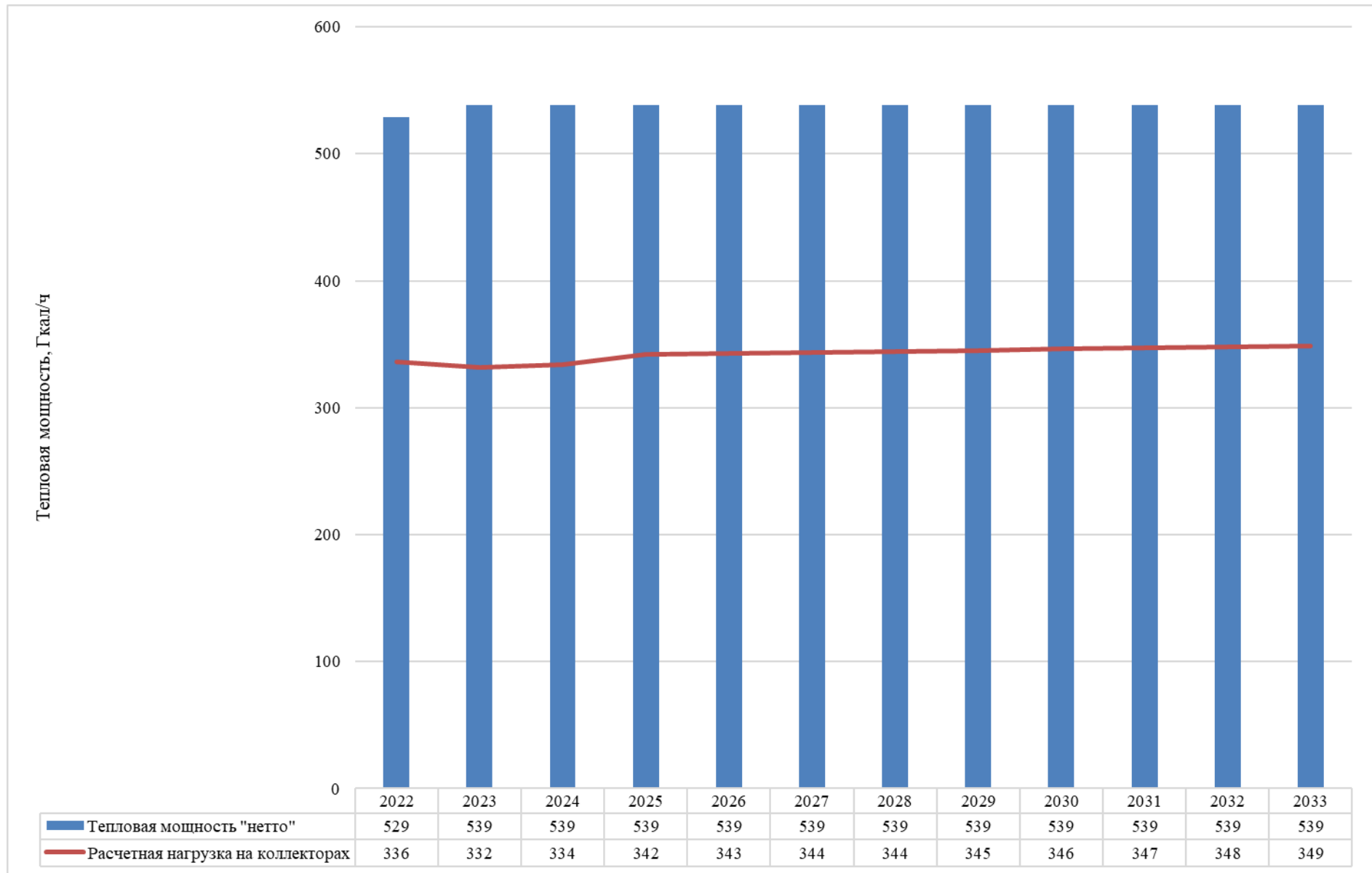
Рисунок 5.1 - Баланс тепловой мощности и подключенной нагрузки Кировской ТЭЦ-3 на расчетный период
