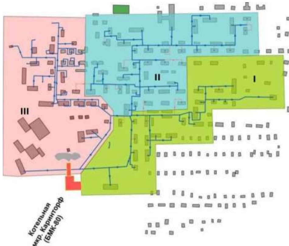
Рисунок 2.4 – Расчетная схема МКР Каринторф
