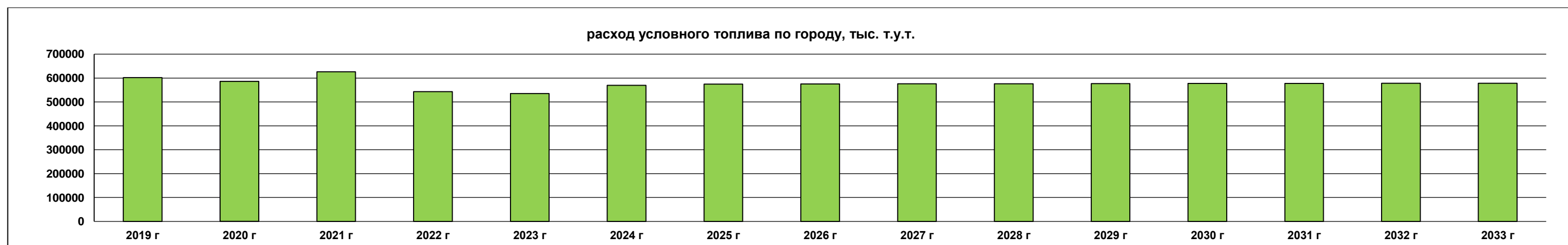
Рисунок 10.1. Перспективный расход условного топлива по г. Кирово-Чепецк
