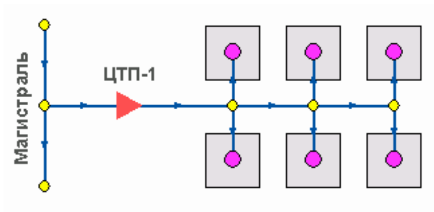
Рисунок 3.4 – Изображение ЦТП
