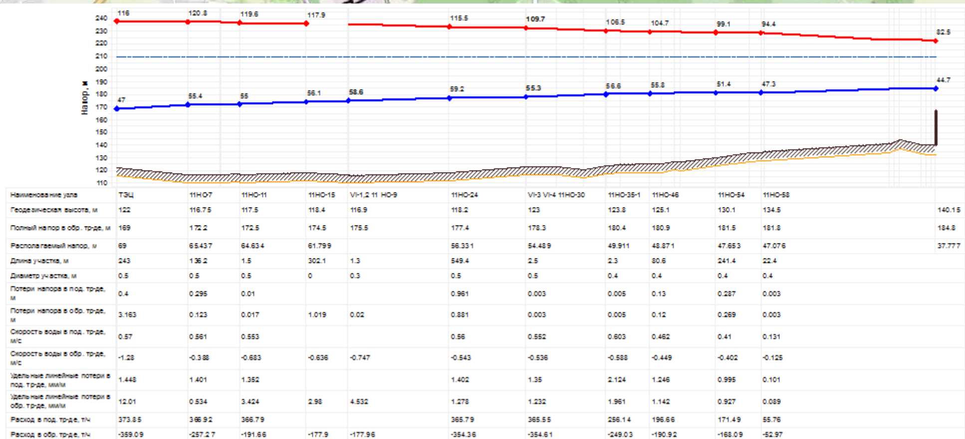
Рисунок 5.5 – Пьезометрический фактического гидравлического режима ТЭЦ-3 – ул. Мелиораторов, 28/1 (магистраль БСИ)
