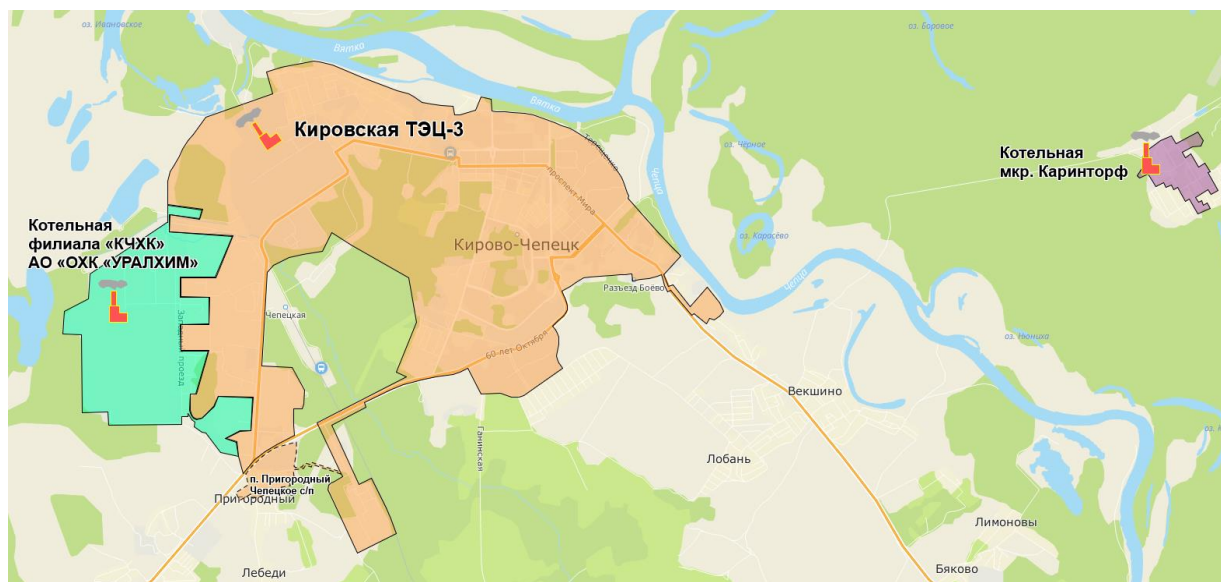
Рисунок 2.1. Схема расположения источников теплоснабжения в г. Кирово-Чепецк
