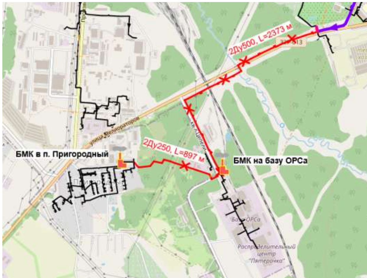
Рисунок 5.6 – Вывод из эксплуатации магистралей на базу ОРСа и п. Пригородный
