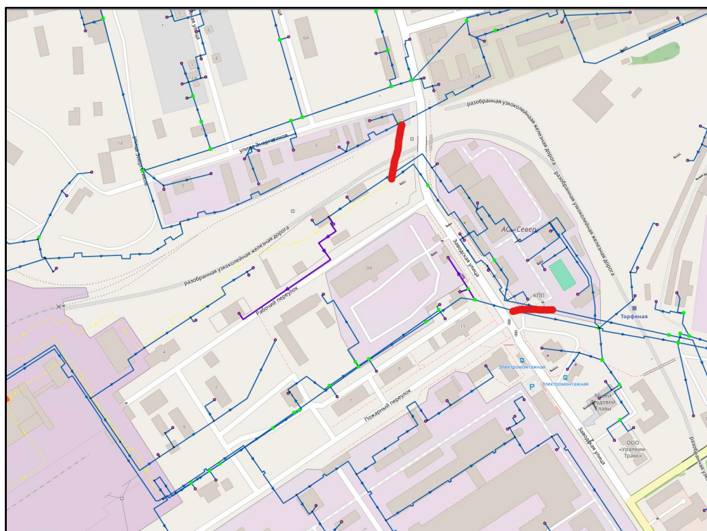
Рисунок 11.8. Строительство дополнительных перемычек для компенсации отключенного головного участка Ду 700 мм
