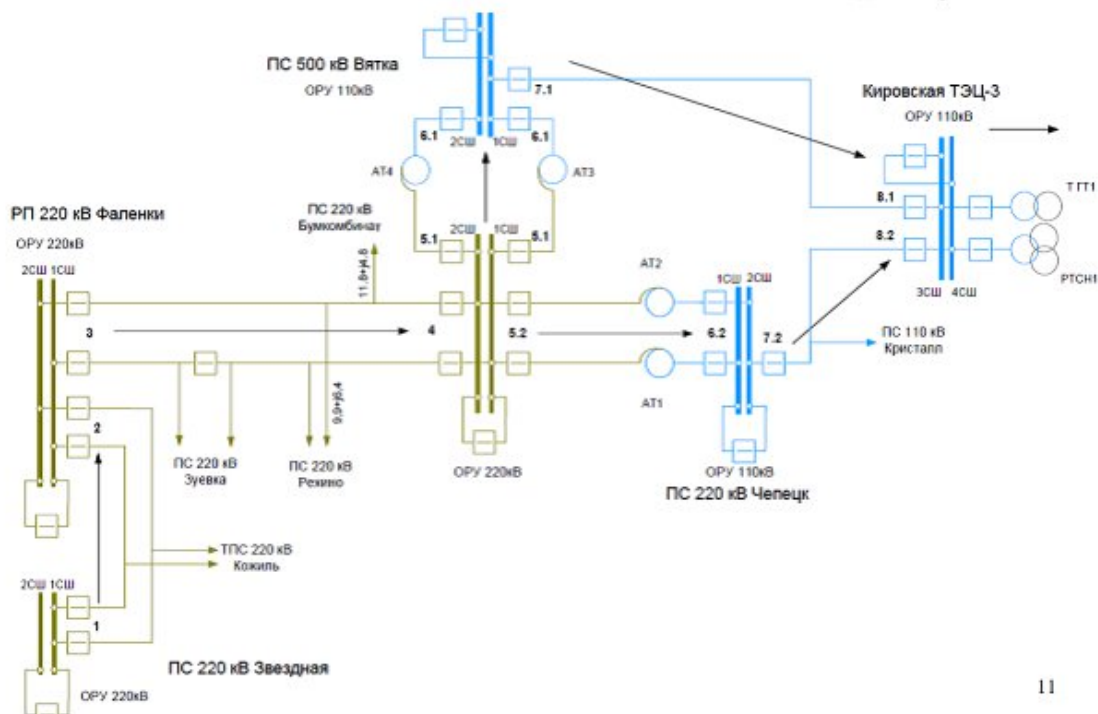
Рисунок 11.3. Схема подачи напряжения №1 на шины 110 кВ Кировской ТЭЦ-3
