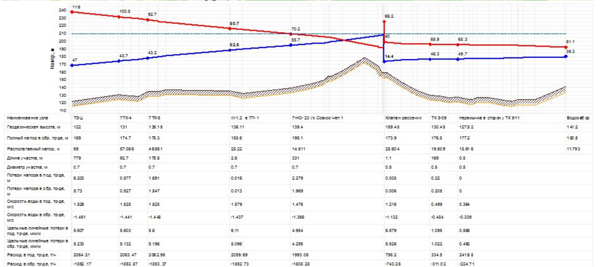
Рисунок 5.2 – Пьезометрический график гидравлического режима ТЭЦ-3 – Водоразбор (магистраль Ду700)
