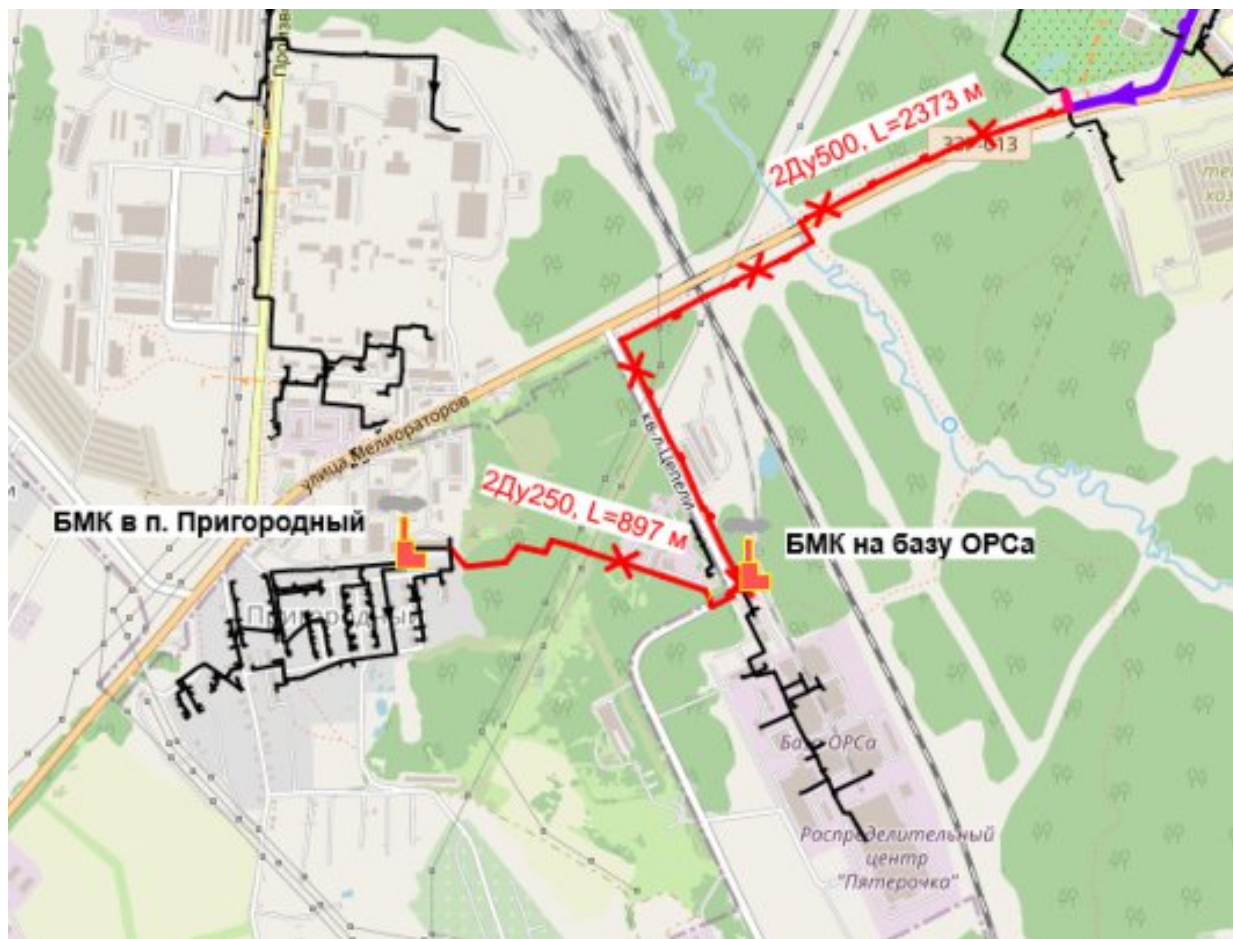
Рисунок 5.6 – Вывод из эксплуатации магистралей на базу ОРСа и п. Пригородный
