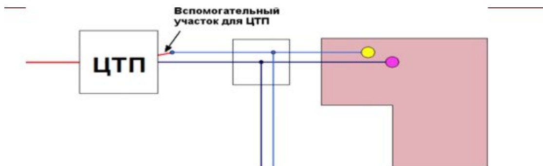
Рисунок 3.5 – Подключение трубопровода ГВС
