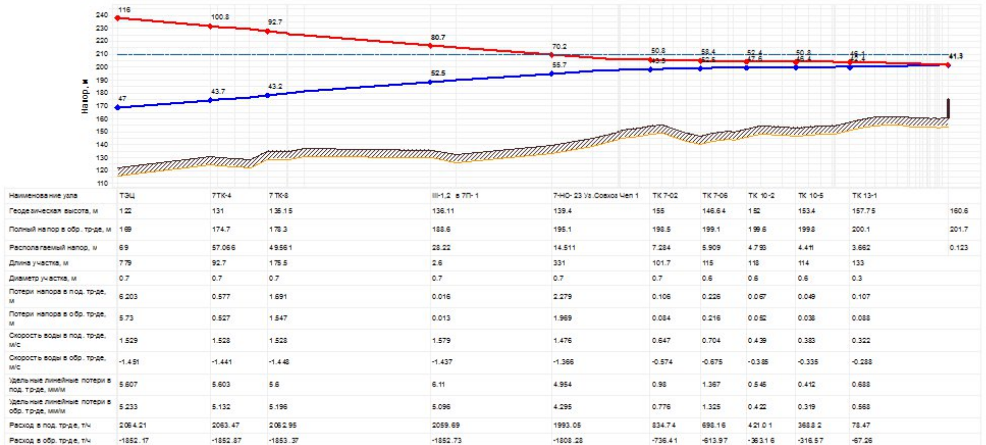
Рисунок 5.3 – Пьезометрический график гидравлического режима ТЭЦ-3 – ул. Юбилейная, 15 (магистраль Ду700)
