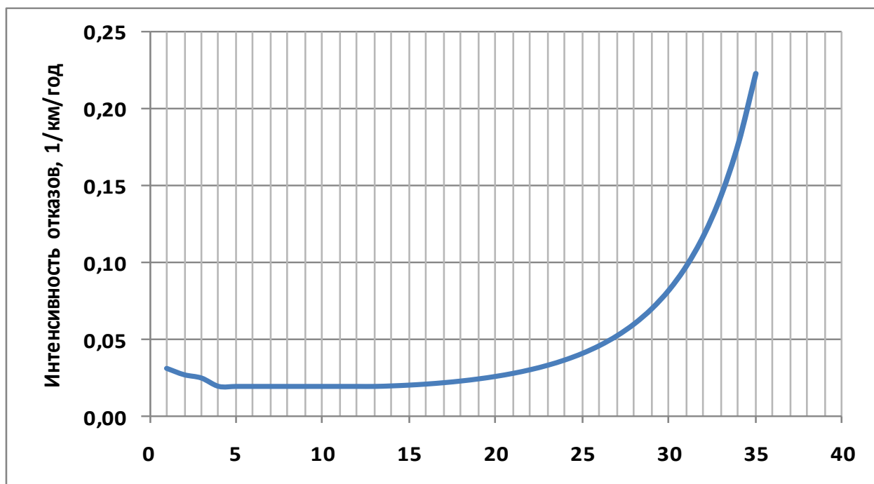
Рисунок 11.2. Интенсивность отказов в зависимости от срока эксплуатации участка тепловой сети
