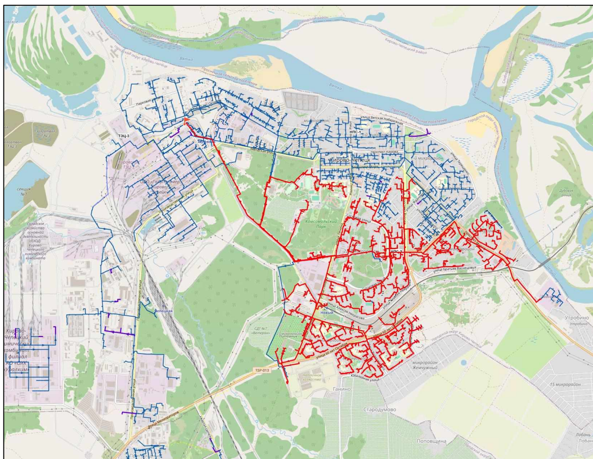
Рисунок 11.6. Зона действия вывода тепловой мощности, с наибольшим диаметром, от ТЭЦ-3 с диаметром головного участка Ду-700 мм
