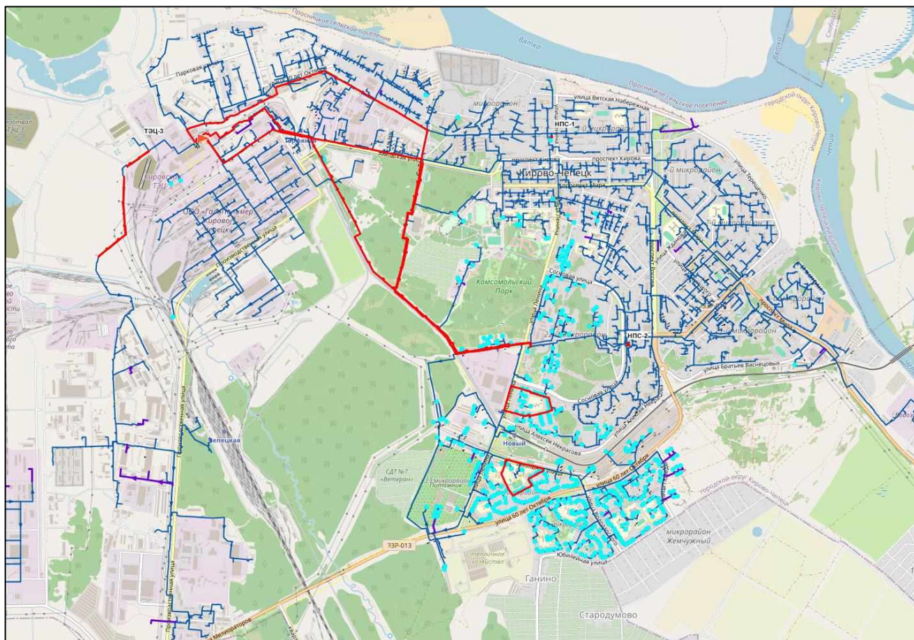
Рисунок 11.7. Потребители с температурой воздуха внутри помещения менее 12 °С при отключении головного участка с наибольшим диаметром и схема размещения колец
