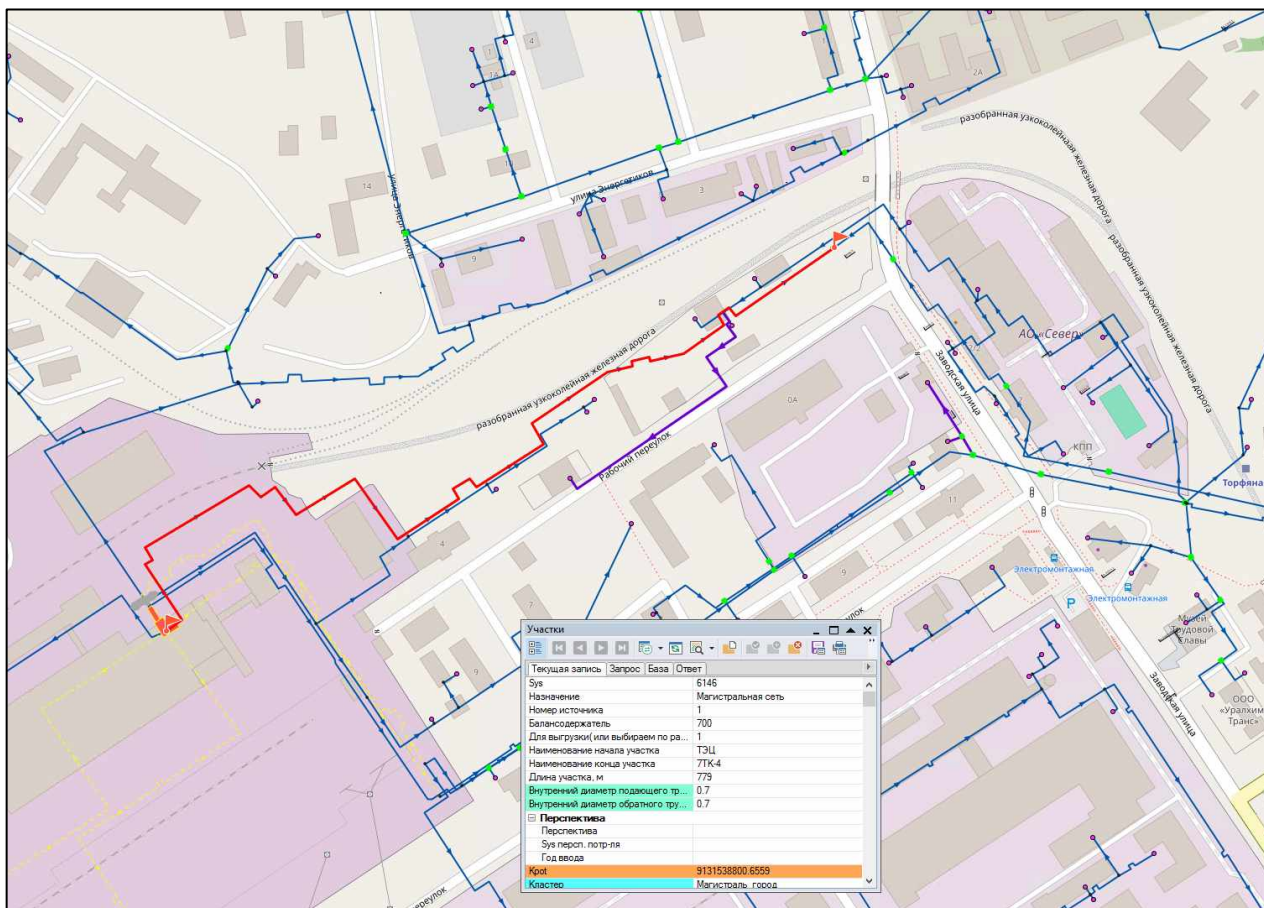
Рисунок 11.11. Головной участок наибольшего диаметра для которого необходимо предусмотреть резервирование
