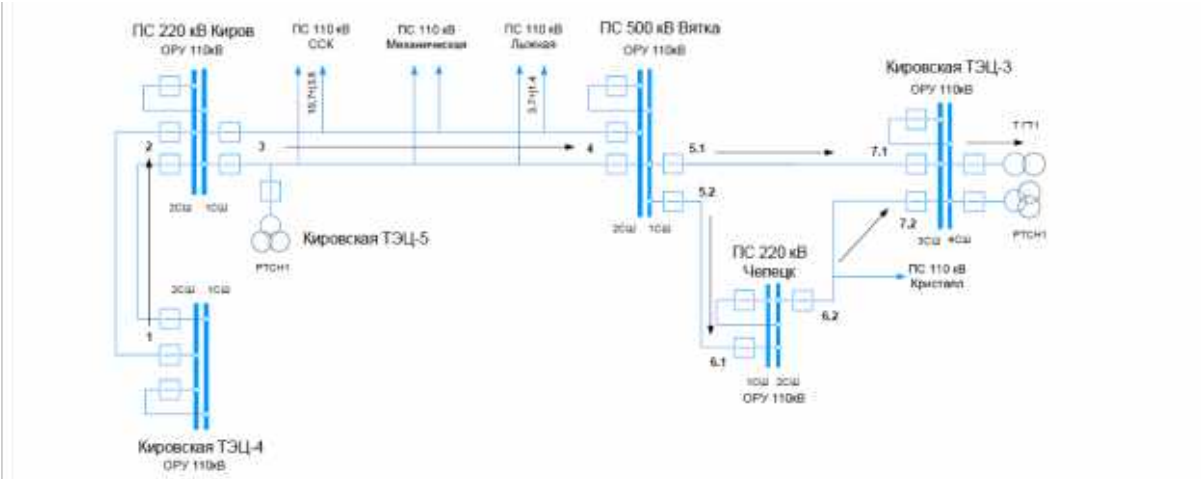
Рисунок 11.5. Схема подачи напряжения №2 на шины 110 кВ Кировской ТЭЦ-3
