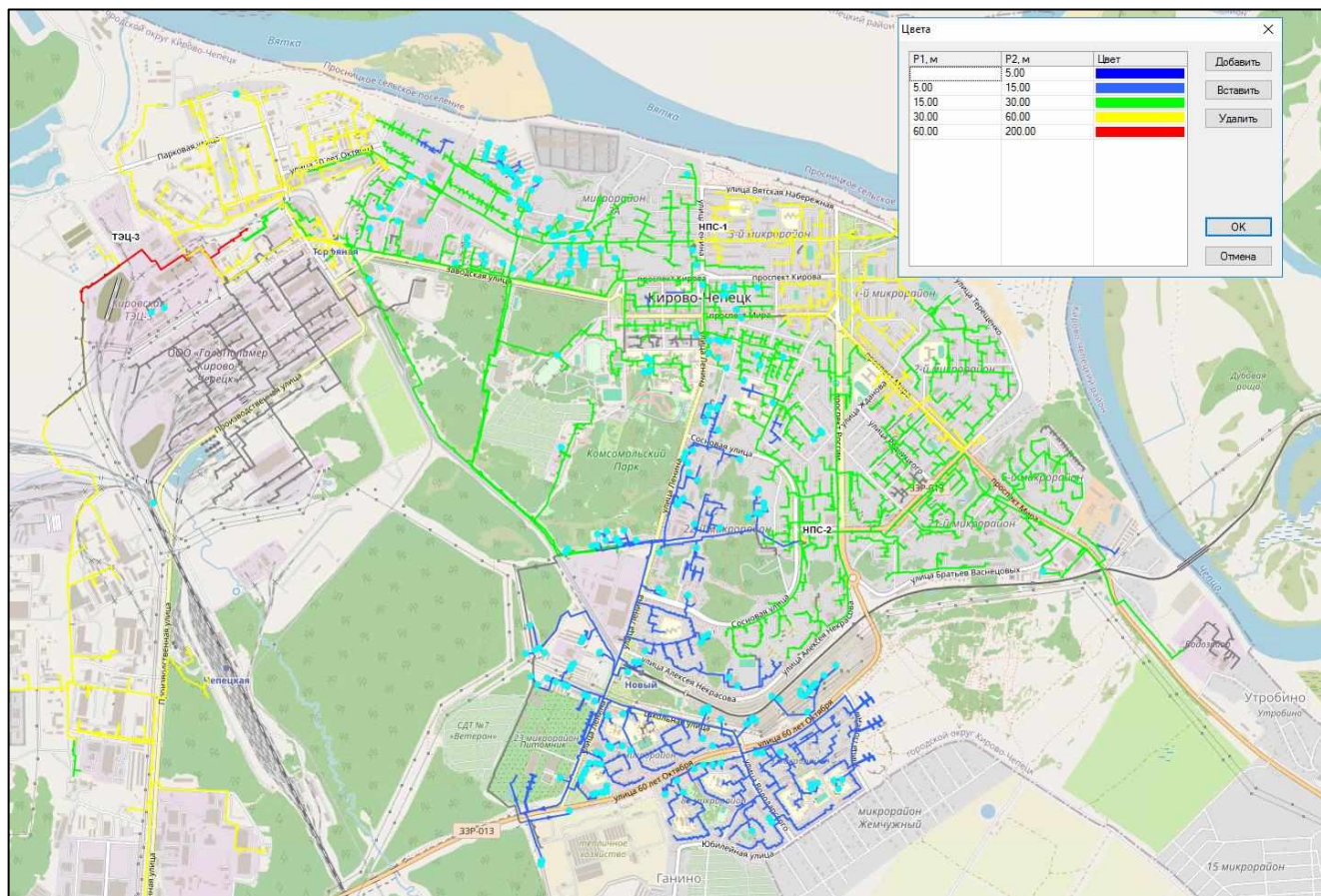
Рисунок 11.10. Потребители с температурой воздуха внутри помещения менее 12 °С при строительстве дополнительных перемычек для компенсации отключенного головного участка
