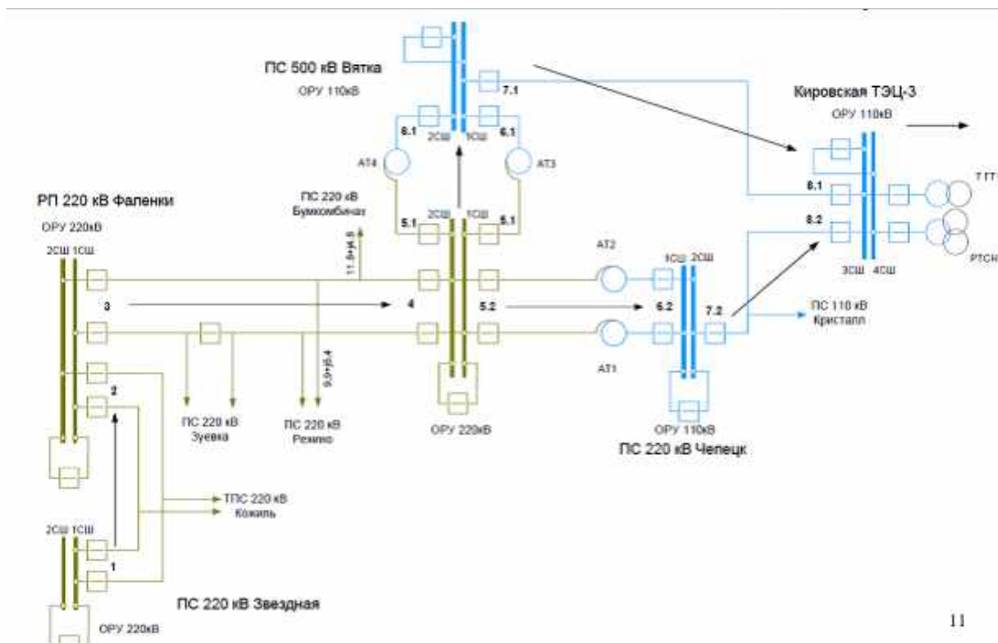
Рисунок 11.4. Схема подачи напряжения №1 на шины 110 кВ Кировской ТЭЦ-3
