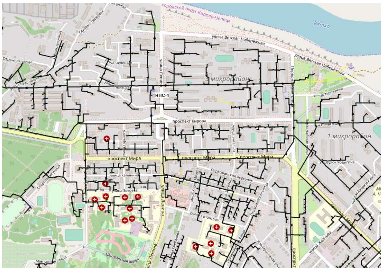
Рисунок 26 – Фрагмент схемы тепловых сетей
