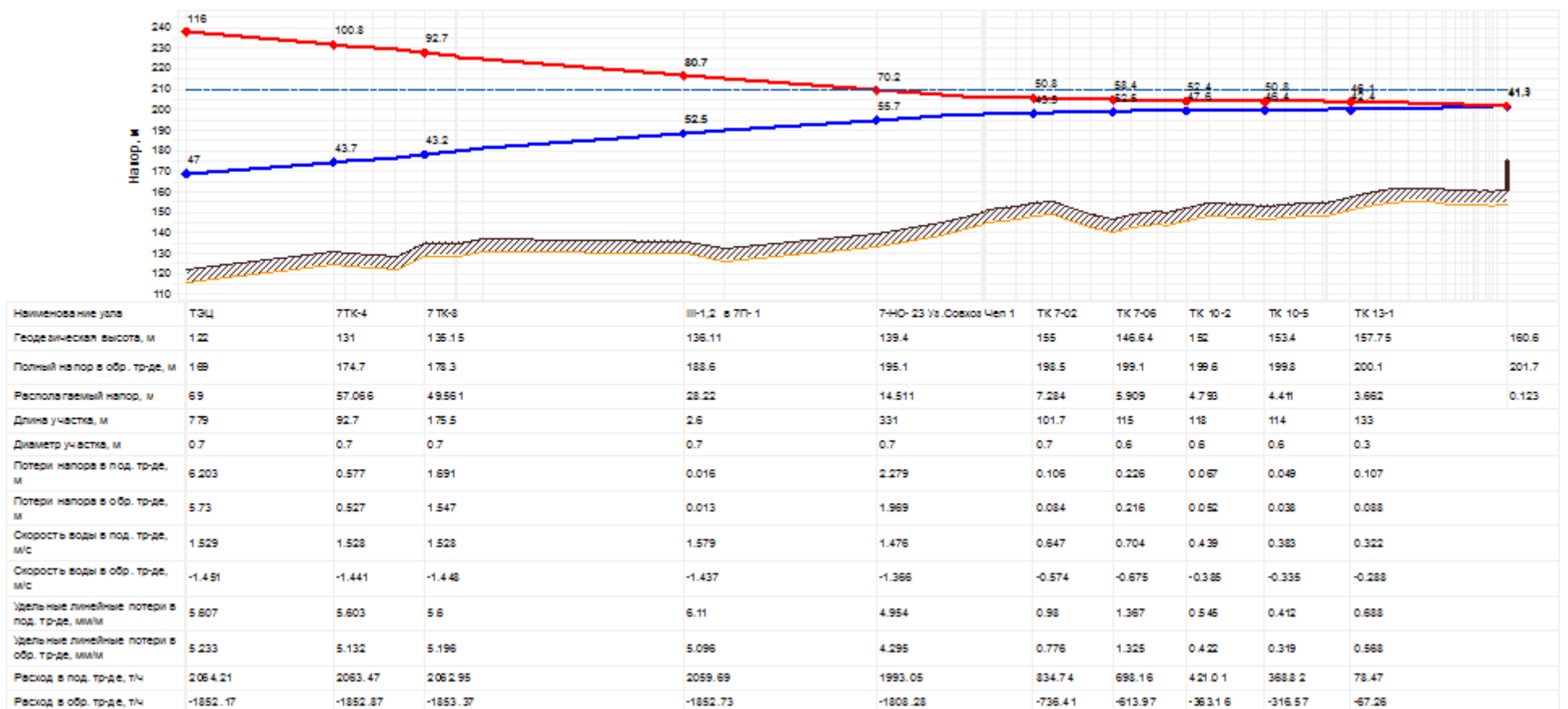
Рисунок 29 – Пьезометрический график фактического гидравлического режима ТЭЦ-3 – ул. Юбилейная, 15 (магистраль Ду700)
