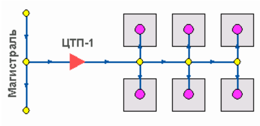
Рисунок 4 – Изображение ЦТП
