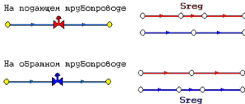
Рисунок 17 – Дросселирующие устройства
