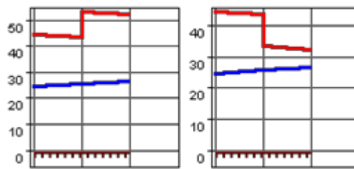
Рисунок 15 – Пьезометрические графики
