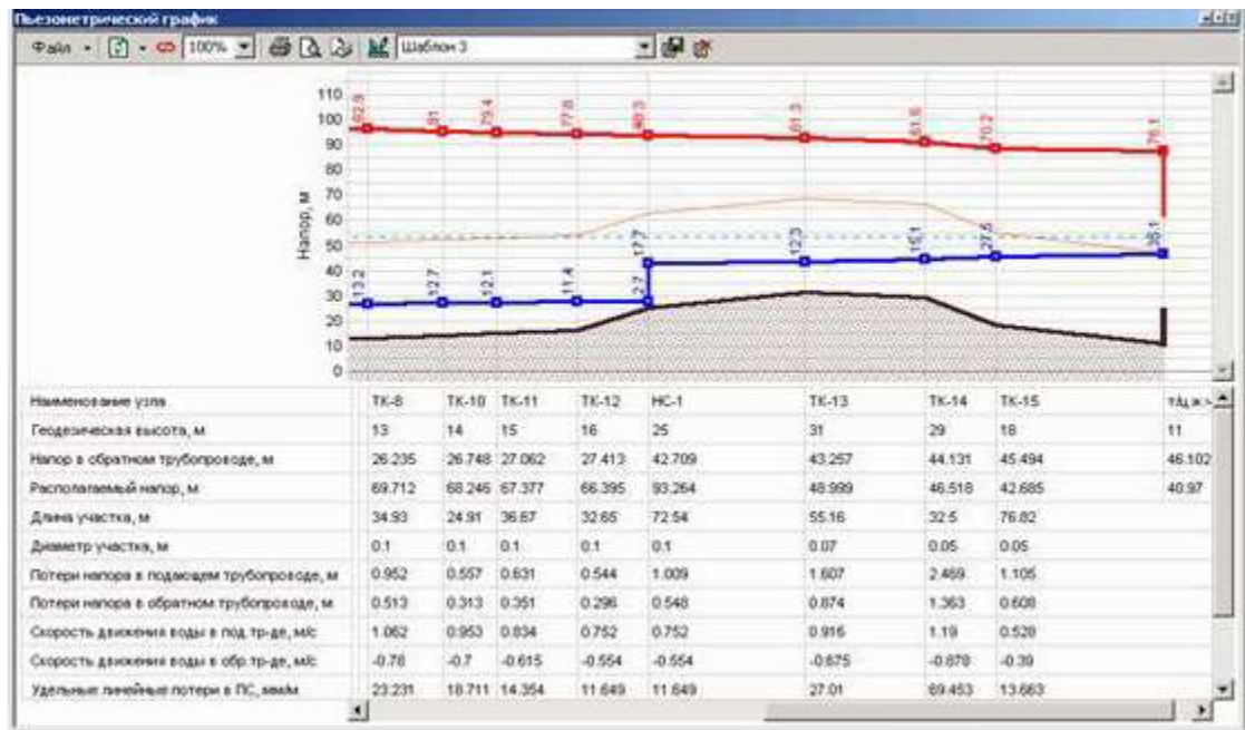
Рисунок 23 – Пьезометрический график
